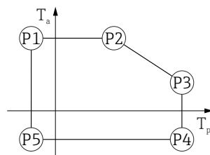
16 Boîtier plastique ; température de process -40 \dots +130 \text{ °C} ( -40 \dots +266 \text{ °F} )
