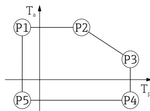
32 Boîtier 316L ; gamme de température de process : -40 \dots +150 \text{ }^{\circ}\text{C} ( -40 \dots +302 \text{ }^{\circ}\text{F} )
