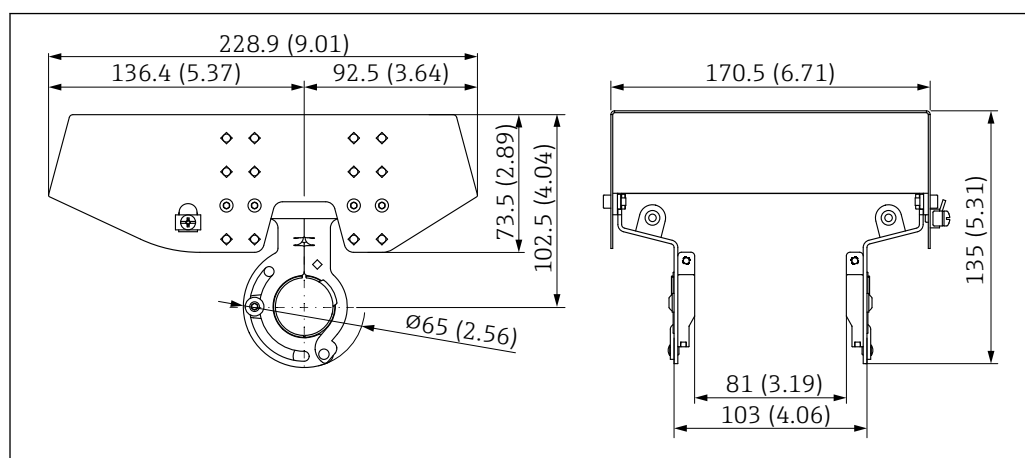
64 Dimensions du capot de protection climatique, 316 L, XW112. Unité de mesure mm (in)
