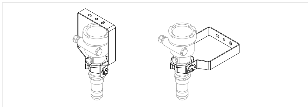
66 Étrier de montage réglable FMR6xB ; montage sur toit ou sur paroi
