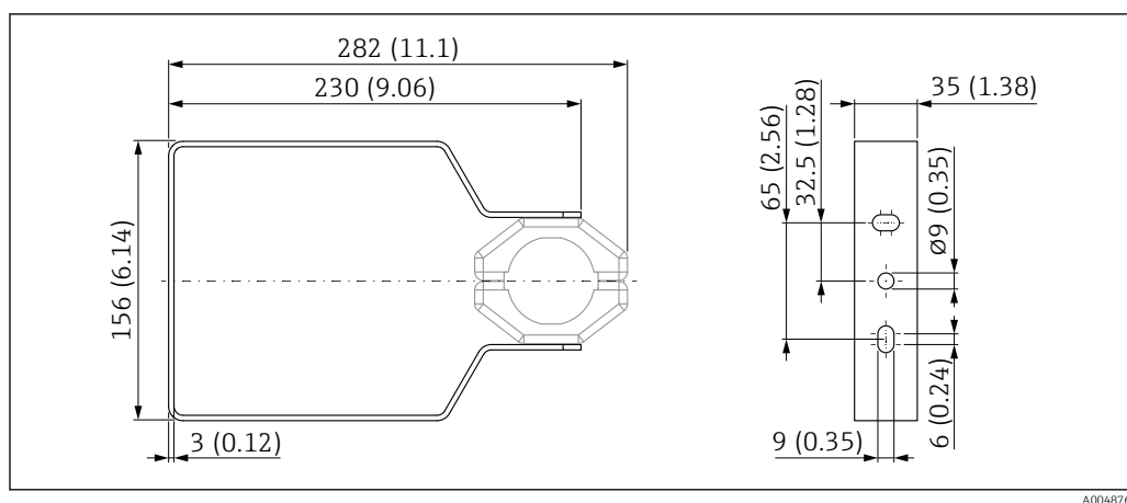
67 Dimensions ; étrier de montage réglable FMR6xB. Unité de mesure mm (in)
