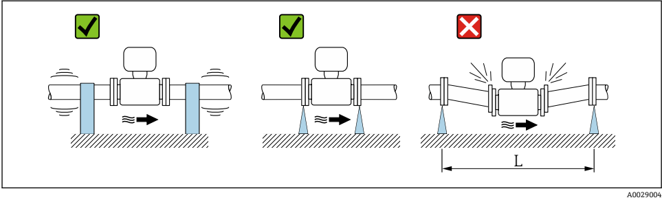
6 避免仪表振动的措施( L > 10\text{ m} (33 ft))
