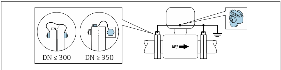
2 Potenzialausgleich über Erdungsklemme und Rohrleitungsflansche
