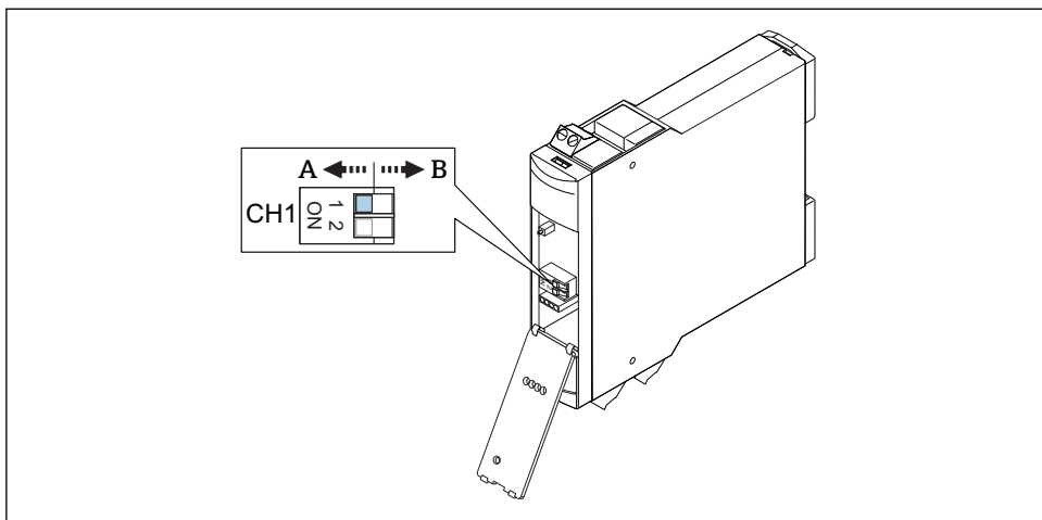
図 12 スイッチングユニットのスイッチ位置
