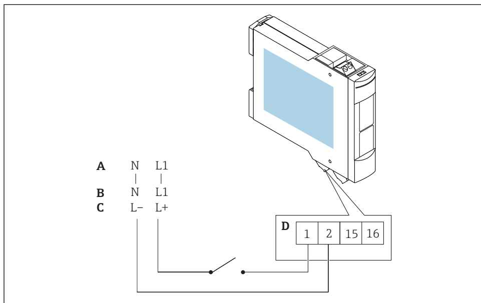
図 6 端子の配置
