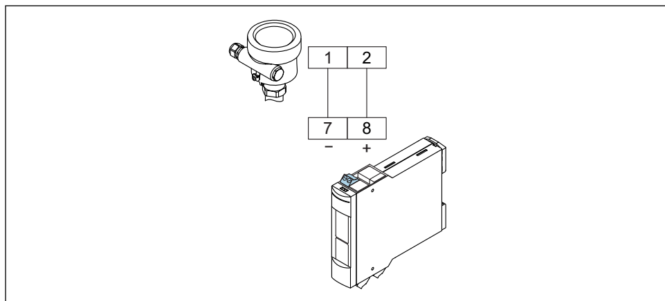
図 7 センサと NAMUR センサとの接続
