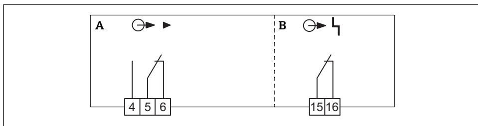
8 Conectarea ieșirilor
