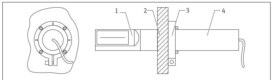
5 Installatie van de staafsensor met een montageflens
