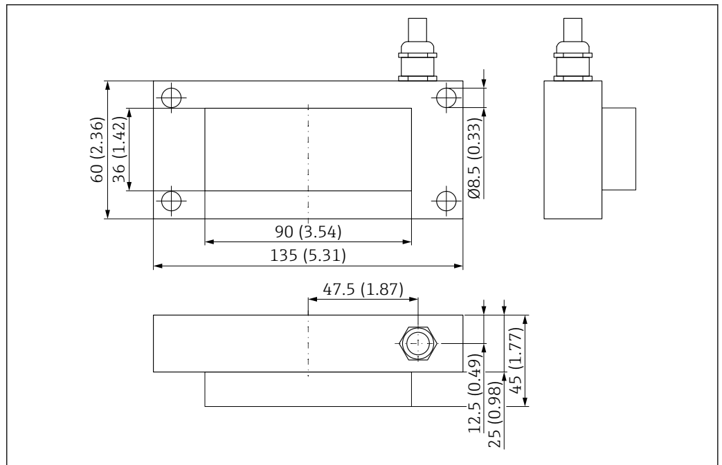
4 Afmetingen van rechthoekige sensor. Maateenheid mm (in)
