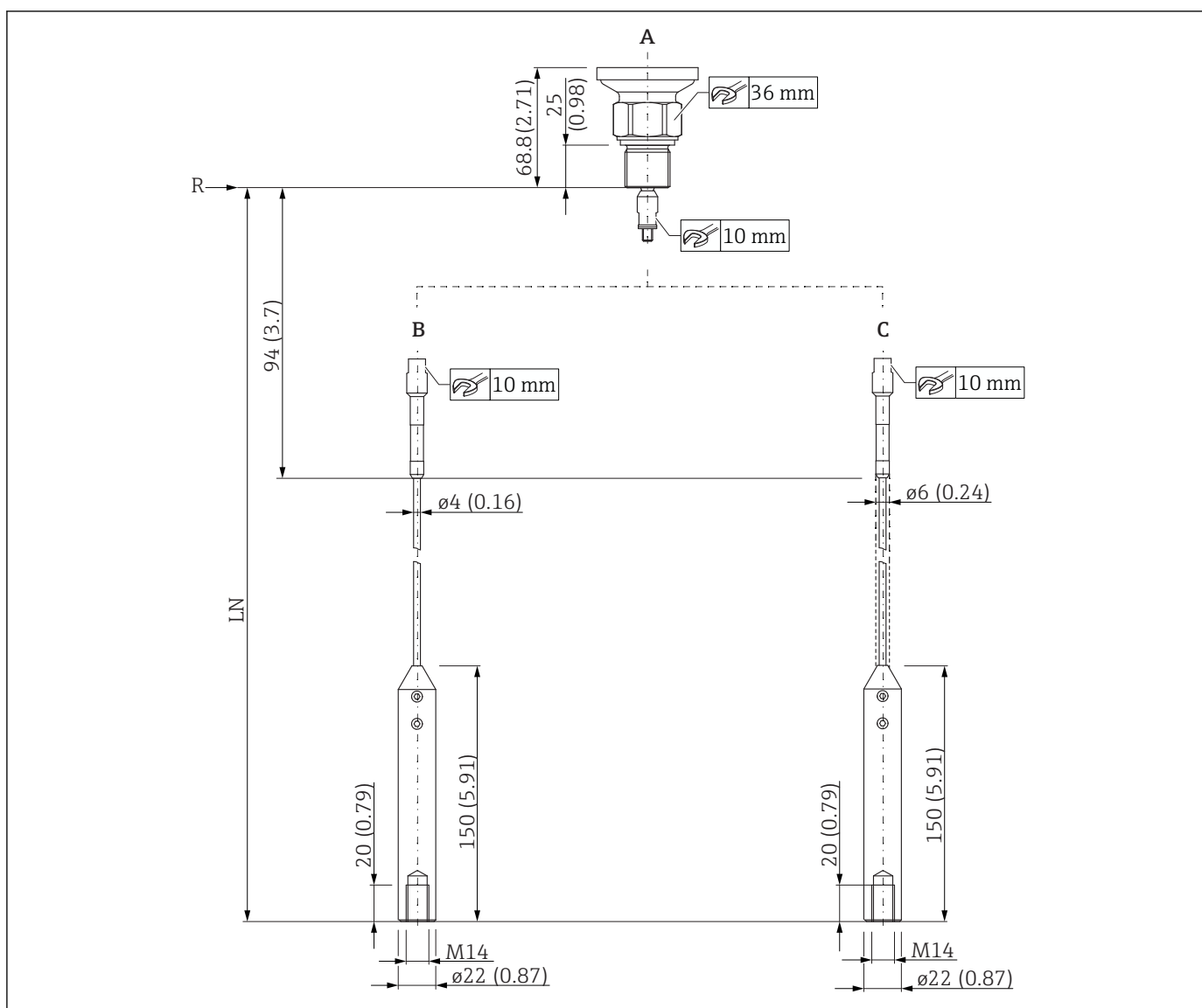
33 FMP56: Przyłącze procesowe / falowód. Jednostka miary mm (in)
