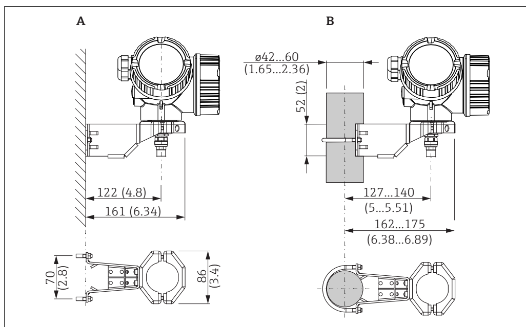
31 Wspornik montażowy obudowy modułu elektronicznego. Jednostka miary mm (in)
