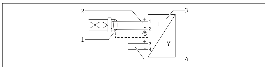
14 Schemat blokowy wersji PROFIBUS PA / FOUNDATION Fieldbus
