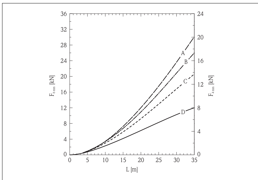
23 Pszenica w zbiorniku o gładkich ścianach metalowych; obciążenie rozciągające w funkcji poziomu L dla liny 6 mm (0,24") i 4 mm (0,16")
