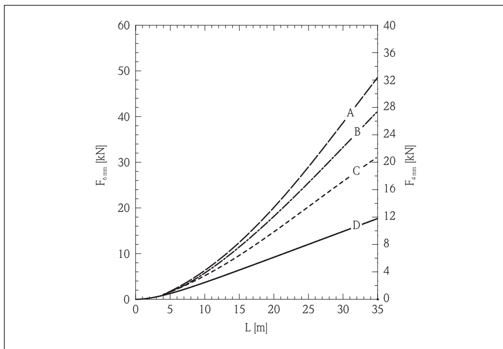
21 Piasek kwarcowy w zbiorniku o gładkich ścianach metalowych; obciążenie rozciągające w funkcji poziomu L dla liny 6 mm (0,24") i 4 mm (0,16")
