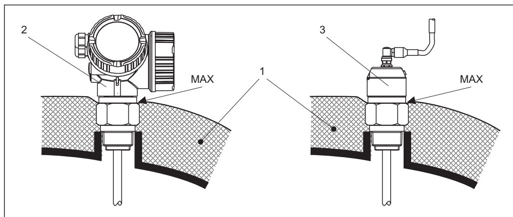
26 Przyłącze procesowe z gwintem - FMP56, FMP57
