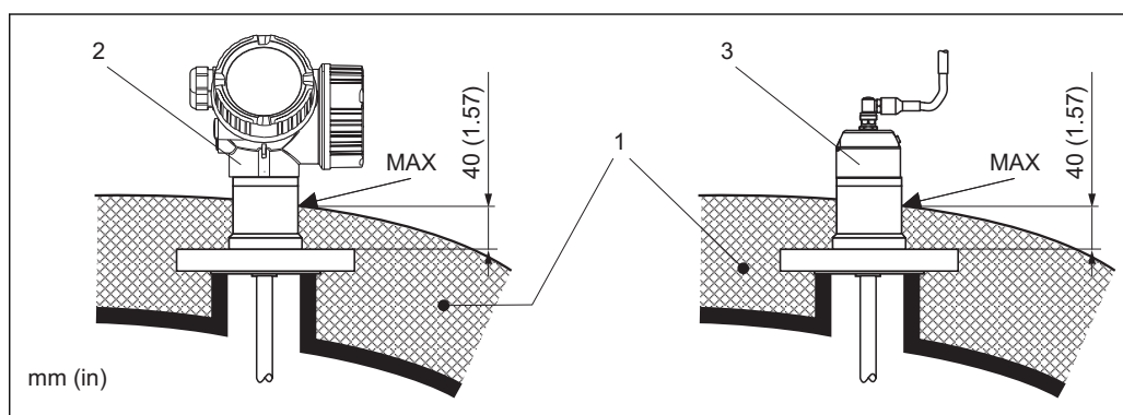
27 Przyłącze procesowe z kołnierzem - FMP57
