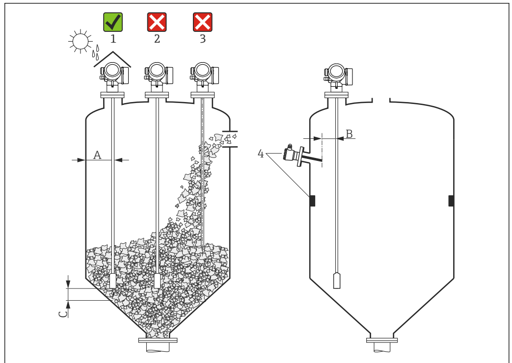
20 Wymagania montażowe dla Levelflex
