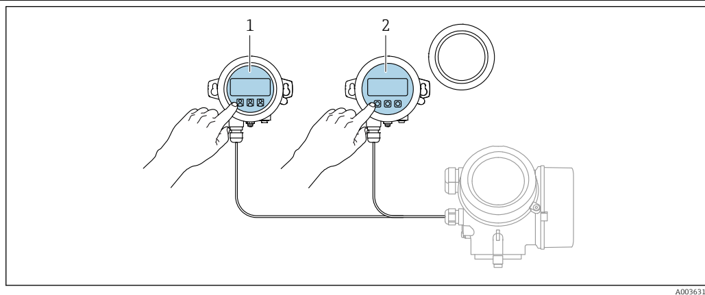
35 Warianty obsługi za pomocą zewnętrznego wskaźnika FHX50
