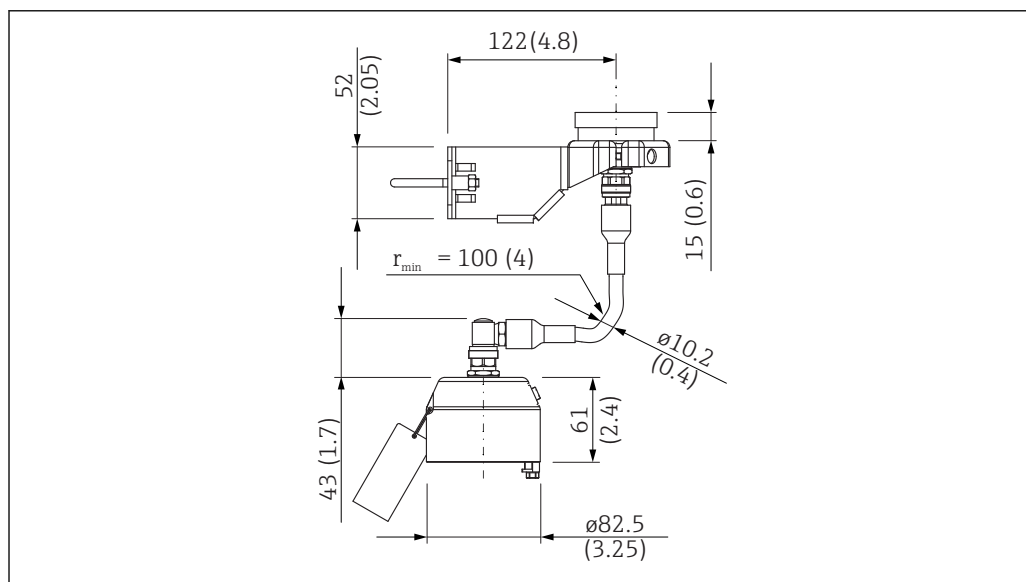
32 Wspornik montażowy dla wersji rozdzielnej sondy; Długość przewodu podłączeniowego zgodna z zamówieniem. Jednostka miary mm (in)
