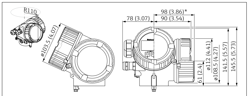
30 Obudowa GT20 (aluminiowa malowana proszkowo); Wymiary w mm (calach)
