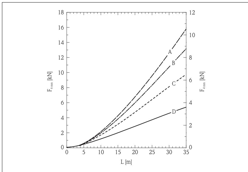
22 Granulat polietyleny w zbiorniku o gładkich ścianach metalowych; obciążenie rozciągające w funkcji poziomu L dla liny 6 mm (0,24") i 4 mm (0,16")
