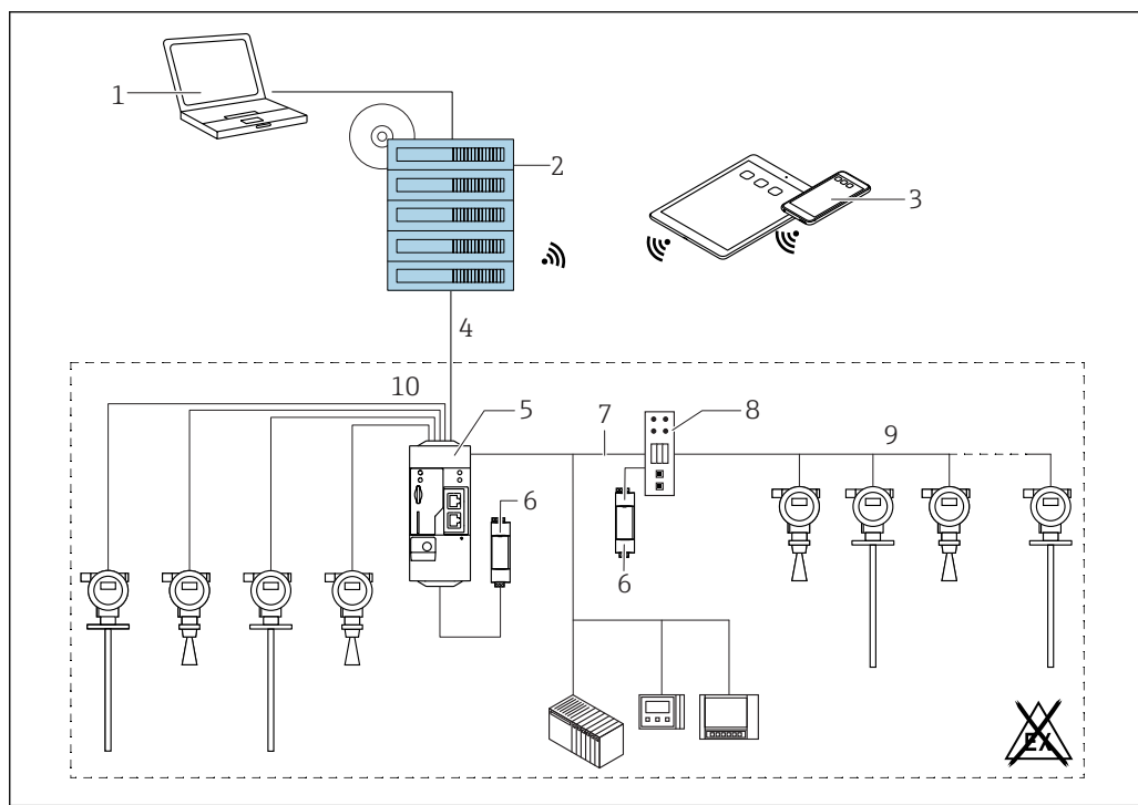
42 Przykład platformy do zarządzania stanami magazynowym w wersji SupplyCare Enterprise SCE30B
