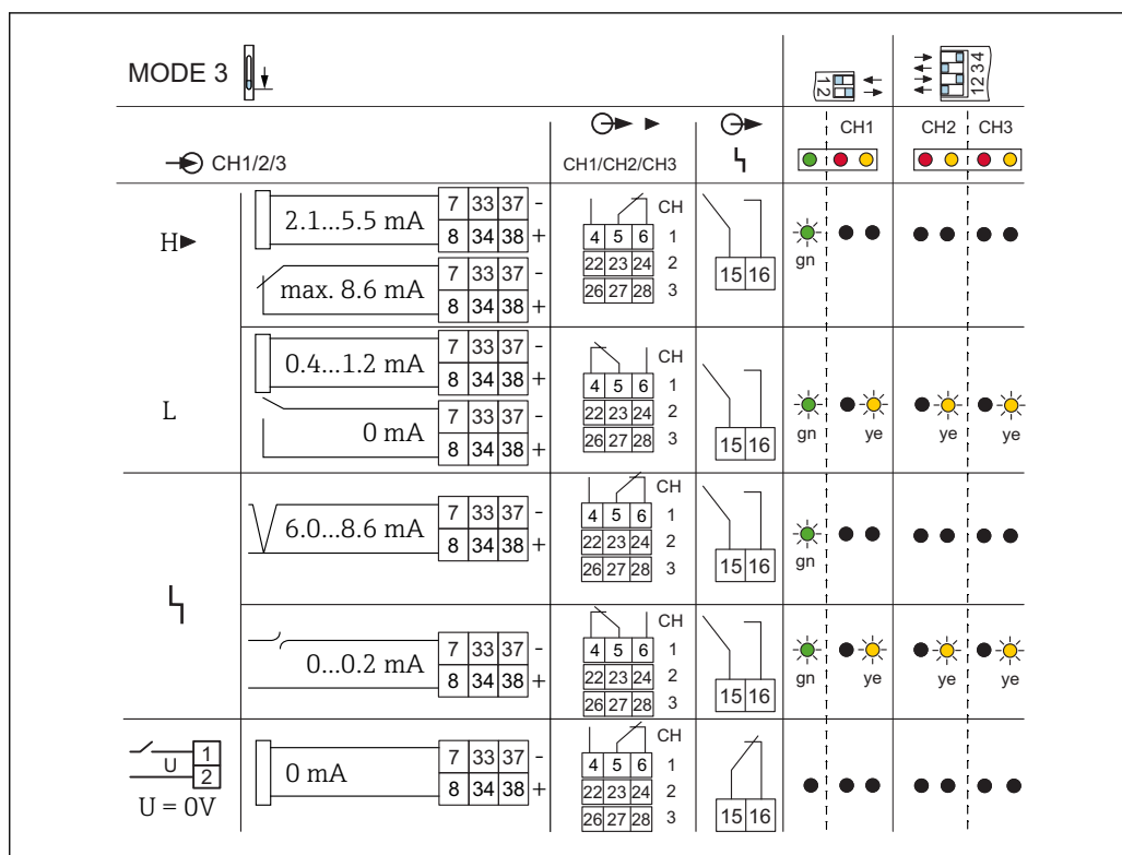
26 スイッチング動作およびエラー電流 H > 2.1 \text{ mA} (FEL56) の場合の信号伝達
