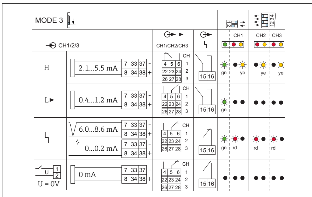
図 27 スイッチング動作およびエラー電流 L < 1.2 \text{ mA} (FEL48、FEL58、FEL68、FEM58、FEI58) の場合の信号伝達
