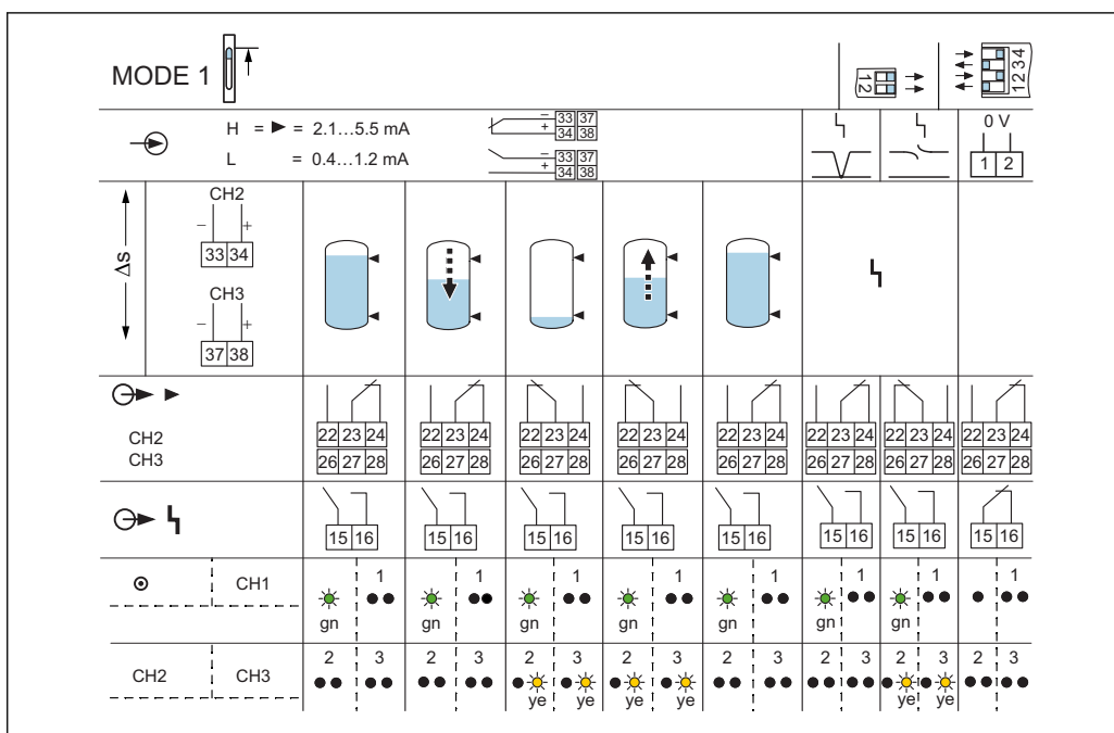
30 スイッチング動作およびエラー電流 H > 2.1 \text{ mA} (FEL56) の場合の信号伝達
