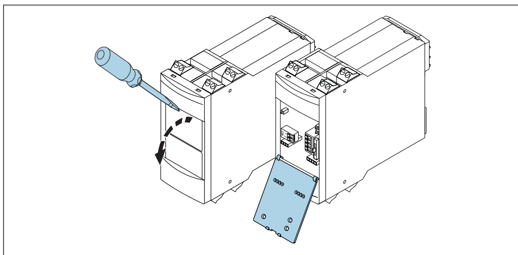
■ 11 フロントパネルの開放
