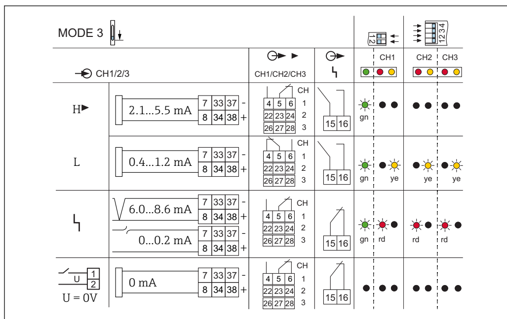
図 25 スイッチング動作およびエラー電流 H > 2.1 \text{ mA} (FEL56) の場合の信号伝達
