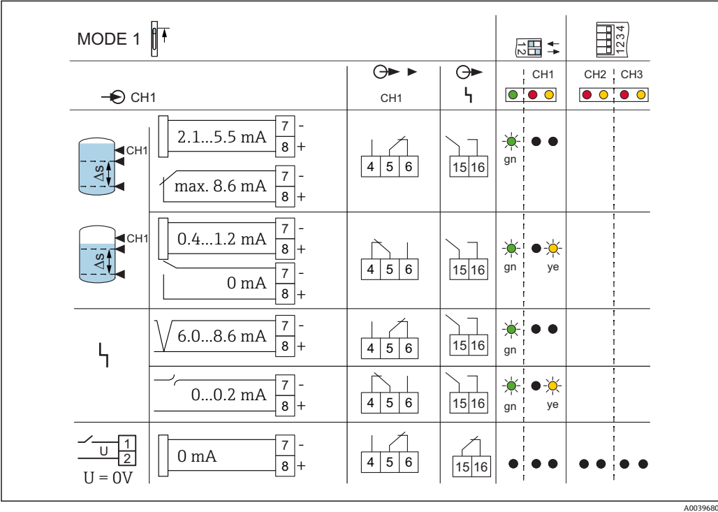
図 34 スイッチング動作およびエラー電流 H > 2.1 mA (FEL56) の場合の信号伝達
