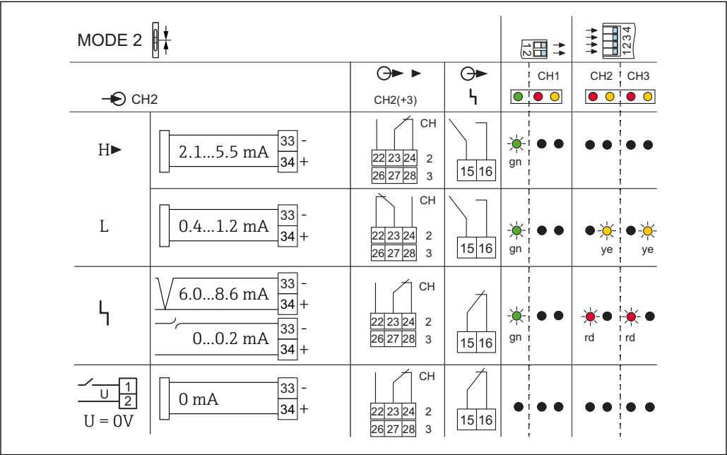
図 17 スイッチング動作およびエラー電流 H > 2.1 mA (FEL56) の場合の信号伝達
