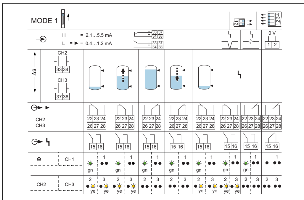
■ 32 スイッチング動作およびエラー電流 L < 1.2 \text{ mA} (FEL48、FEL58、FEL68、FEM58、FEI58) の場合の信号伝達
