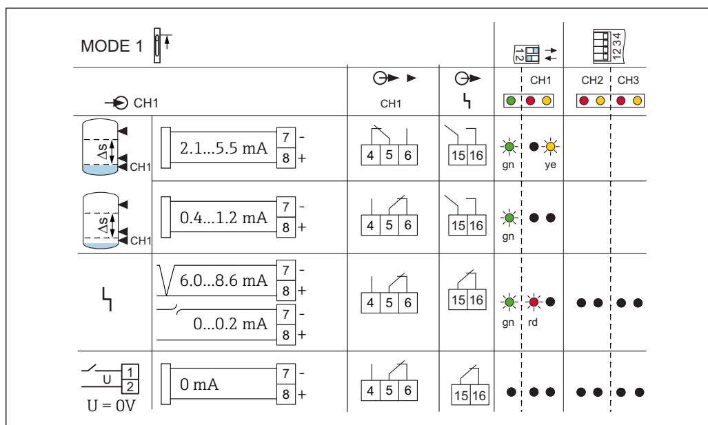
図 35 スイッチング動作およびエラー電流 L < 1.2 \text{ mA} (FEL48、FEL58、FEL68、FEM58、FEI58) の場合の信号伝達
