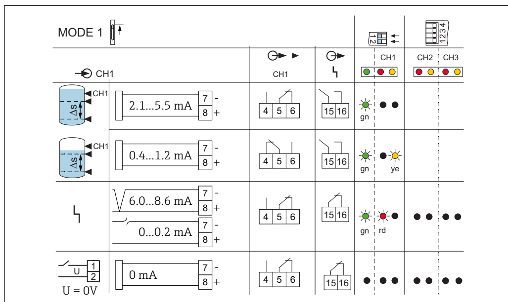
33 スイッチング動作およびエラー電流 H > 2.1 \text{ mA} (FEL56) の場合の信号伝達
