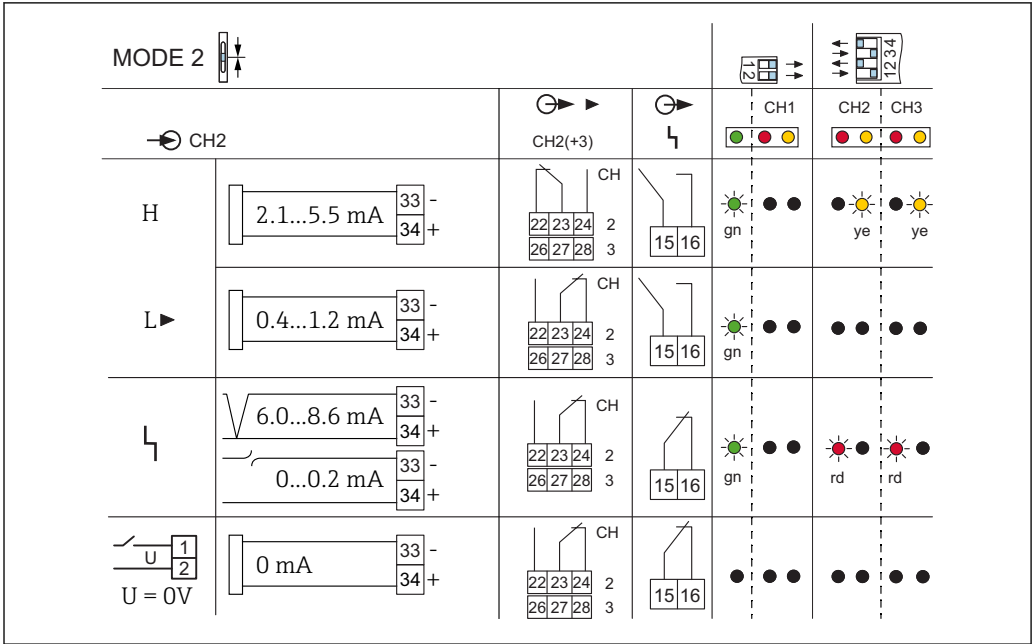
図 19 スイッチング動作およびエラー電流 L < 1.2 \text{ mA} (FEL48、FEL58、FEL68、FEM58、FEI58) の場合の信号伝達
