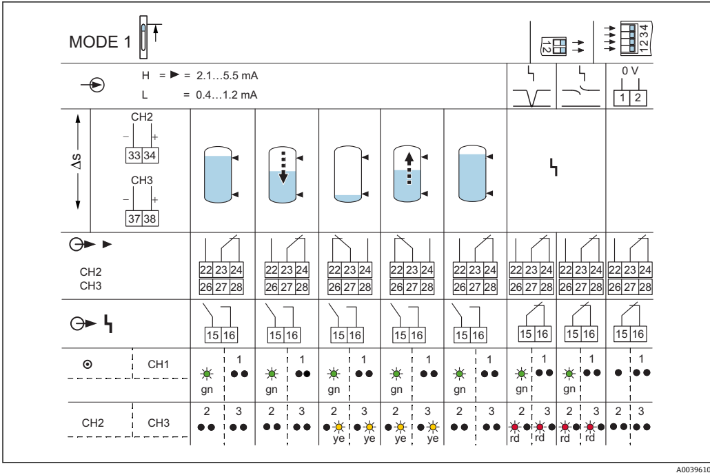
図 29 スイッチング動作およびエラー電流 H > 2.1 mA (FEL56) の場合の信号伝達
