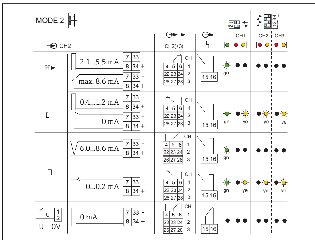
図 22 スイッチング動作およびエラー電流 H > 2.1 \text{ mA} (FEL56) の場合の信号伝達
