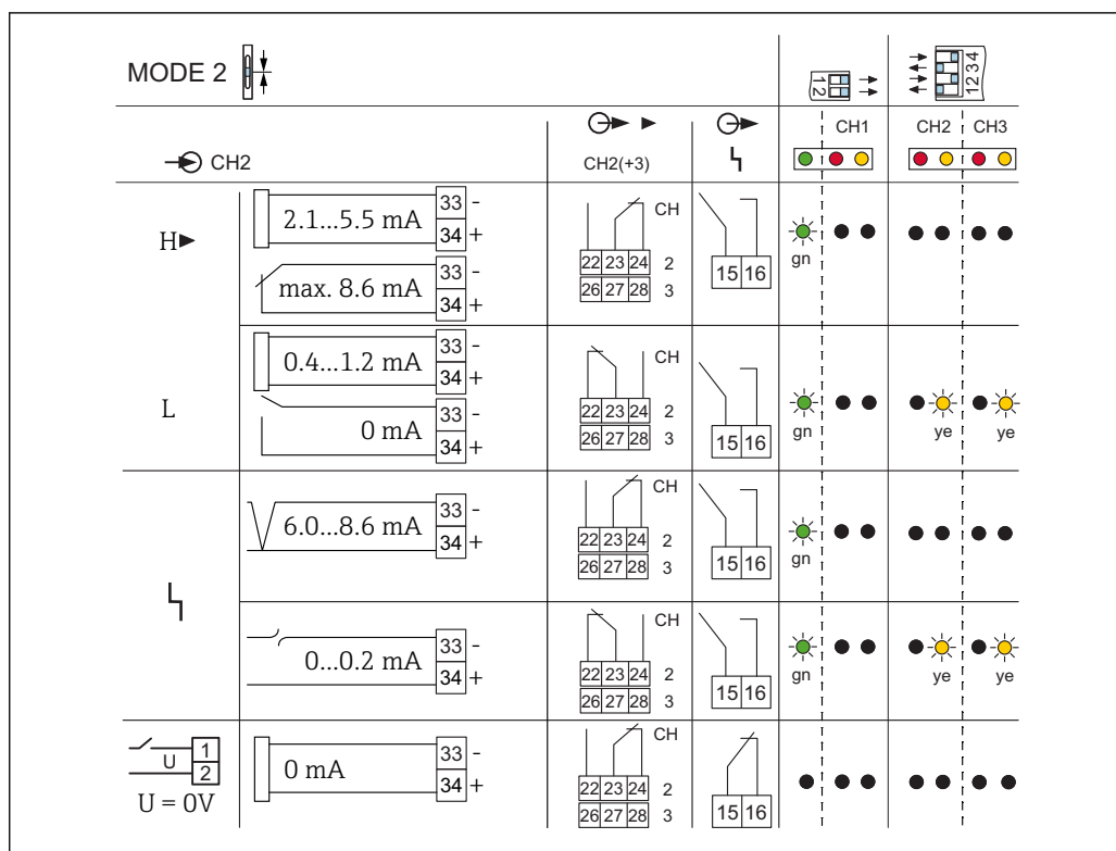
図 18 スイッチング動作およびエラー電流 H > 2.1 \text{ mA} (FEL56) の場合の信号伝達
