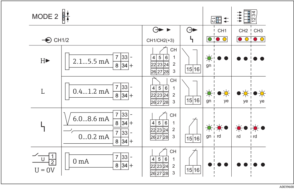
図 21 スイッチング動作およびエラー電流 H > 2.1 \text{ mA} (FEL56) の場合の信号伝達
