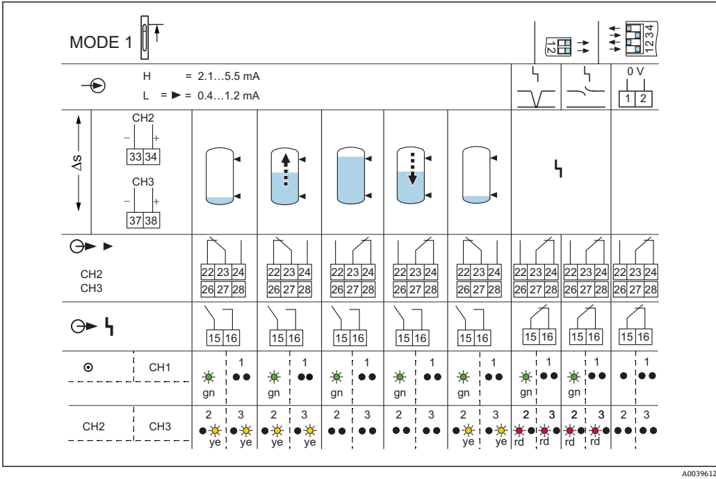
図 31 スイッチング動作およびエラー電流 L < 1.2 \text{ mA} (FEL48、FEL58、FEL68、FEM58、FEI58) の場合の信号伝達
