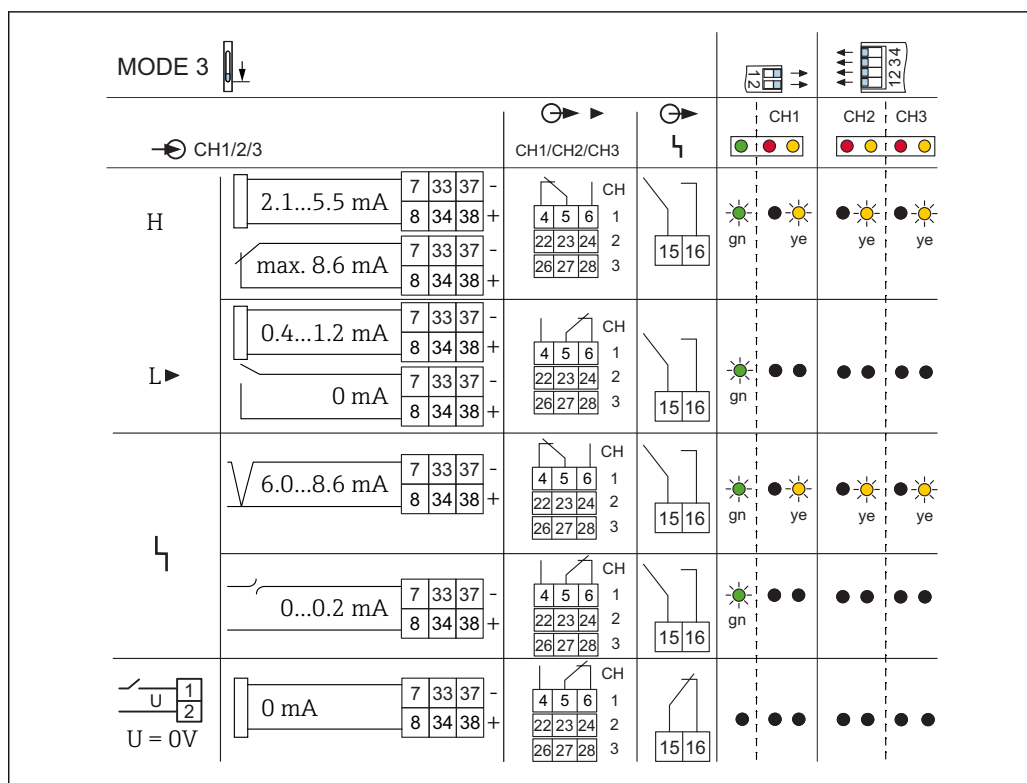
■ 28 スイッチング動作およびエラー電流 L < 1.2 \text{ mA} (FEL48、FEL58、FEL68、FEM58、FEI58) の場合の信号伝達
