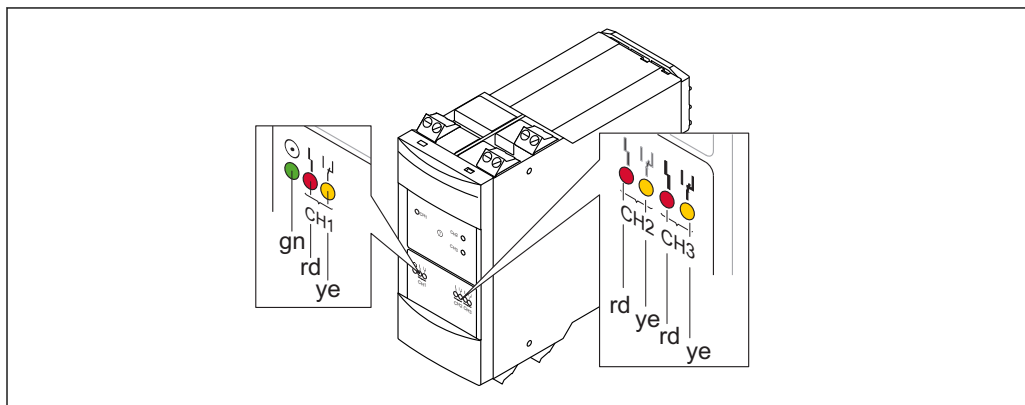
■ 12 Nivotester、発光ダイオード (LED)
