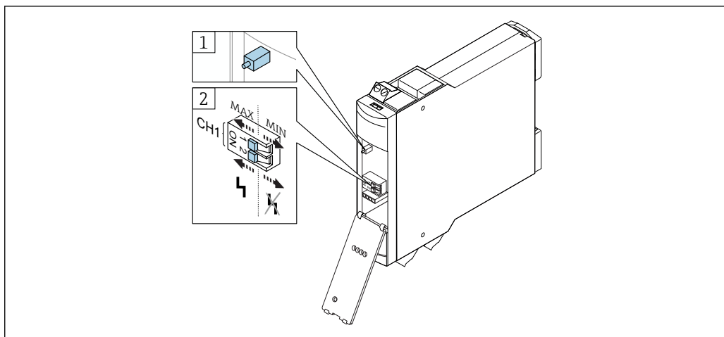
図 12 操作部
