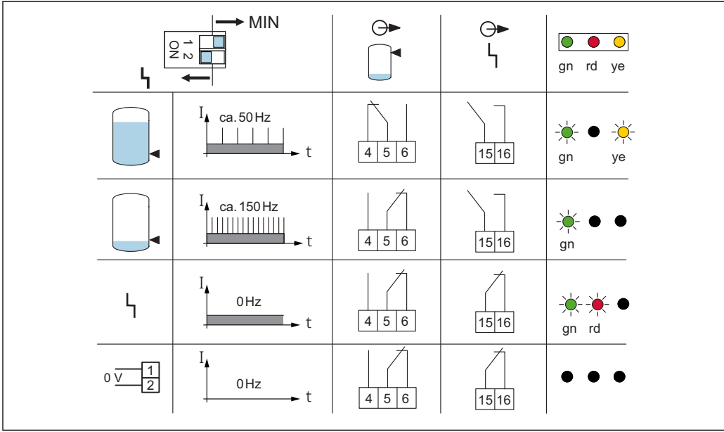
図 18 スイッチング動作および信号伝達
