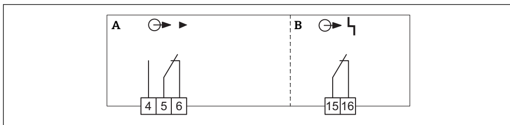
図 9 出力の接続
