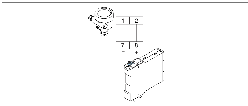
図 8 センサと Nivotester の接続
