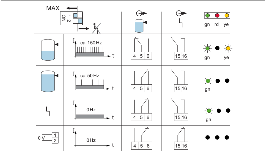
図 17 スイッチング動作および信号伝達
