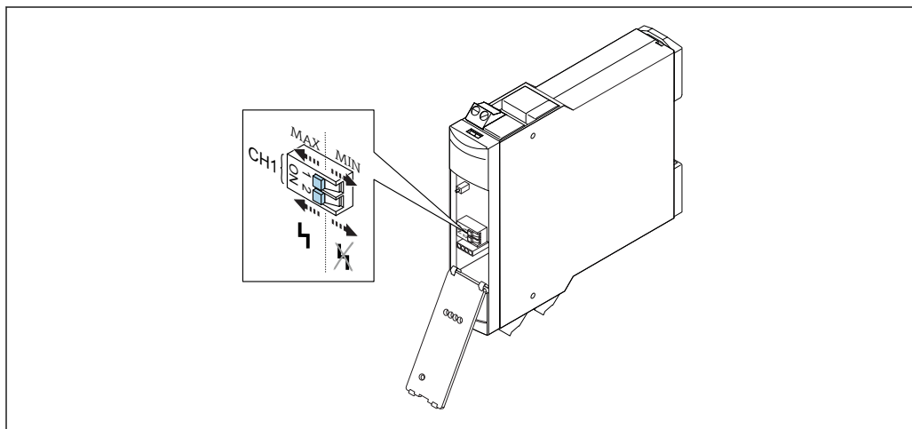
図 13 機能設定用のスイッチ
