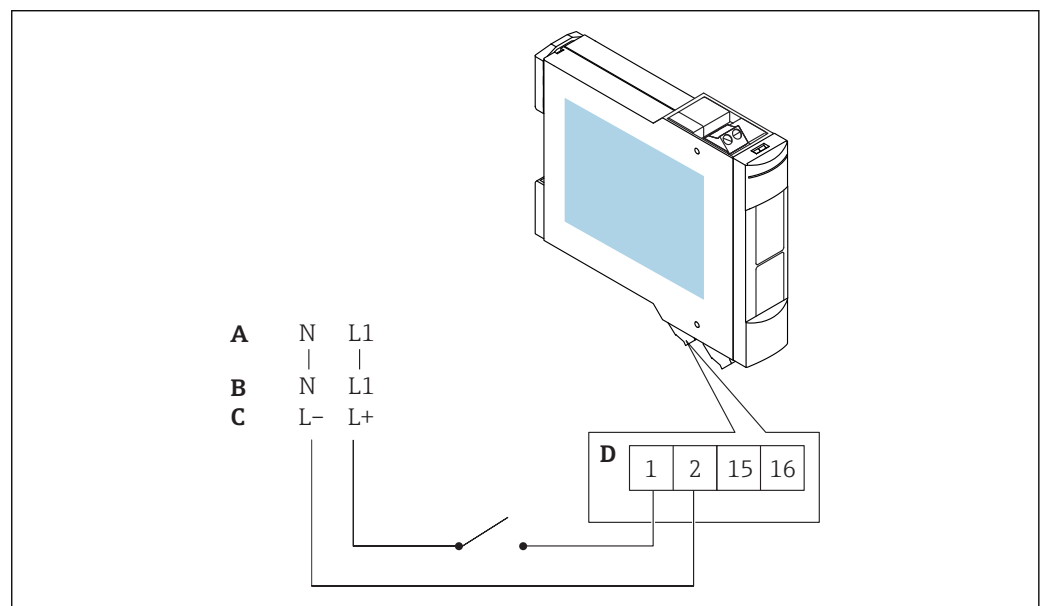
図 7 端子の配置
