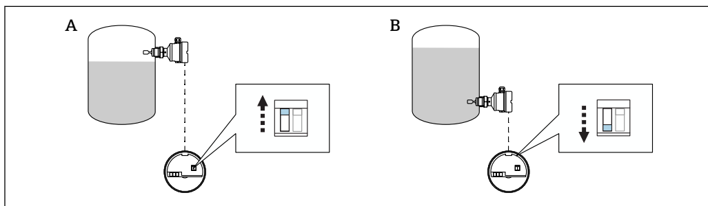
図 14 エレクトロニックインサート (FEL67) のスイッチ位置
