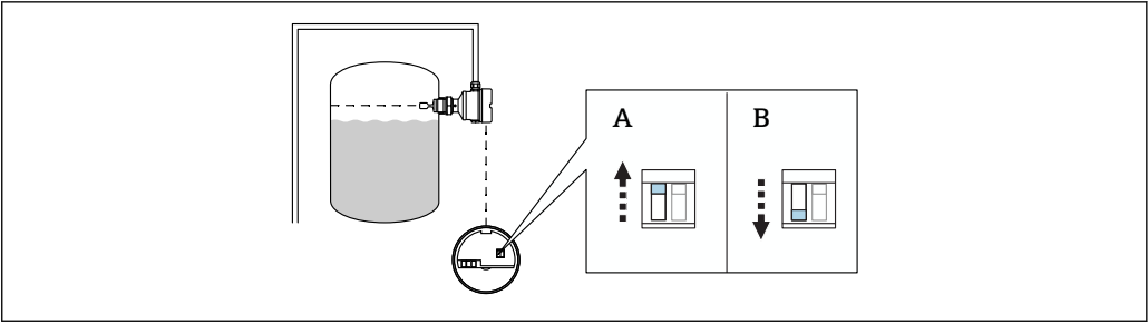
15 エレクトロニックインサート (FEL57) のスイッチ位置
