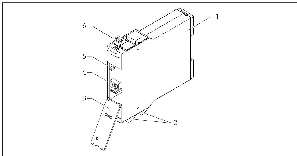
図 1 製品構成
