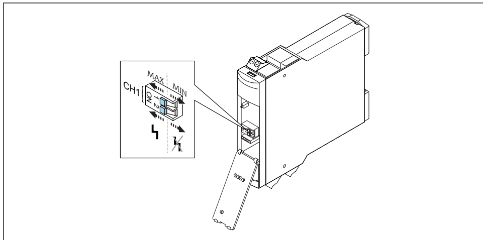
図 12 機能設定用のスイッチ
