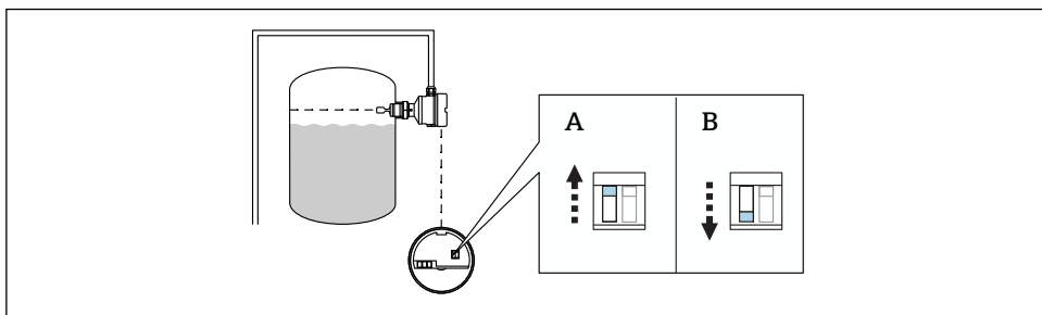
図 14 エレクトロニックインサート (FEL57) のスイッチ位置
