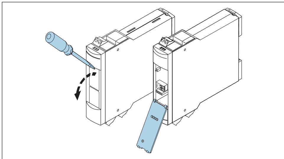
図 9 フロントパネルの開放
