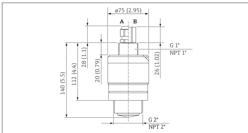
図 24 G 2" または MNPT 2" プロセス接続ネジの寸法、単位 : mm (in)
