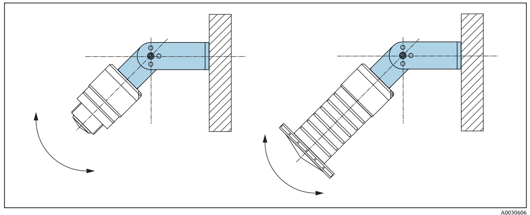
図 18 調整可能な取付ブラケットによる設置
