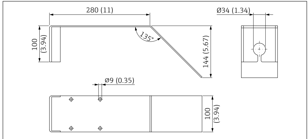
■ 58 下水シャフト用水平取付ブラケットの寸法。測定単位 mm (in)
