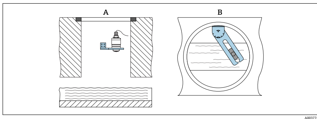
図 21 シャフトに取付け、回転および調整可能
