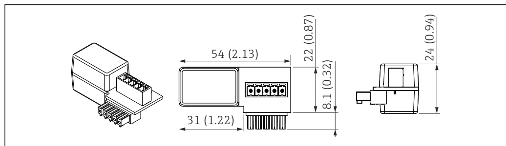
図 60 HART 通信抵抗器の寸法、単位：mm (in)
