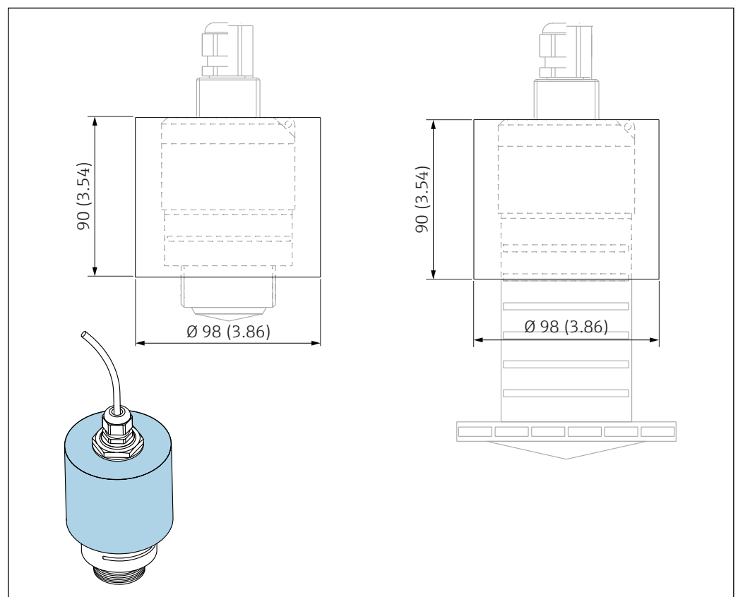
図 35 日除けカバーの寸法、単位：mm (in)
