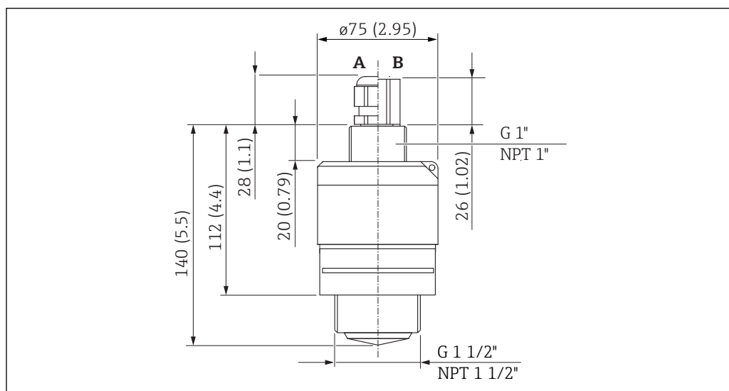
図 23 G 1-½" または MNPT 1-½" プロセス接続ネジの寸法、単位 : mm (in)
