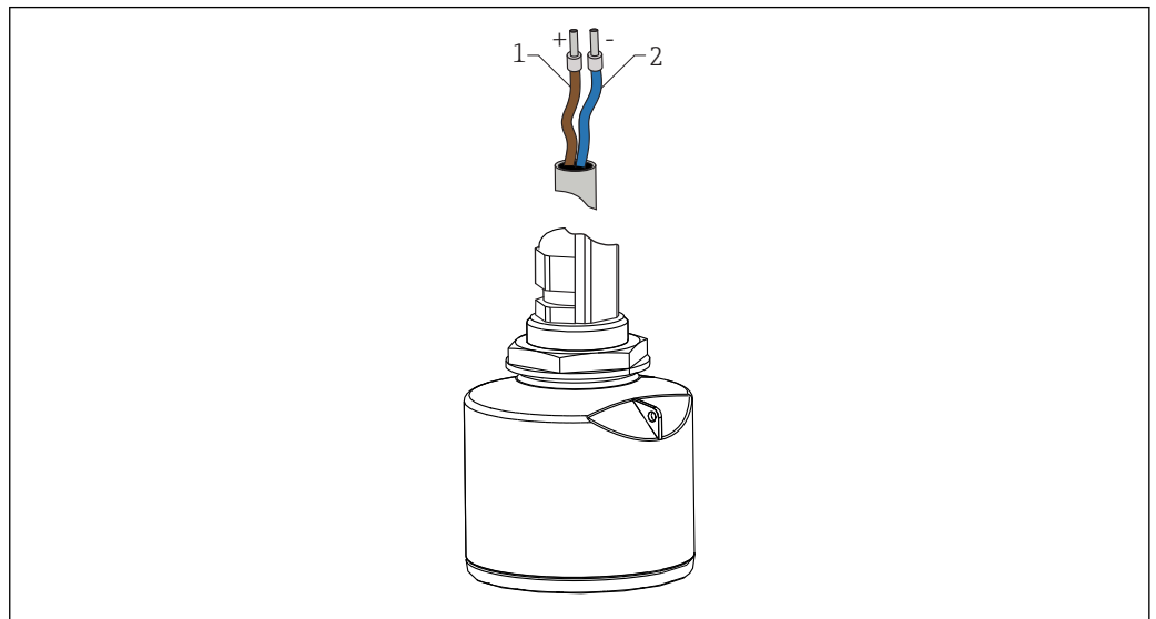
図 2 ケーブルの割当て
