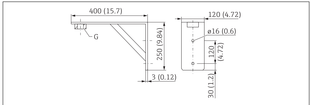
図 44 アングルブラケットの寸法。測定単位 mm (in)
