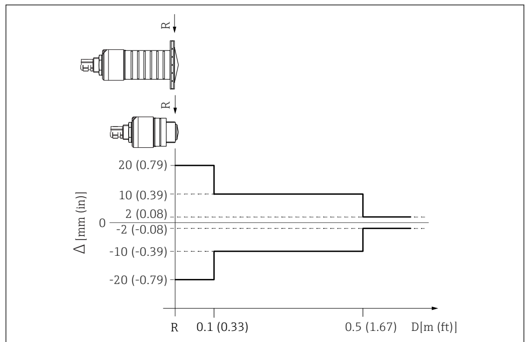
図 9 近範囲アプリケーションにおける最大測定誤差、標準バージョンの値
