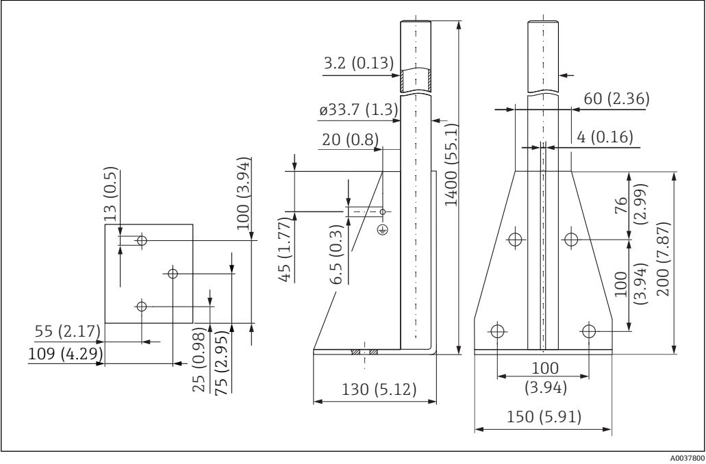
図 54 取付フレーム（ロング）の寸法。測定単位 mm (in)
