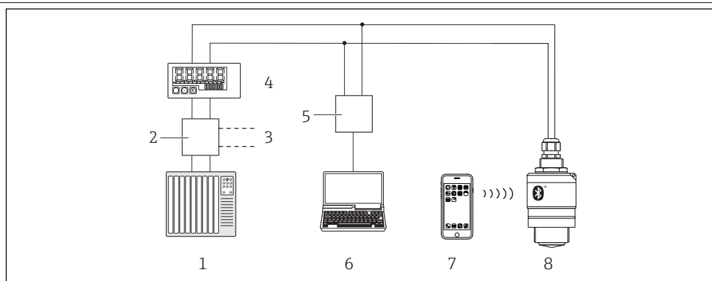
図 34 HART 経由のリモート操作オプション
