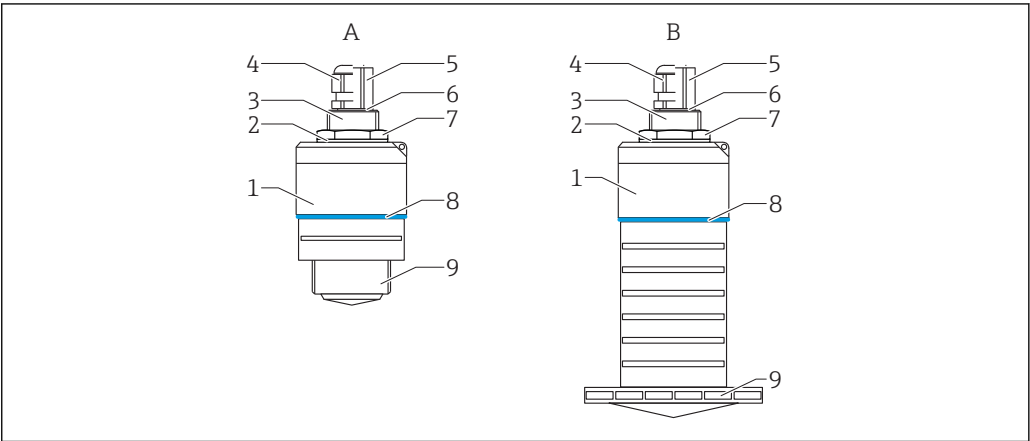
図 32 材質の概要
