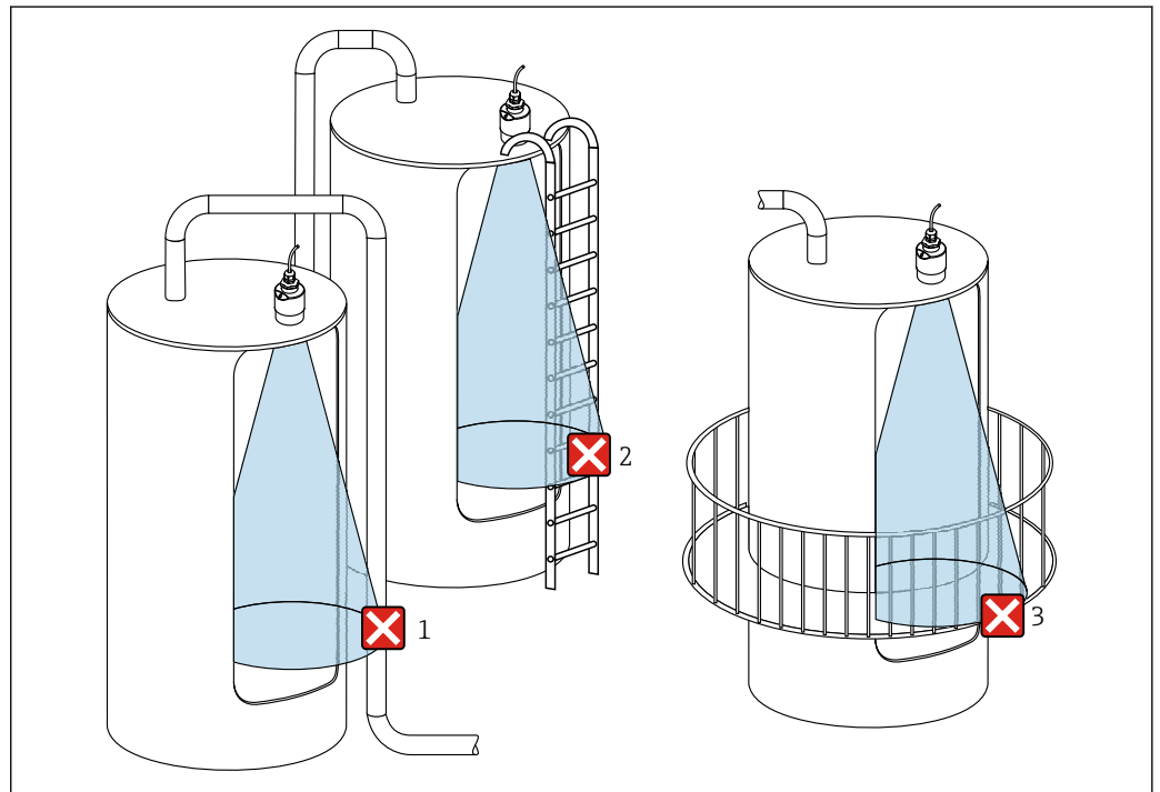
図 15 金属製の干渉物がタンク外側にあるプラスチックタンク内の測定
