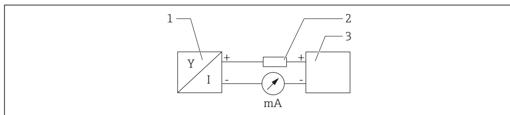
図 4 HART 接続のブロック図
