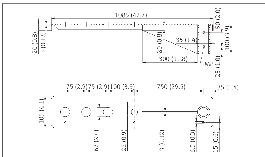
図 52 回転可能なセンササポート（ロング）、前面センサプロセス接続 G 2" の寸法。測定単位 mm (in)
