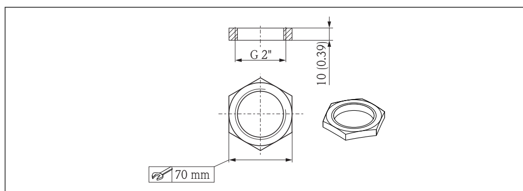
図 37 固定ナットの寸法、単位：mm (in)
