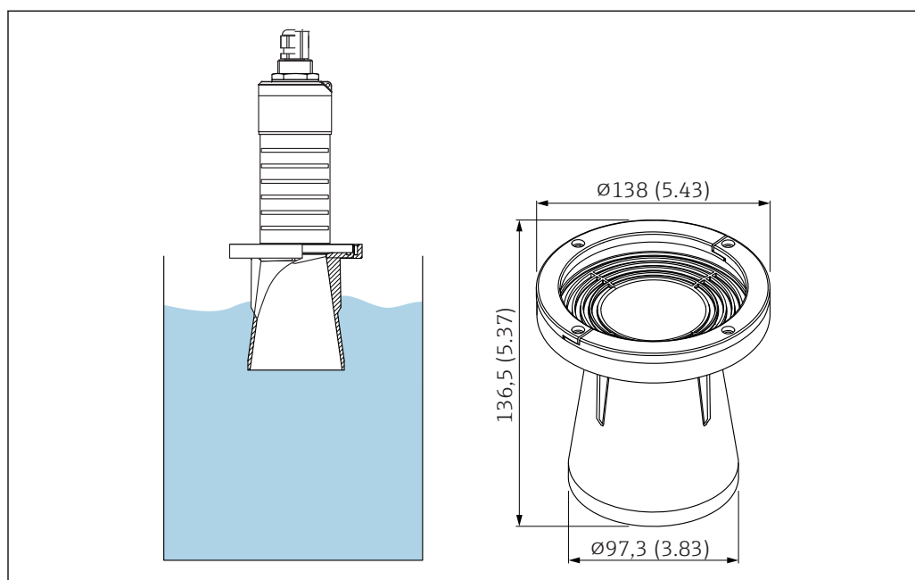
図 39 溢れ防止チューブ 80 mm (3 in) の寸法、単位：mm (in)
