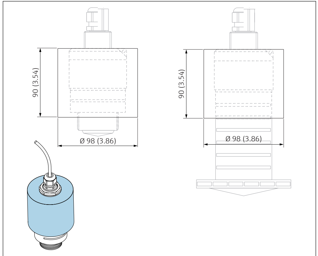
35 日除けカバーの寸法、単位：mm (in)
