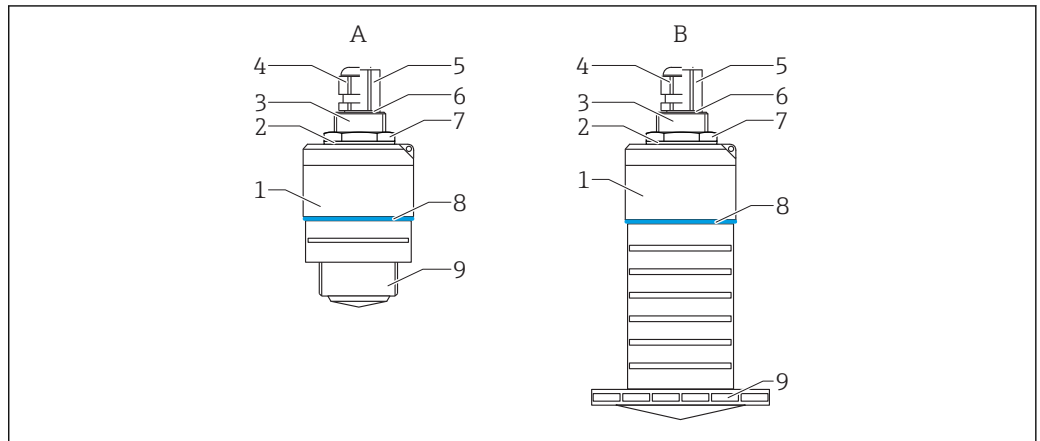
図 32 材質の概要
