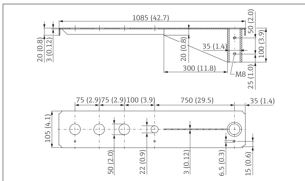
図 50 回転可能なセンササポート（ロング）、前面センサプロセス接続 G 1-½" の寸法。測定単位 mm (in)
