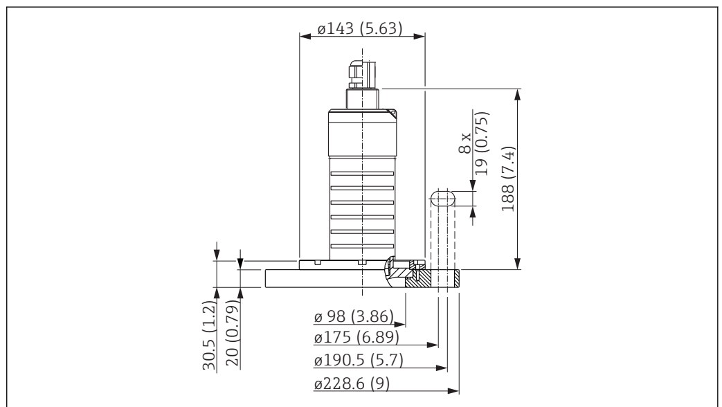
■ 29 スリップオンフランジ 4"/DN100 付き 80 mm (3 in) アンテナの寸法、単位：mm (in)
