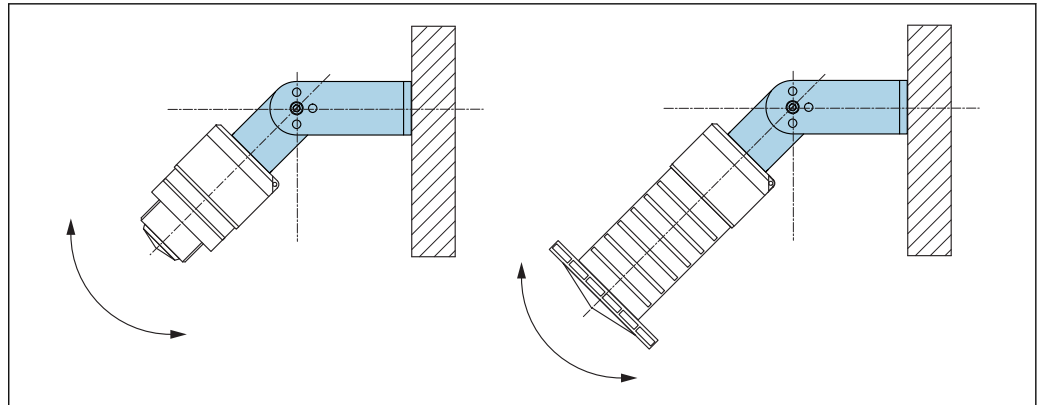
図 18 調整可能な取付ブラケットによる設置
