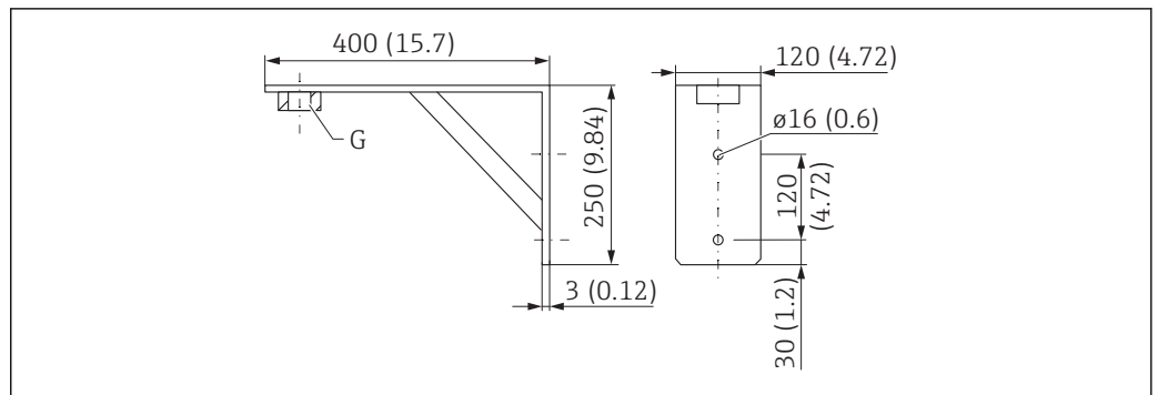
図 44 アングルブラケットの寸法。測定単位 mm (in)
