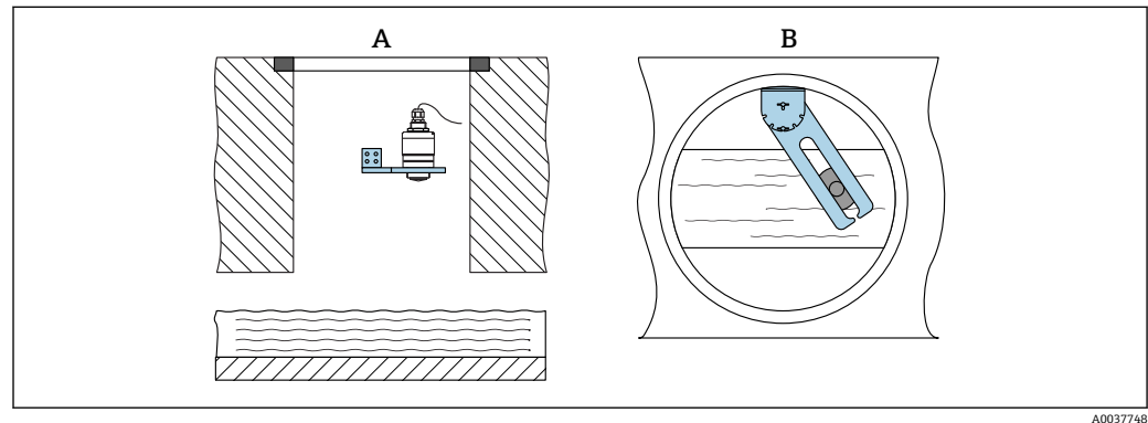
図 21 シャフトに取付け、回転および調整可能
