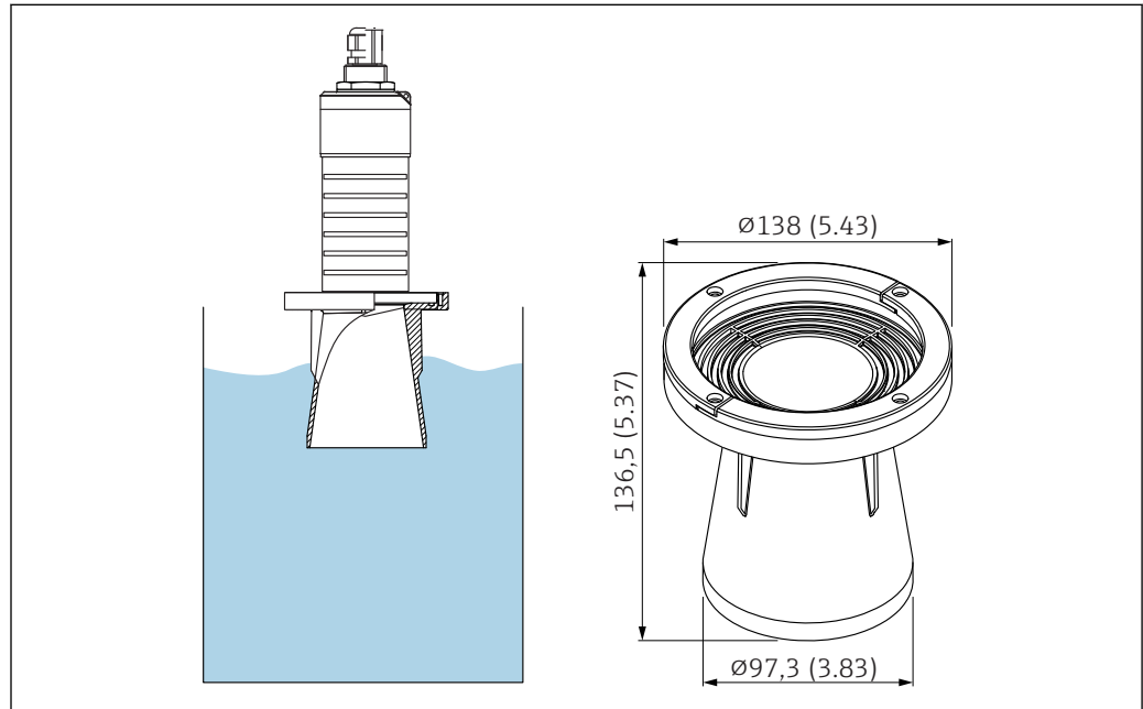
図 39 溢れ防止チューブ 80 mm (3 in) の寸法、単位：mm (in)
