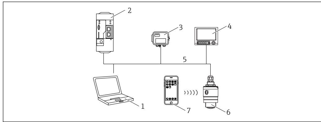
図 34 Modbus プロトコルを介したリモート操作用オプション
