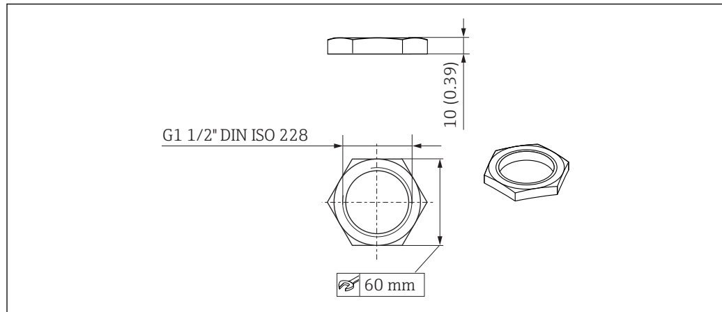
図 36 固定ナットの寸法、単位：mm (in)
