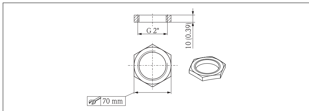
図 37 固定ナットの寸法、単位：mm (in)
