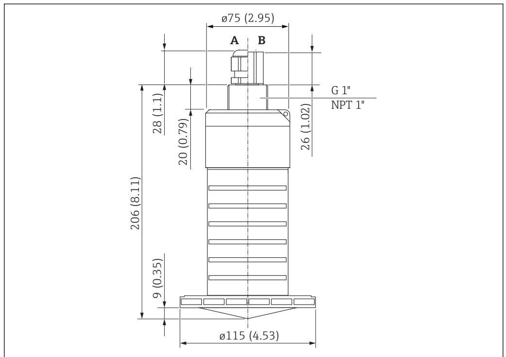
■ 26 80 mm (3 in) アンテナの寸法、単位：mm (in)
