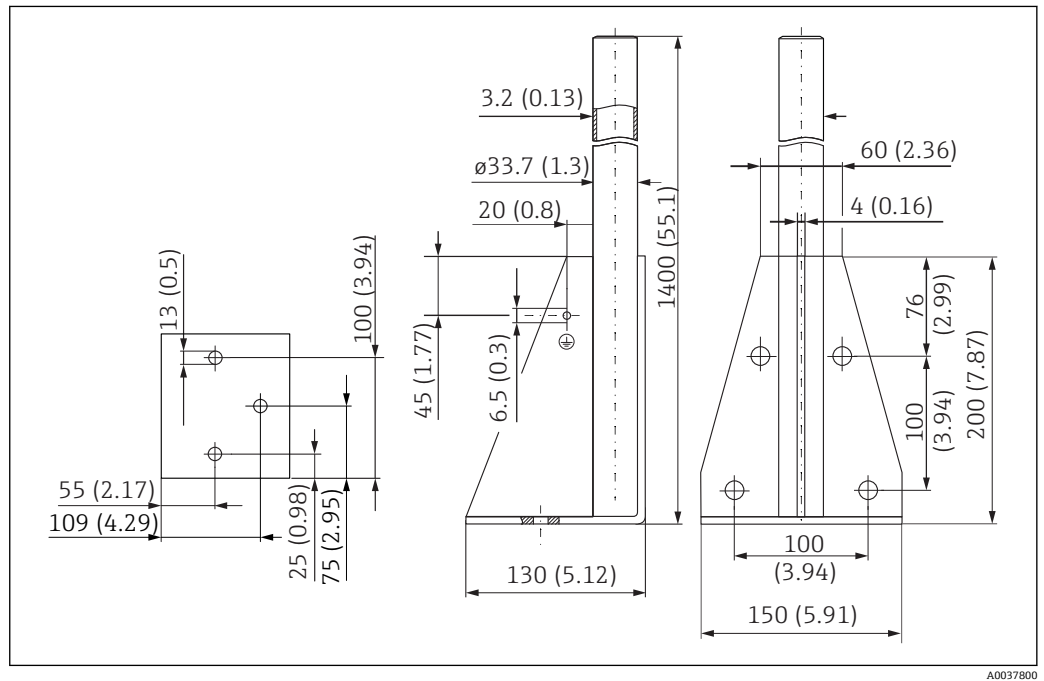
図 54 取付フレーム（ロング）の寸法。測定単位 mm (in)
