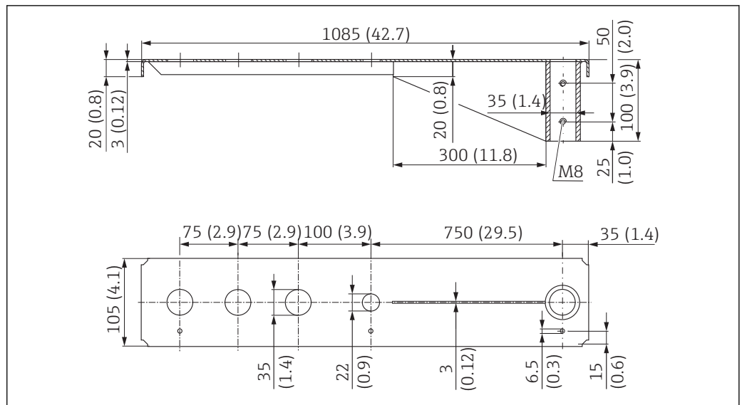
図 47 回転可能なセンササポート（ロング）、背面センサプロセス接続の寸法。測定単位 mm (in)
