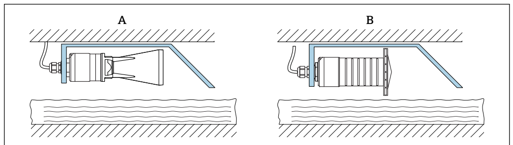
図 20 下水シャフト用水平取付ブラケットの取付け
