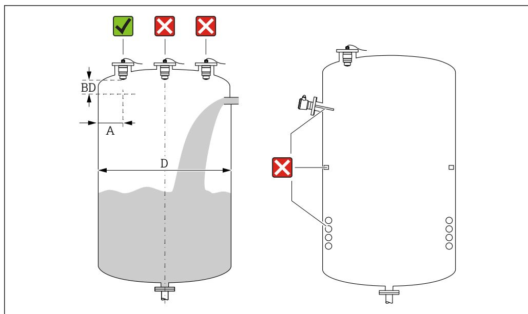
図 11 容器内の設置位置
