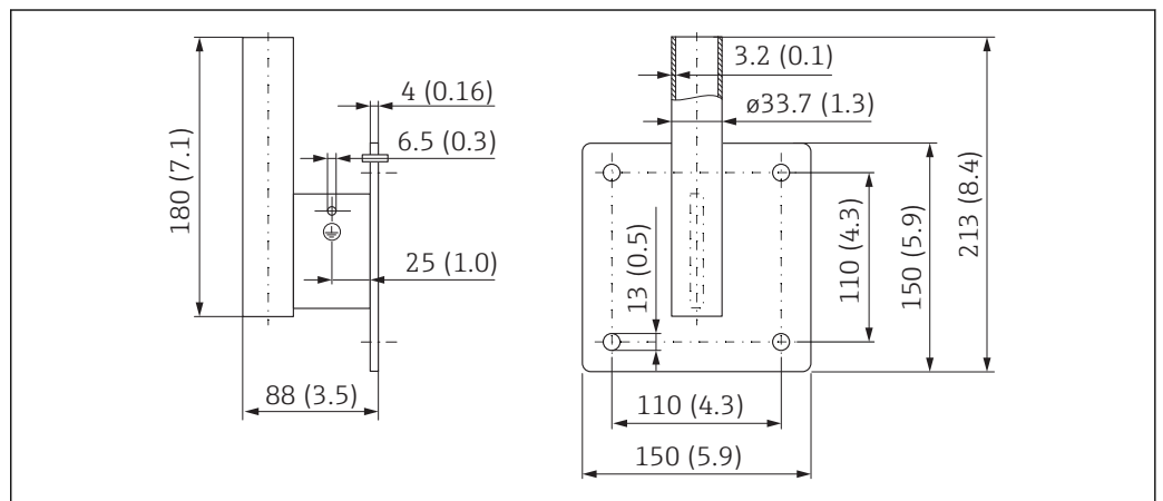
図 55 壁面ブラケットの寸法。測定単位 mm (in)
