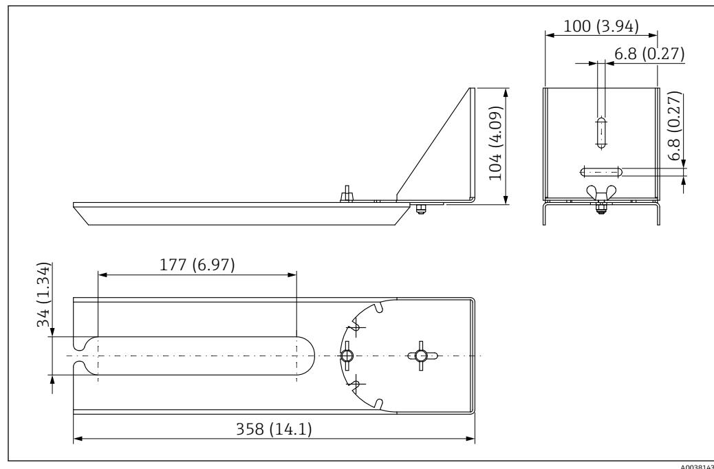
図 57 回転可能な取付ブラケットの寸法。測定単位 mm (in)
