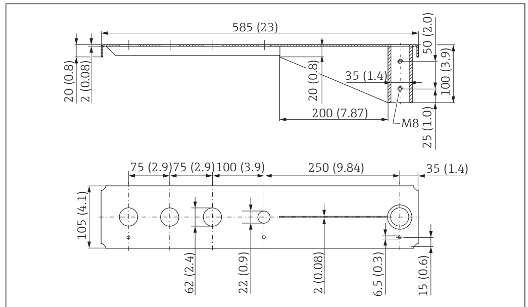
51 回転可能なセンササポート（ショート）、前面センサプロセス接続 G 2" の寸法。測定単位 mm (in)
