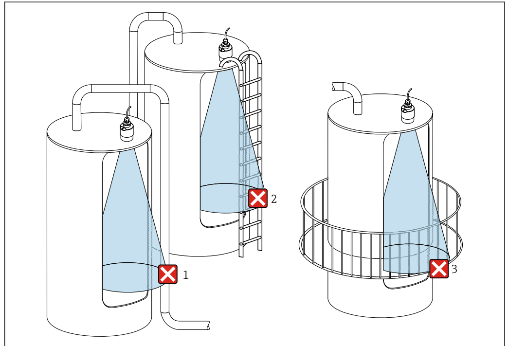
■ 15 金属製の干渉物がタンク外側にあるプラスチックタンク内の測定
