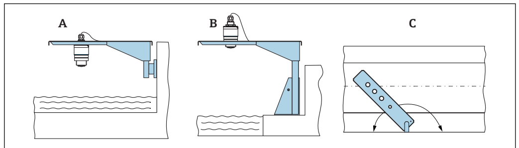
図 19 回転可能なカンチレバーによる設置
