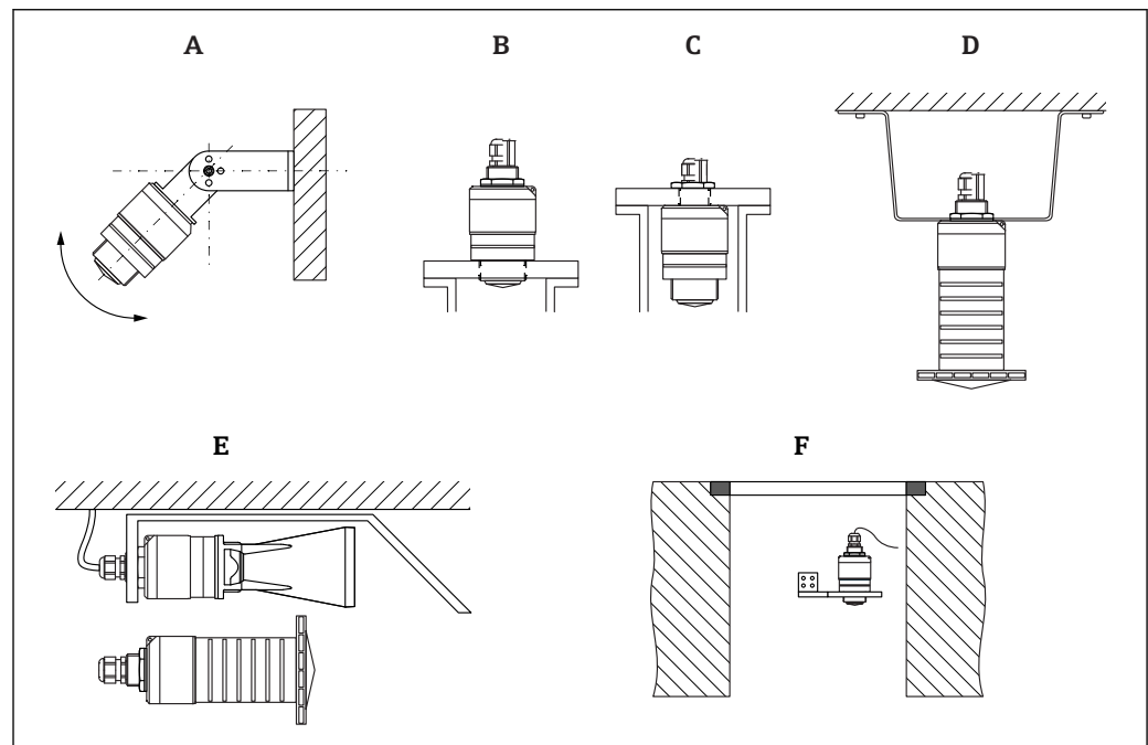
図 10 壁面、天井、またはノズル取付け
