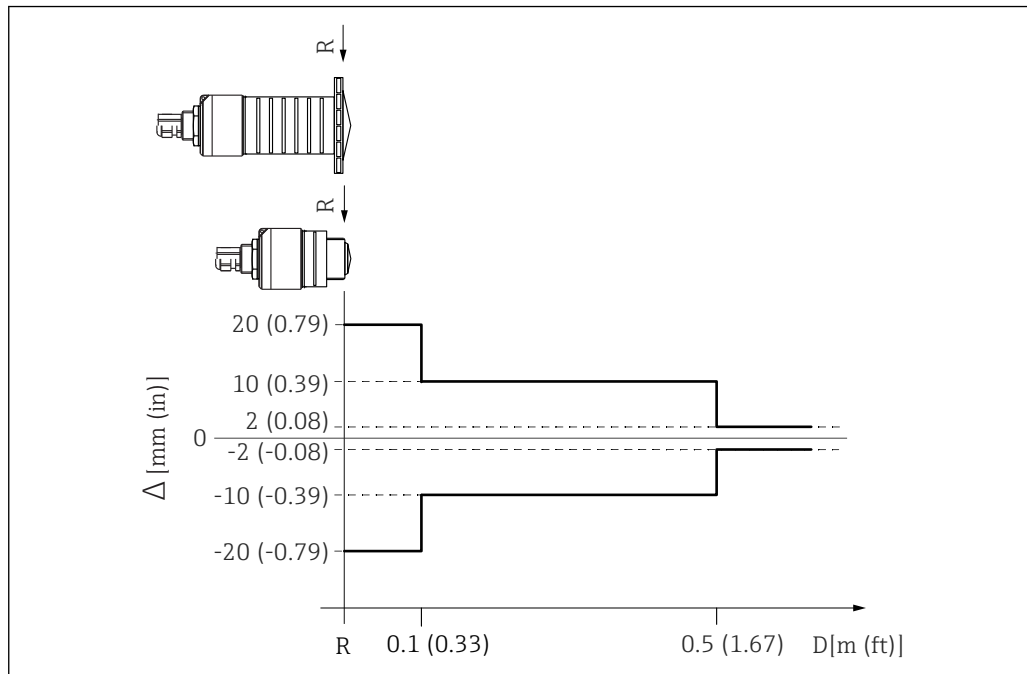
図 9 近範囲アプリケーションにおける最大測定誤差、標準バージョンの値
