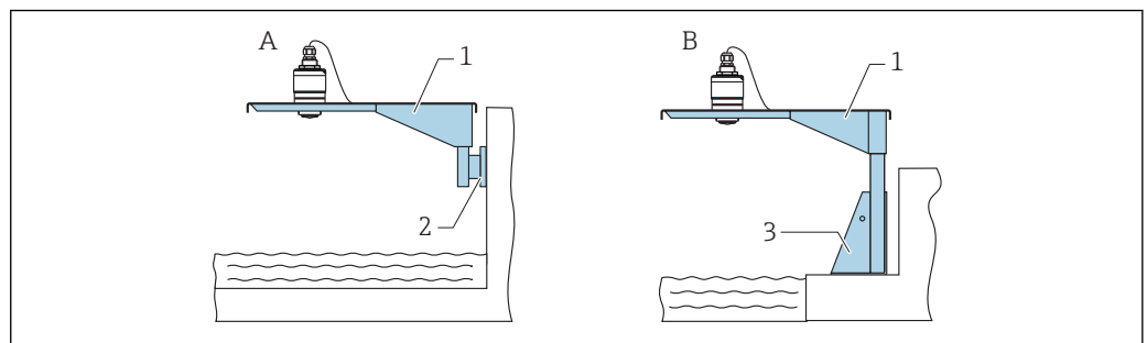
図 48 設置タイプ 前面センサプロセス接続
