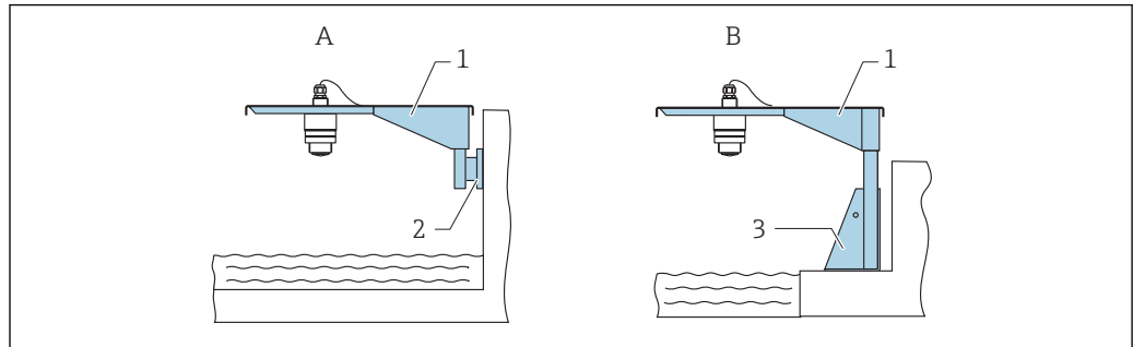
図 45 設置タイプ 背面センサプロセス接続
