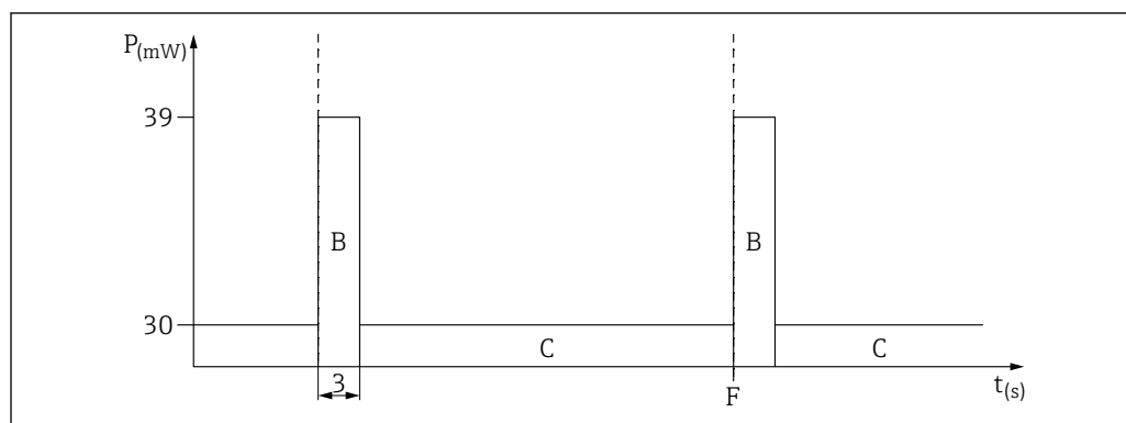
図 4 単発モードが常時オンの消費電力
