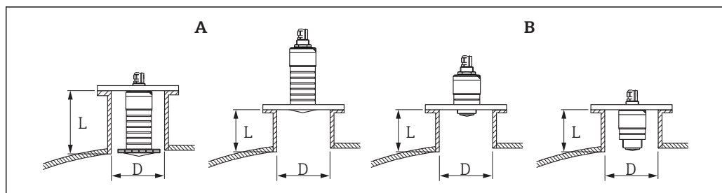
図 12 ノズル取付け
