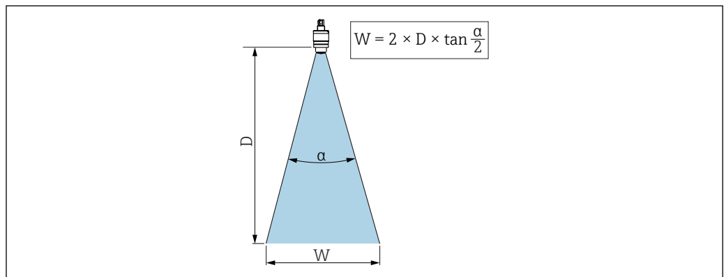
図 14 ビーム放射角 \alpha 、距離 D、ビーム幅 W の関係
