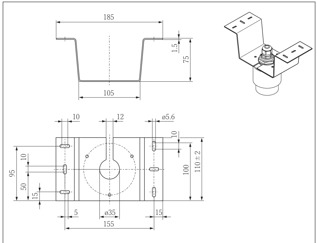
図 56 天井取付ブラケットの寸法。測定単位 mm (in)
