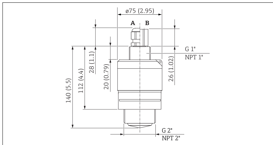
図 24 G 2" または MNPT 2" プロセス接続ネジの寸法、単位 : mm (in)
