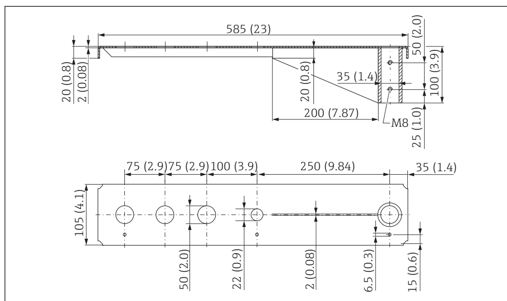
図 49 回転可能なセンササポート（ショート）、前面センサプロセス接続 G 1-½" の寸法。測定単位 mm (in)
