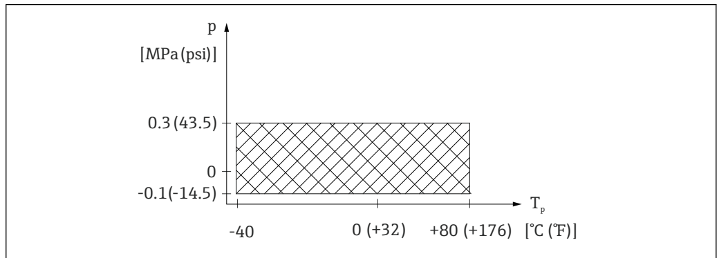
図 22 FMR20 : プロセス温度およびプロセス圧力の許容範囲
