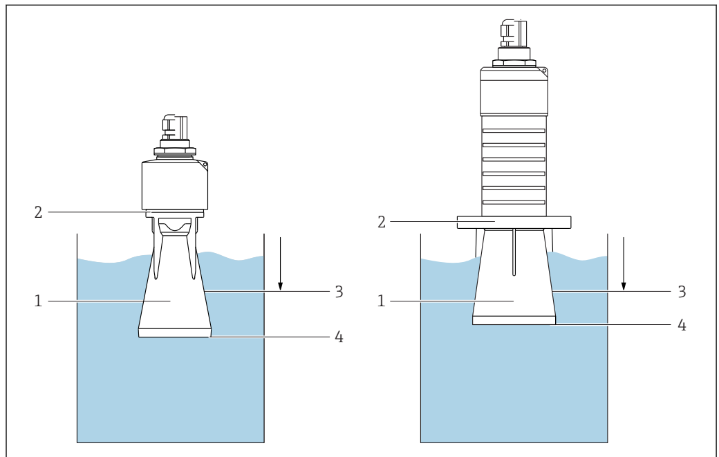
図 17 溢れ防止チューブの機能
