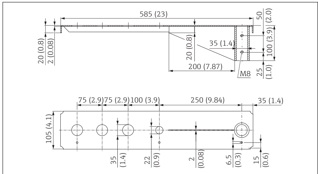
図 46 回転可能なセンササポート（ショート）、背面センサプロセス接続の寸法。測定単位 mm (in)
