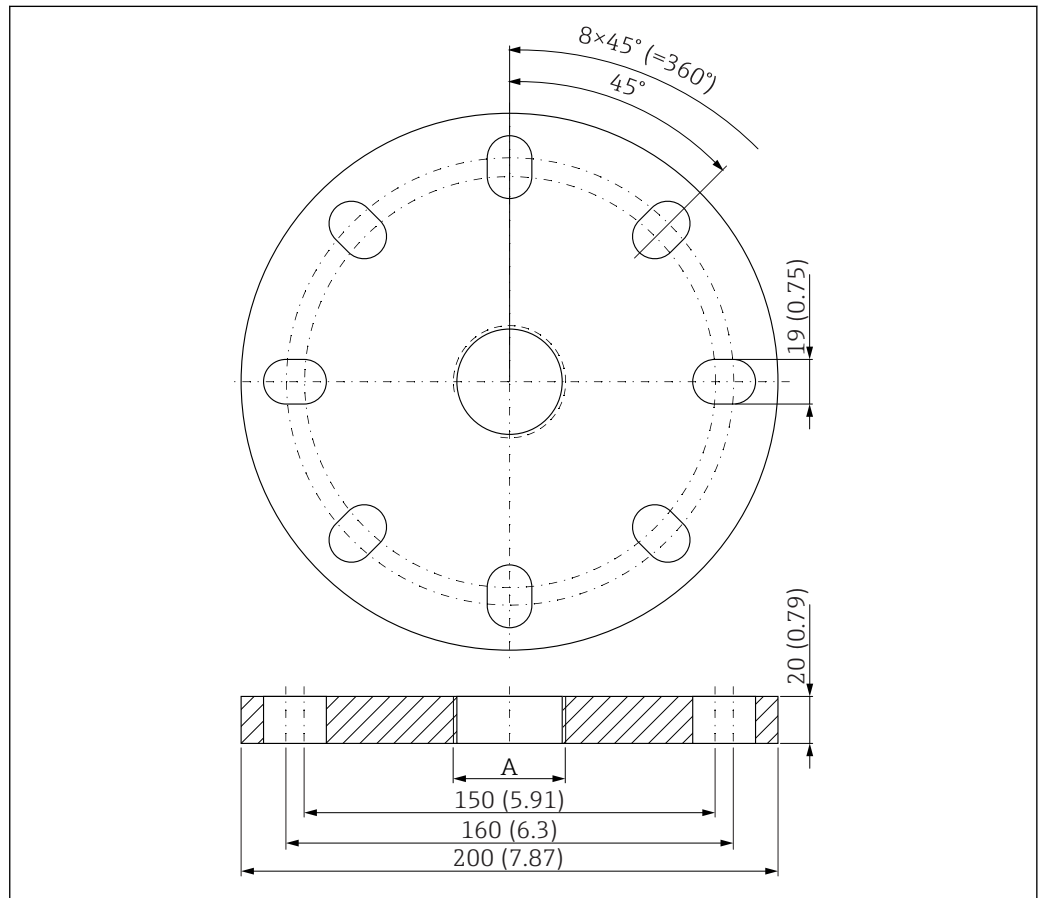
図 42 UNI フランジ 3"/DN80/80 の寸法、単位：mm (in)
