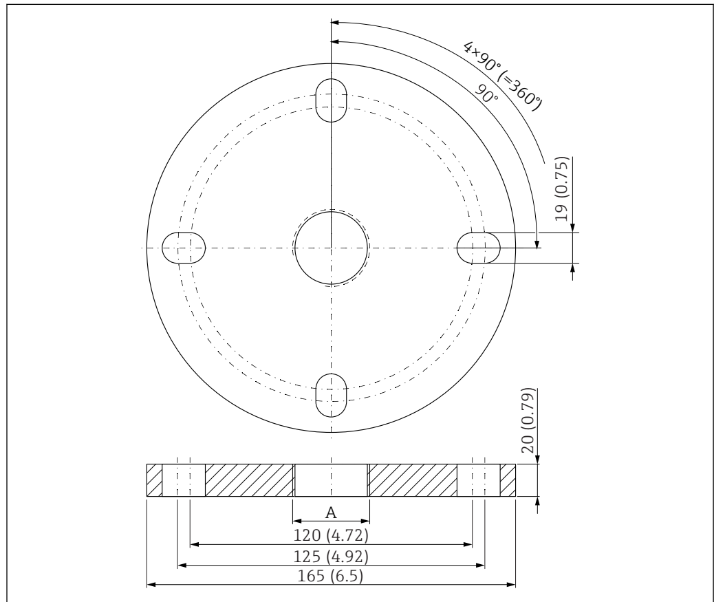
図 41 UNI フランジ 2"/DN50/50 の寸法、単位：mm (in)
