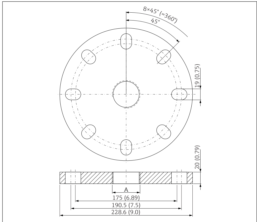
図 43 UNI フランジ 4"/DN100/100 の寸法、単位：mm (in)
