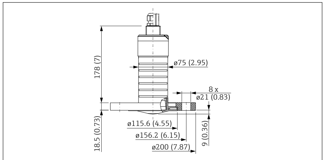
■ 28 スリップオンフランジ 3"/DN80 付き 80 mm (3 in) アンテナの寸法、単位：mm (in)
