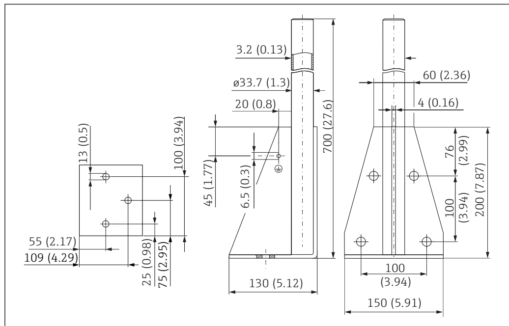
図 53 取付フレーム（ショート）の寸法。測定単位 mm (in)
