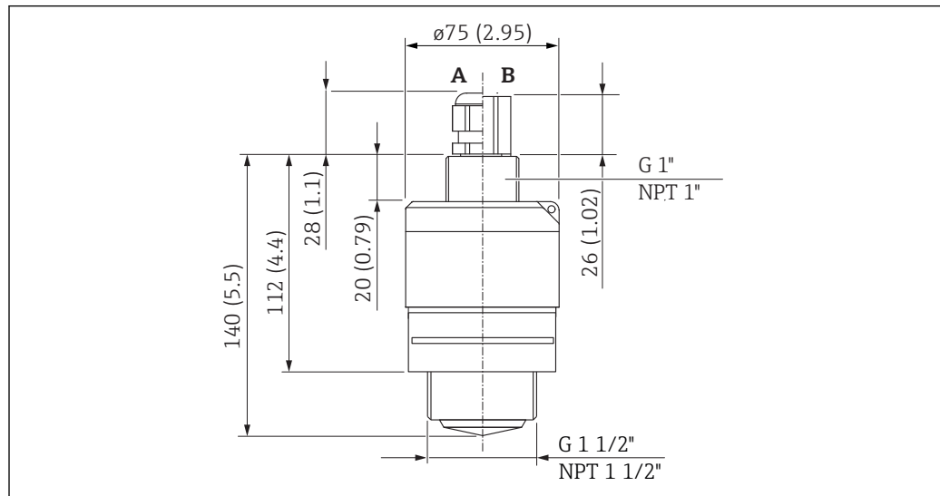
図 23 G 1-½" または MNPT 1-½" プロセス接続ネジの寸法、単位 : mm (in)
