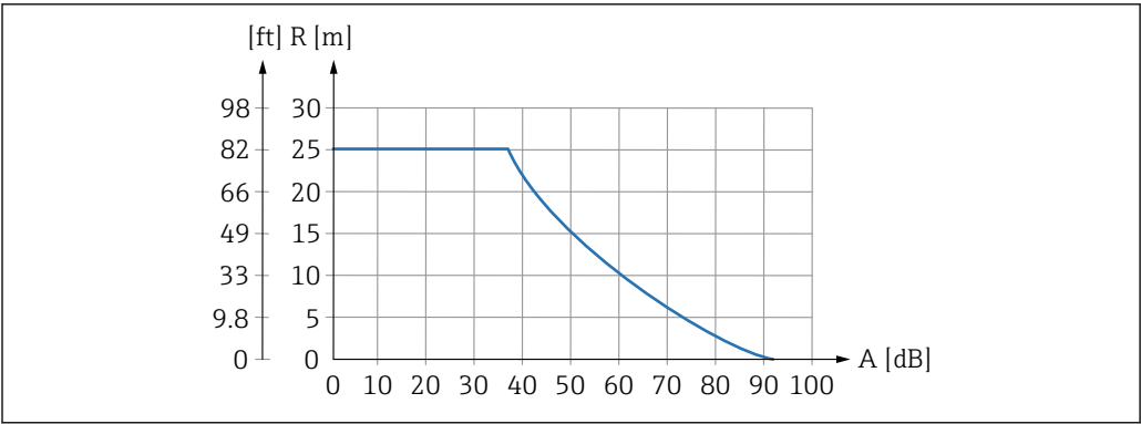
2 Diagramme de portée pour les capteurs à ultrasons
