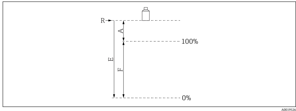
図 10 スパンを定義するための変数
