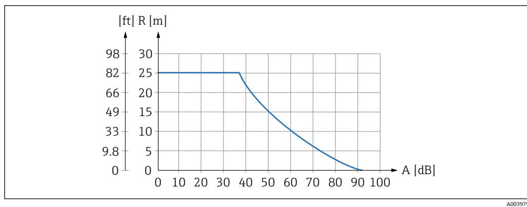
図 2 超音波センサの範囲グラフ
