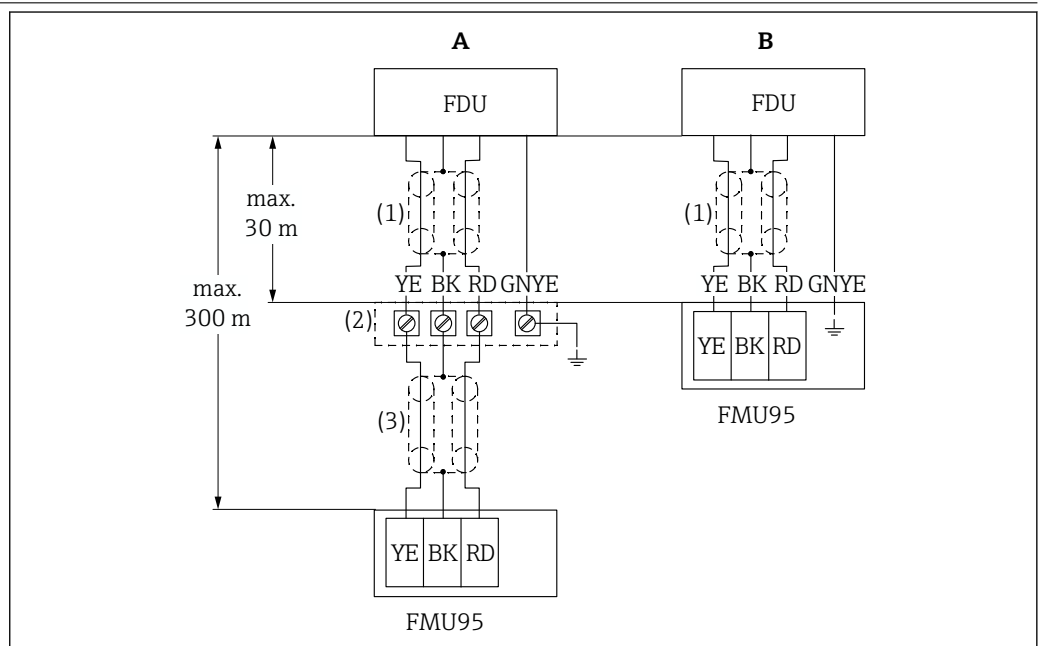
■ 4 センサの接続図；YE：黄色、BK：黒色、RD：赤色、BU：青色、BN：茶色；保護導体 GNYE：緑色/黄色
