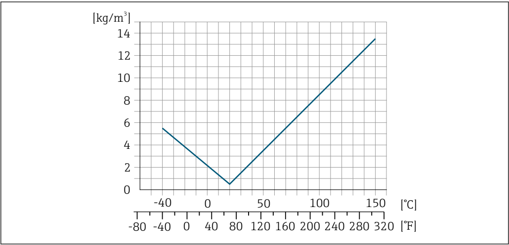
42 Калибровка по плотности на месте эксплуатации, в примере при +20 °C (+68 °F)
