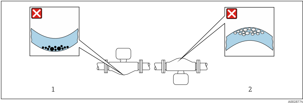
8 Монтажная позиция датчика с изогнутой измерительной трубкой
