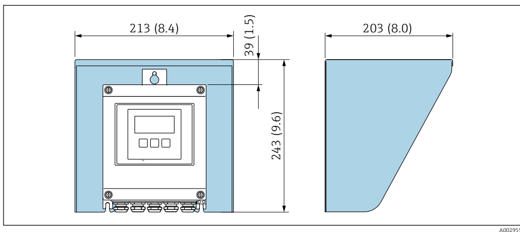
10 Защитный козырек для прибора Proline 500 в цифровом исполнении; единицы измерения – мм (дюймы)
