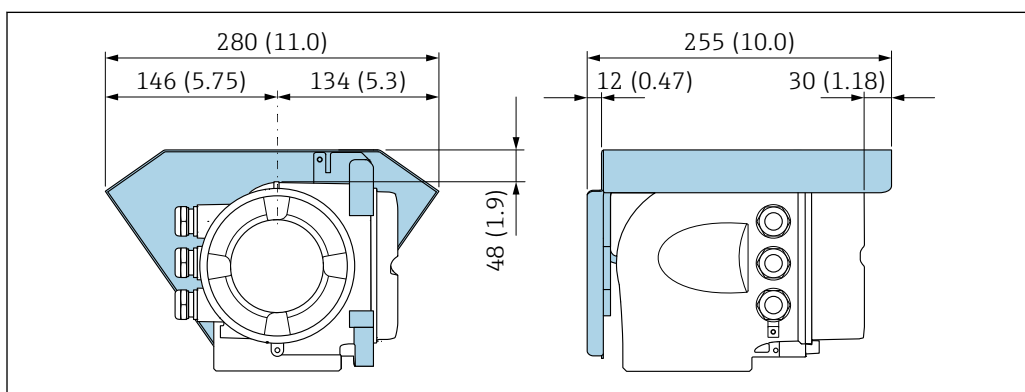
11 Защитный козырек для прибора Proline 500; единицы измерения – мм (дюймы)
