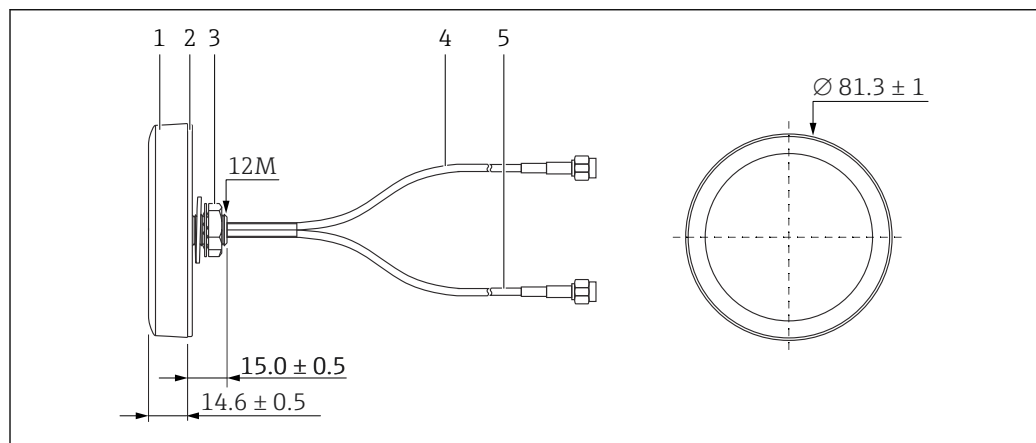
19 Antena LTE
