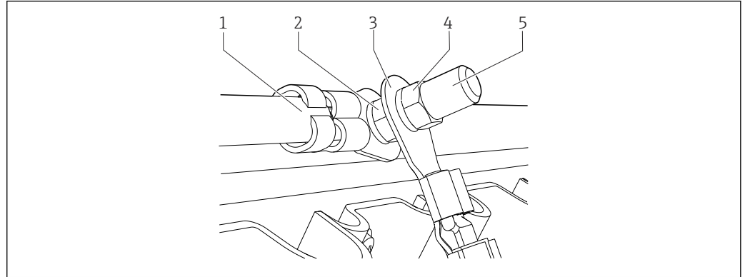
16 Podłączenia uziemienia ochronnego lub uziemienia roboczego
