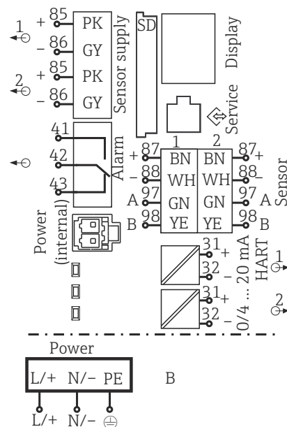
15 Schemat podłączeń modułu centralnego BASE-E i dodatkowego zasilacza (B)
