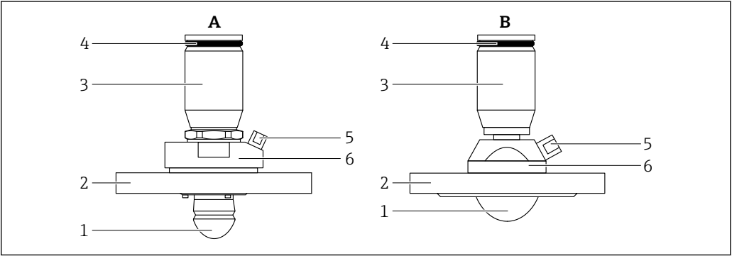
A ドリップオフアンテナ DN50 B フラッシュマウント型アンテナ DN80
