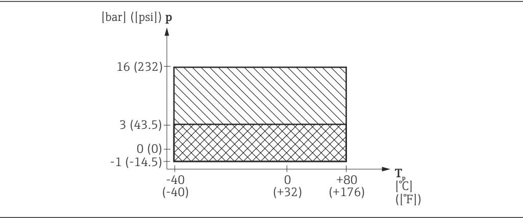
図 18 FMR67 : プロセス温度およびプロセス圧力の許容範囲、ドリップオフアンテナ、PTFE DN50
