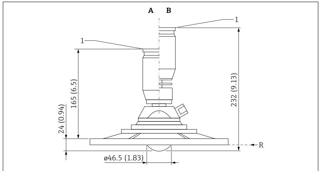
■ 32 アンテナ（UNI フランジ、角度調節器、エアーパージコネクション付き）の寸法。測定単位 mm (in)
