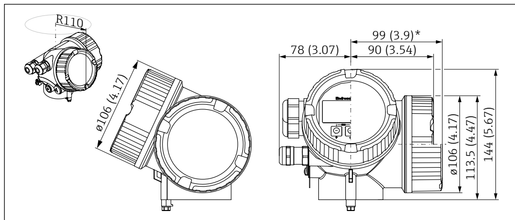
図 23 GT19 ハウジング (プラスチック PBT)。測定単位 mm (in)
