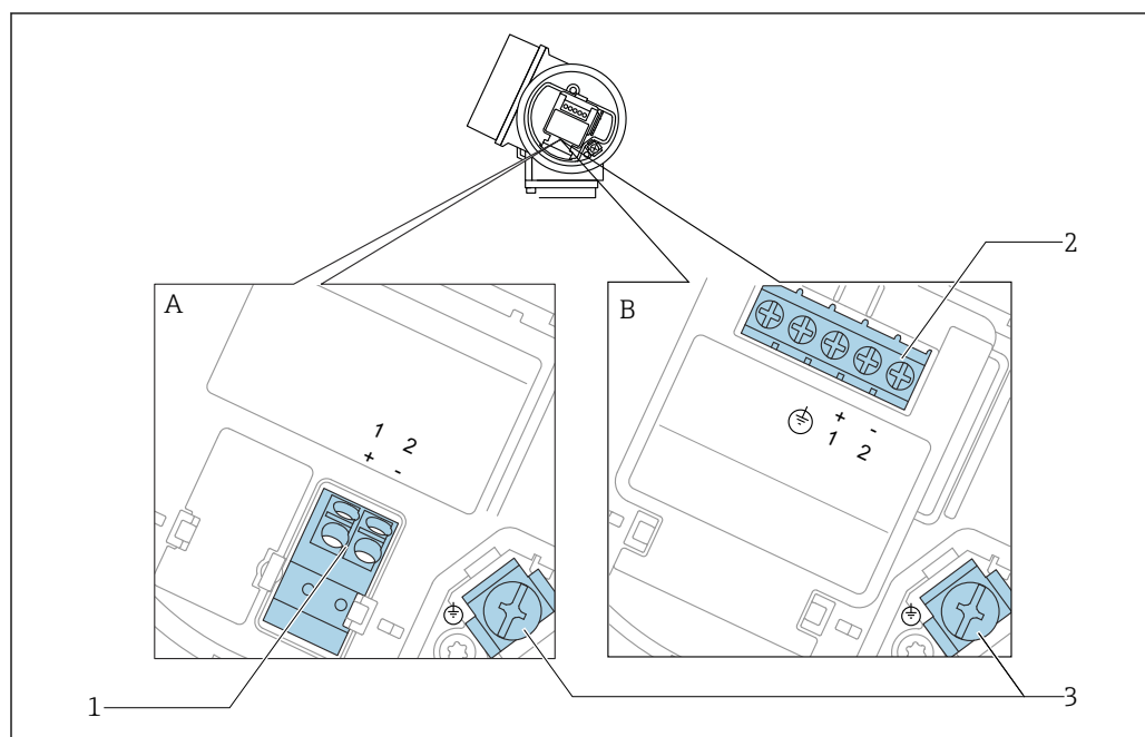
図 3 2 線式、4-20 mA HART の端子割当て
