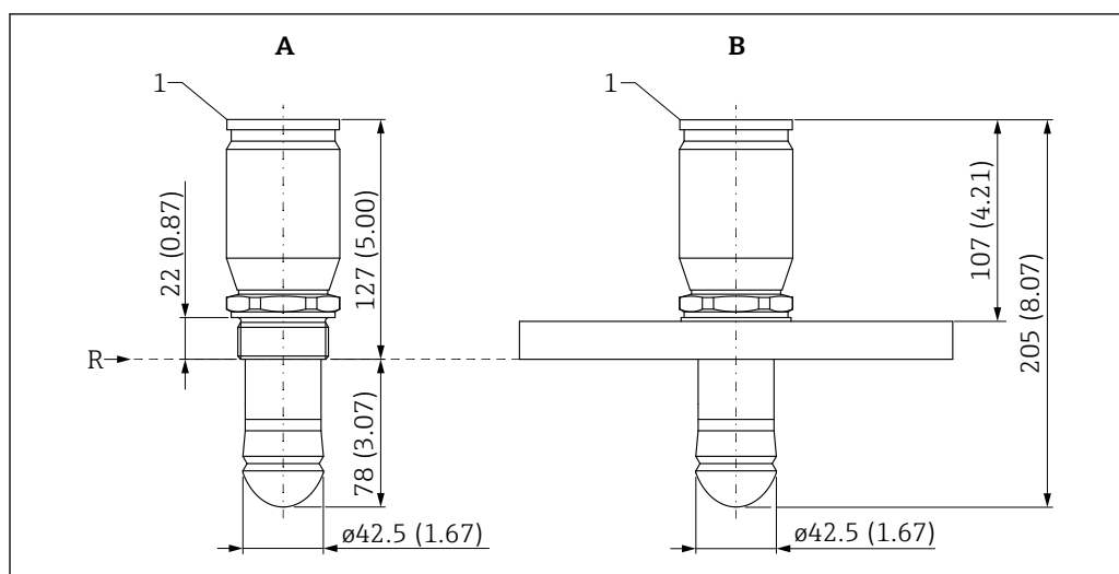
図 25 ドリップオフアンテナ（エアージャコネクションなし）の寸法。測定単位 mm (in)
