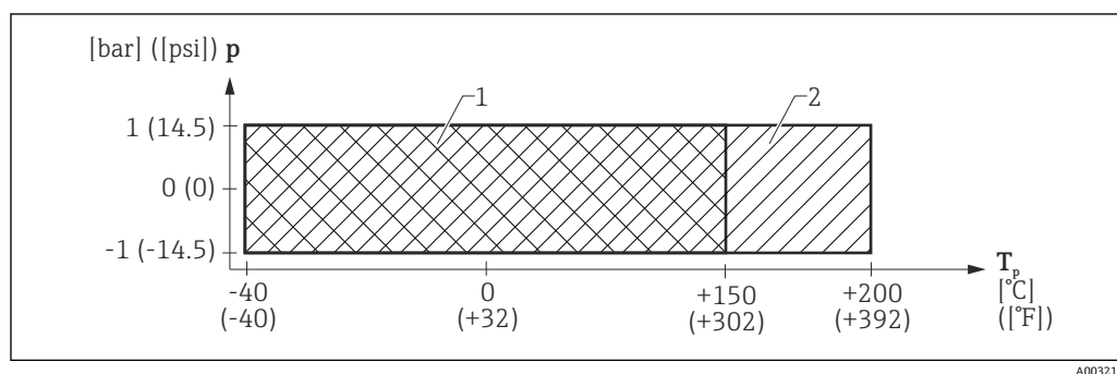
図 21 FMR67：プロセス温度およびプロセス圧力の許容範囲、アンテナ、PTFE DN80、UNI フランジ、アルミニウム、調整可能
