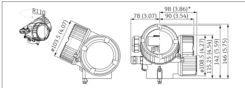
図 22 ハウジング GT18 (SUS 316L 相当)。測定単位 mm (in)
