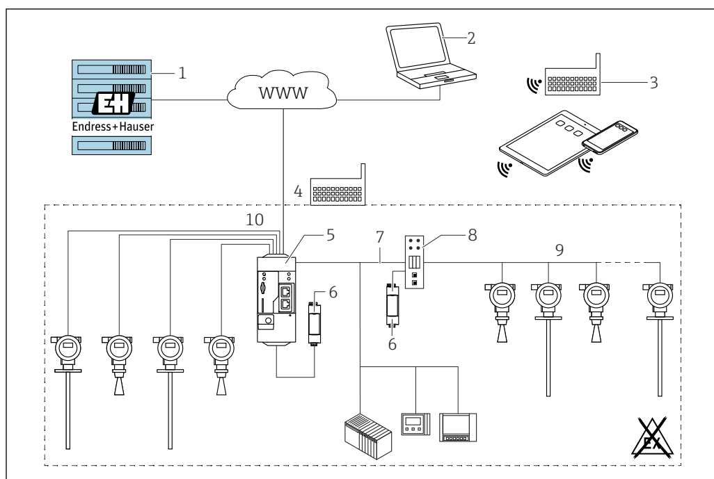
図 40 SupplyCare Hosting SCH30 を使用した在槽管理プラットフォームの例
