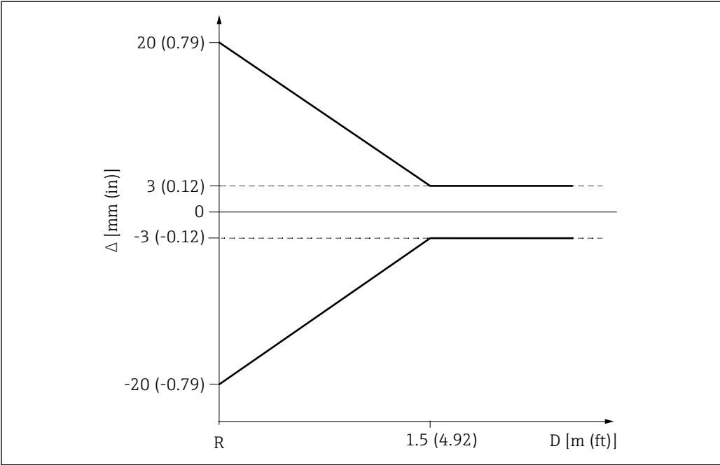
図 13 近範囲アプリケーションにおける最大測定誤差
