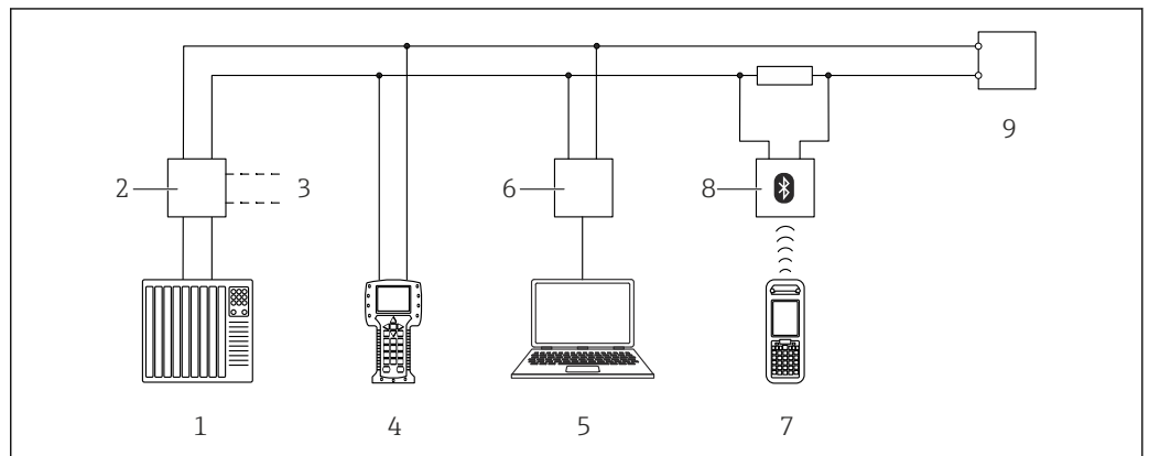
図 37 HART 経由のリモート操作オプション
