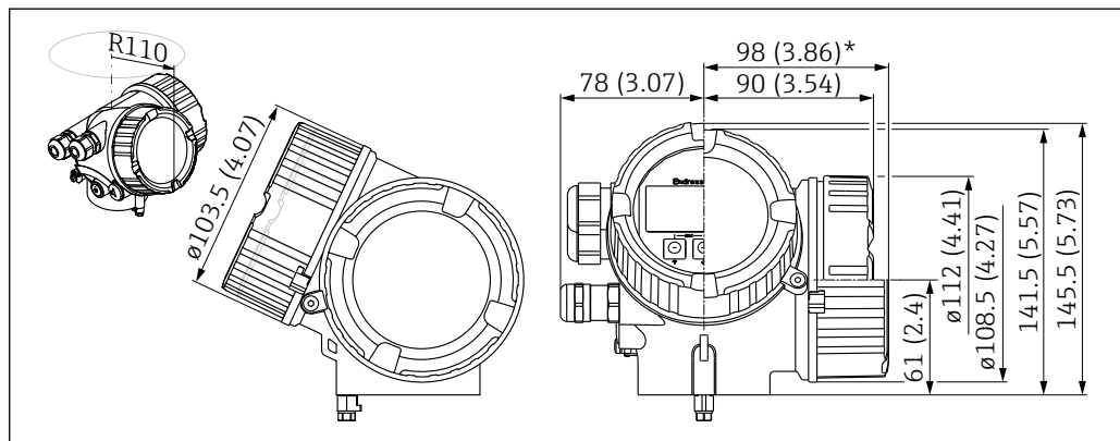
図 24 ハウジング GT20 (アルミダイカスト、塗装)。測定単位 mm (in)
