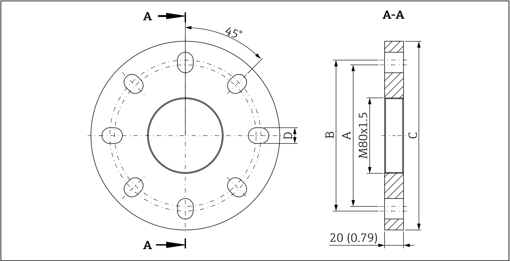
28 FMR67 用の UNI フランジ（エアパージコネクション付き）の寸法。測定単位 mm (in)
