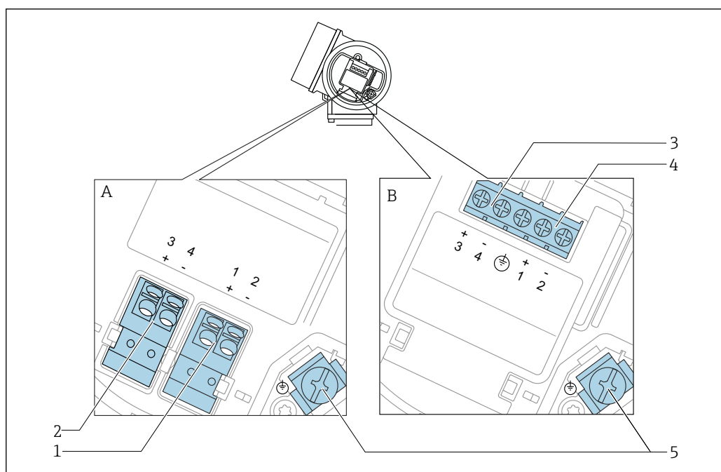
5 2線式、4~20 mA HART、スイッチ出力の端子割当て
