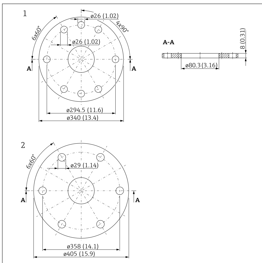
図 31 FMR67 用の UNI フランジ (エアージャコネクション付き) の寸法。測定単位 mm (in)
