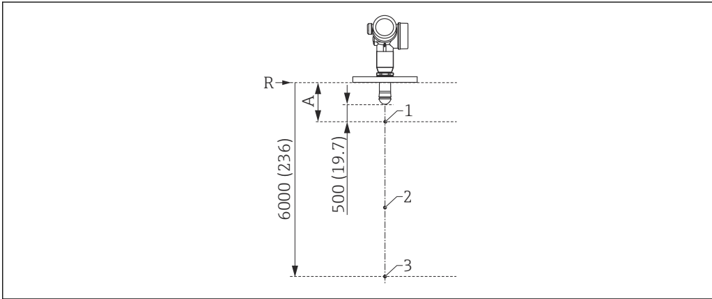
図 41 3 点リニアリティプロトコルの各点。測定単位 mm (in)
