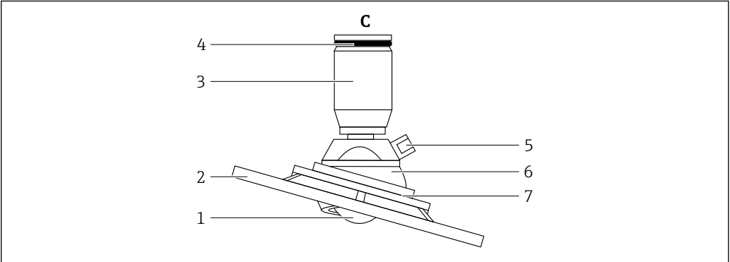
C フラッシュマウント型アンテナ DN80、角度調節器付き
