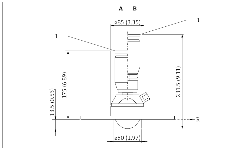
図 30 アンテナ（UNI フランジおよびエアーパージコネクション付き）の寸法。測定単位 mm (in)
