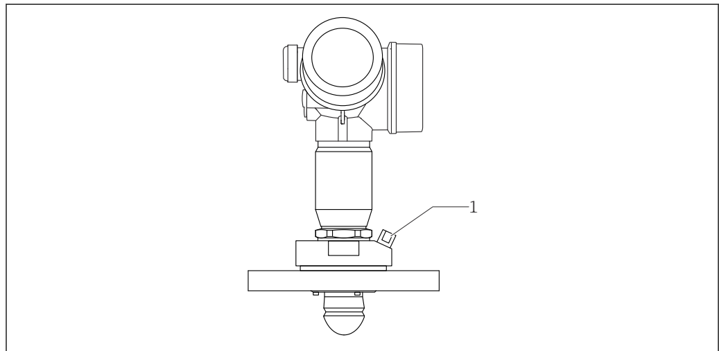
図 16 ドリップアンテナ用のパージエアアダプタ
