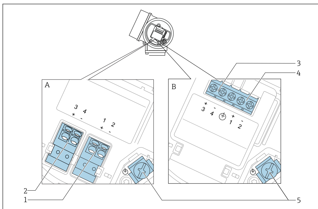
図 7 2 線式、4～20 mA HART、4～20 mA の端子割当て
