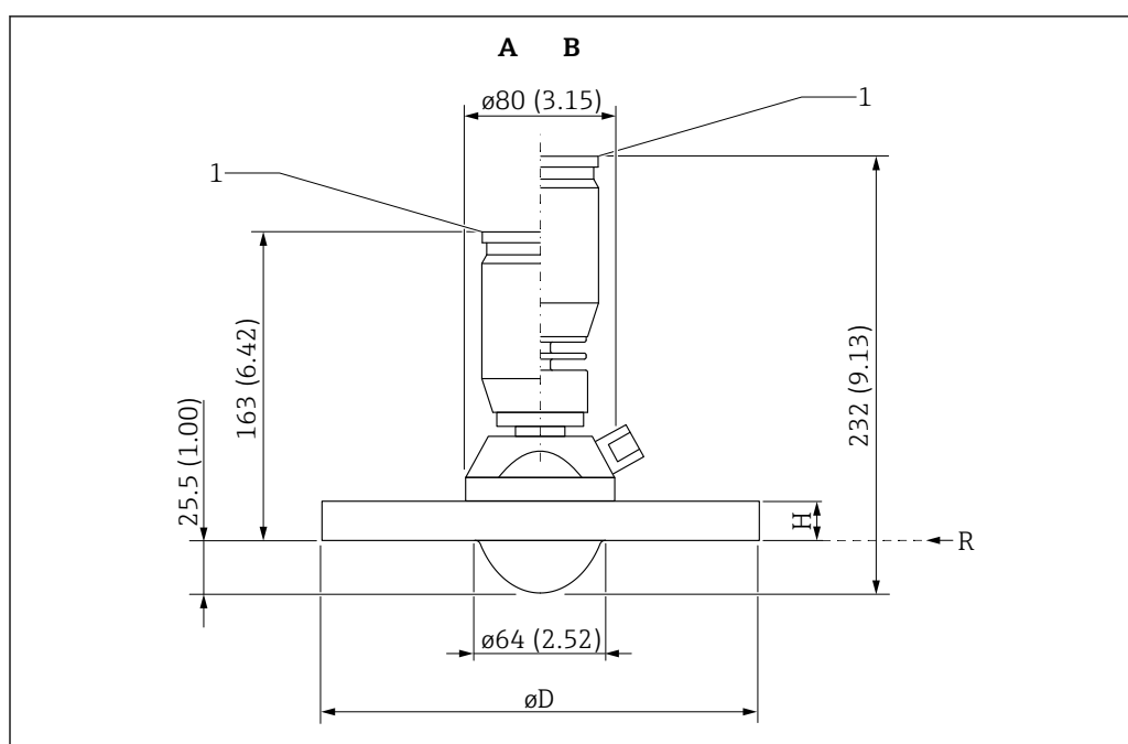
図 29 フラッシュマウントアンテナ（標準フランジおよびエアージャコネクション付き）の寸法。測定単位 mm (in)
