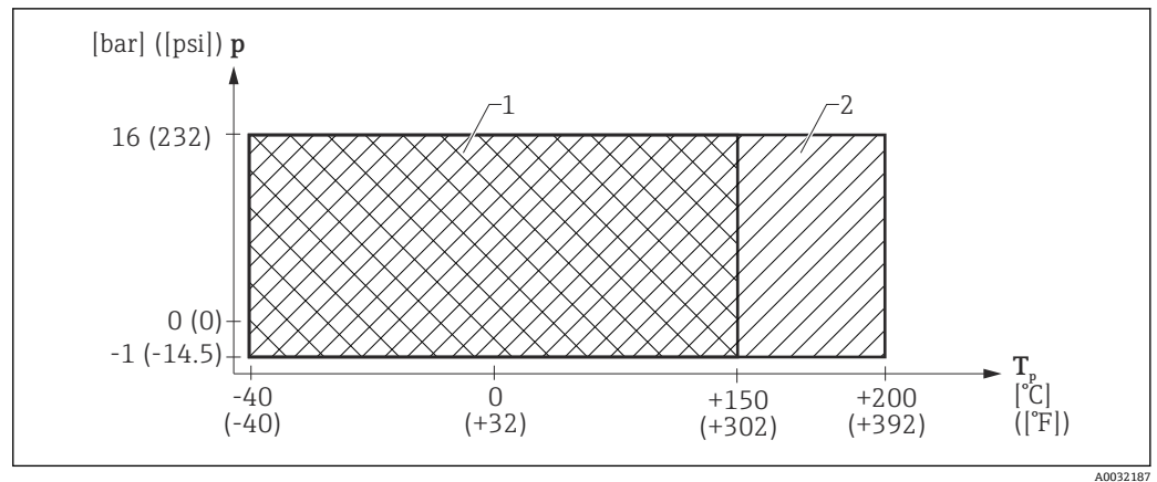
図 19 FMR67：プロセス温度およびプロセス圧力の許容範囲、アンテナ、PTFE DN80、標準フランジ SUS 316L 相当
