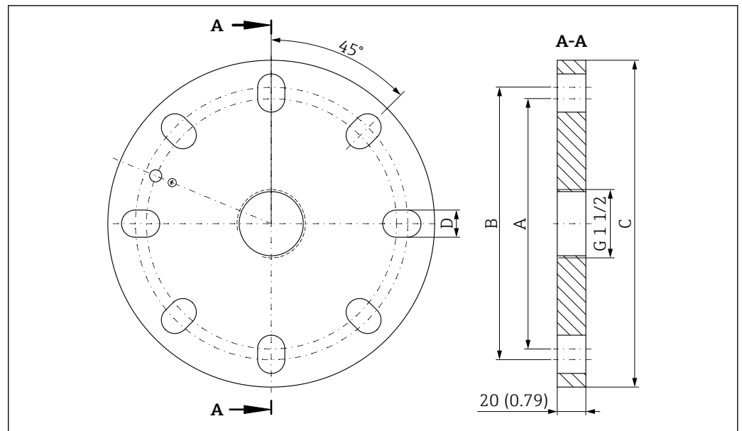
図 26 FMR67 用の UNI フランジ（エアージャコネクションなし）の寸法。測定単位 mm (in)
