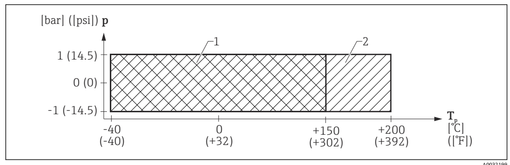
図 20 FMR67：プロセス温度およびプロセス圧力の許容範囲、アンテナ、PTFE DN80、UNI フランジ SUS 316L 相当
