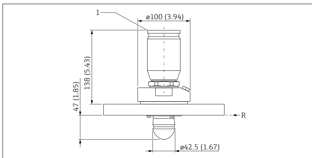
図 27 ドリップオフアンテナ（エアージャコネクション付き）の寸法。測定単位 mm (in)
