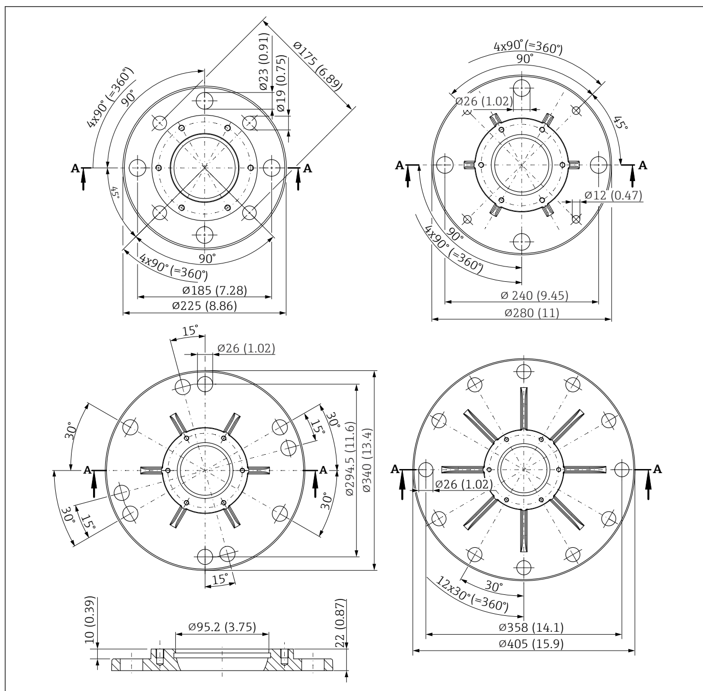
図 33 FMR67 用の UNI フランジ（角度調節器およびエアージャコネクション付き）の寸法。測定単位 mm (in)
