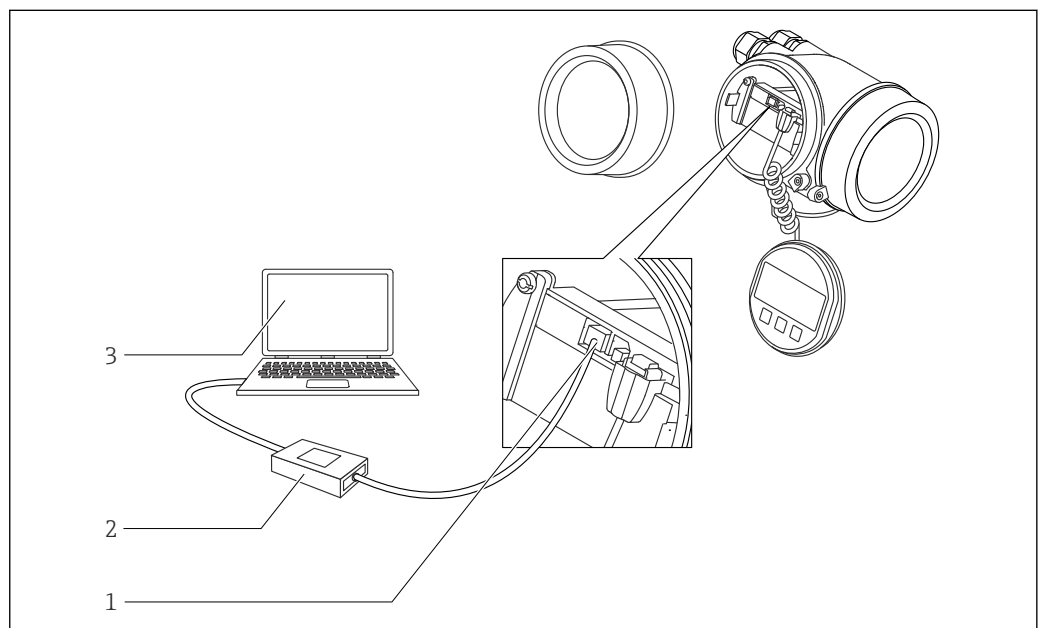
図 38 サービスインターフェイス (CDI) 経由の DeviceCare/FieldCare
