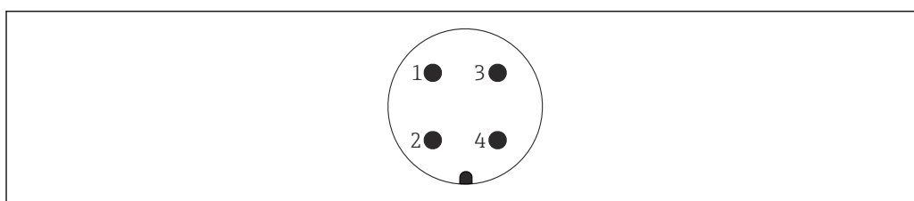
図 12 7/8" プラグのピン割当て
