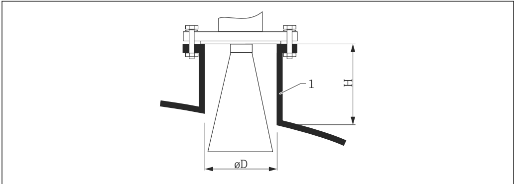
7 Altezza e diametro del tronchetto per antenna a cono (FMR54)
