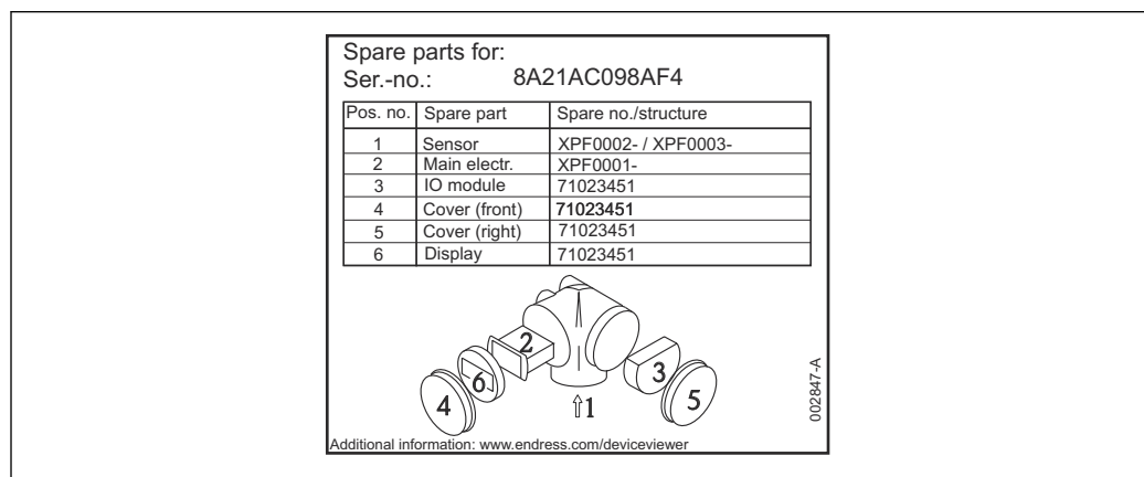
28 Esempio di etichetta della parte di ricambio nel coperchio del vano connessioni
