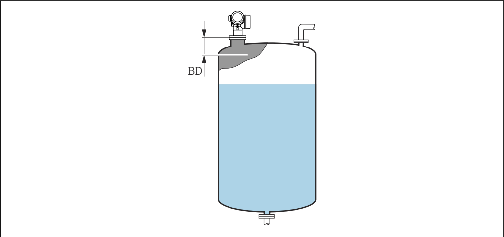
34 Distanza di blocco (BD) per misure di liquidi
