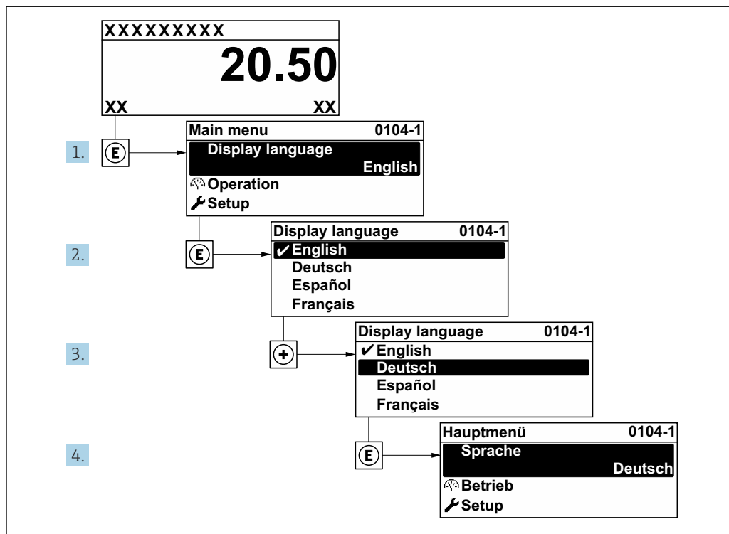
30 Pozycje menu wyświetlane na wyświetlaczu wskaźnika lokalnego
