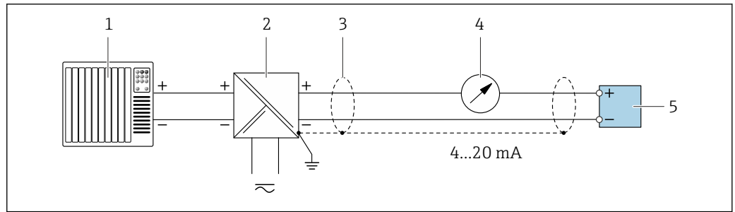
12 Przykład podłączenia wersji z pasywnym wyjściem prądowym 4...20 mA HART
