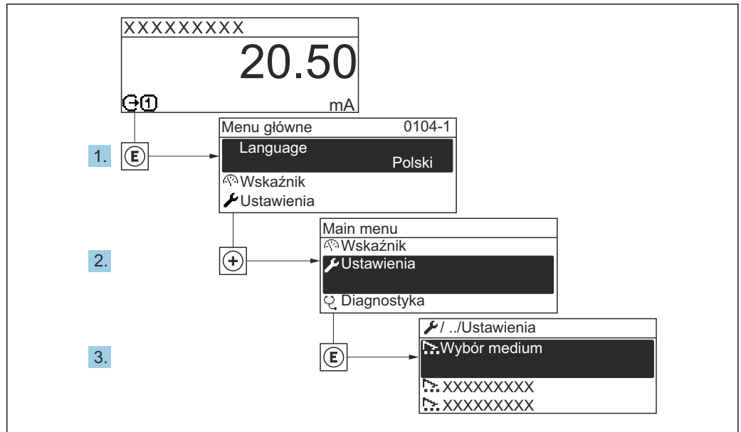
31 Przykład menu na wyświetlaczu lokalnym
