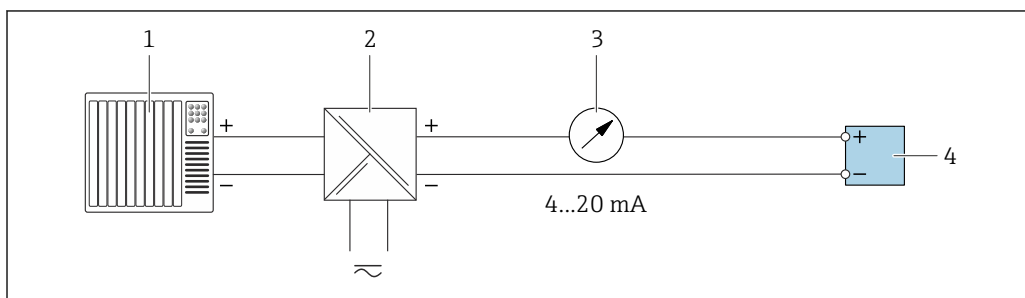
15 Przykład podłączenia wyjścia prądowego 4-20 mA (pasywnego)
