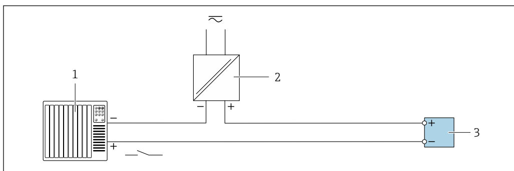
22 Przykład podłączenia wejścia statusu
