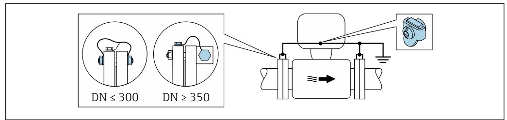
9 Wyrównanie potencjałów poprzez podłączenie obu kołnierzy rurociągu do zacisku uziemiającego przetwornika
