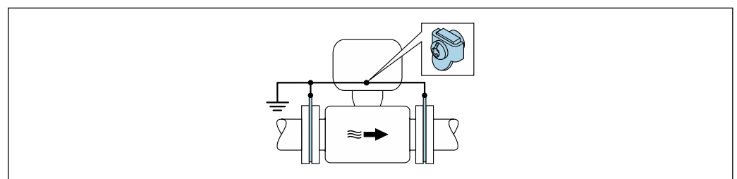
10 Wyrównanie potencjałów realizowane jest za pomocą dodatkowych pierścieni uziemiających, podłączonych do zacisku uziemiającego przewodem uziemiającym
