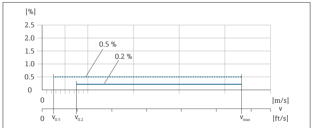
38 Płaska charakterystyka błędu; błąd w % w.w.
