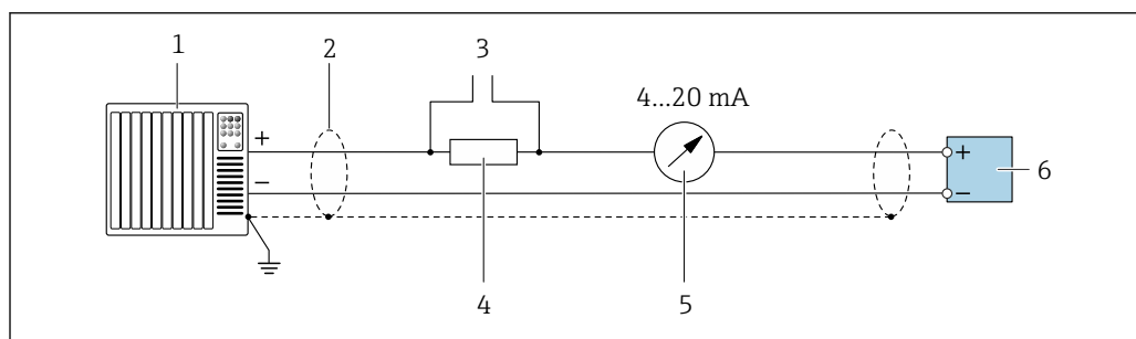
11 Przykład podłączenia wersji z aktywnym wyjściem prądowym 4...20 mA HART
