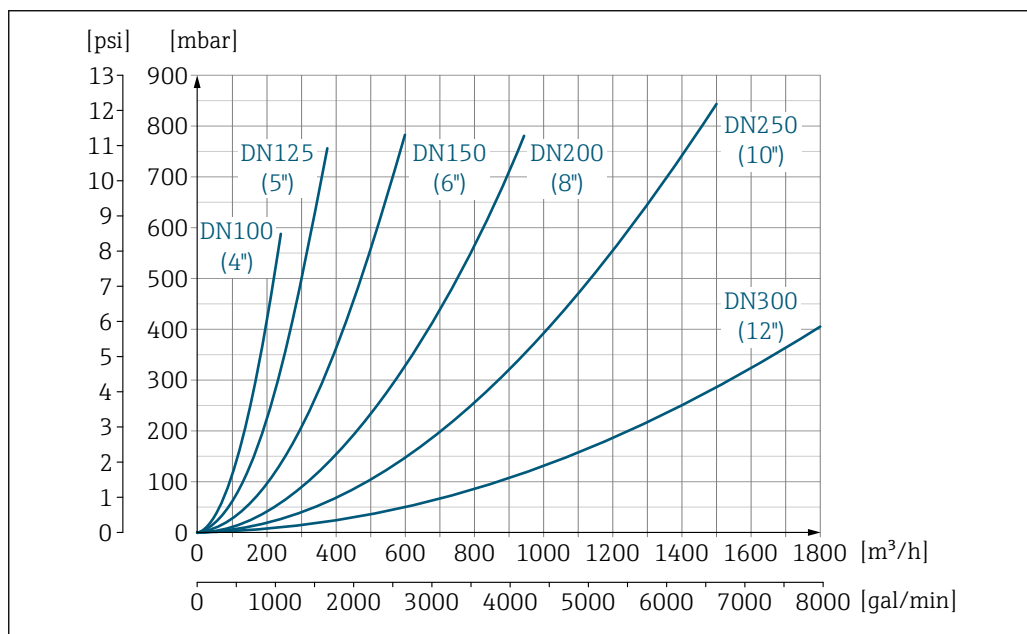
40 Straty ciśnienia: DN 100-300 (4-12"), pozycja kodu zam. "Konstrukcja", opcja C "Kołnierz stały, bez prostoliniowych odcinków dolotowych i wylotowych"
