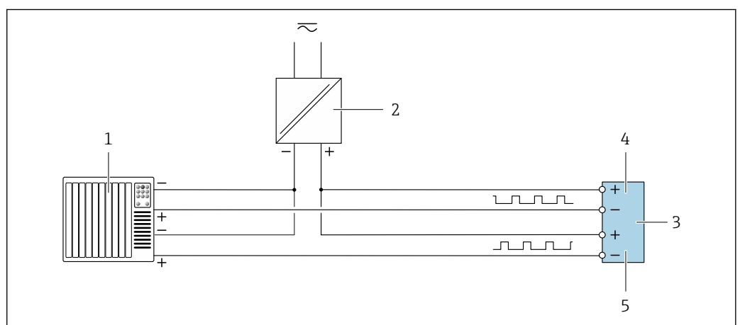
19 Przykład podłączenia wersji z podwójnym wyjściem impulsowym (pasywnym)
