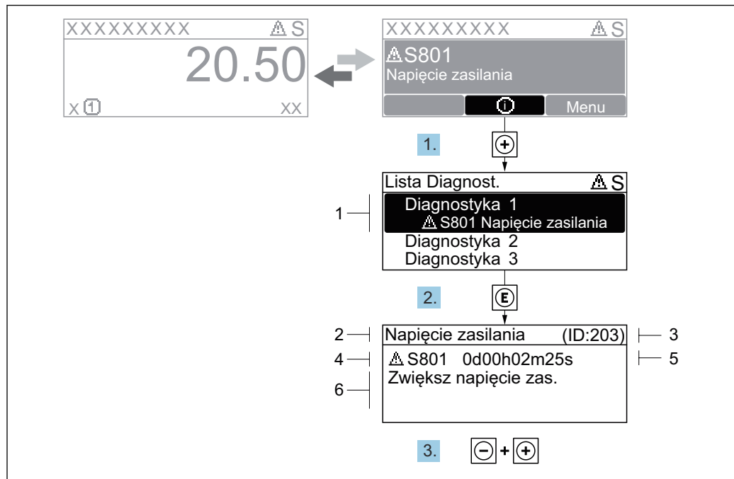
33 Komunikat o możliwych działaniach
