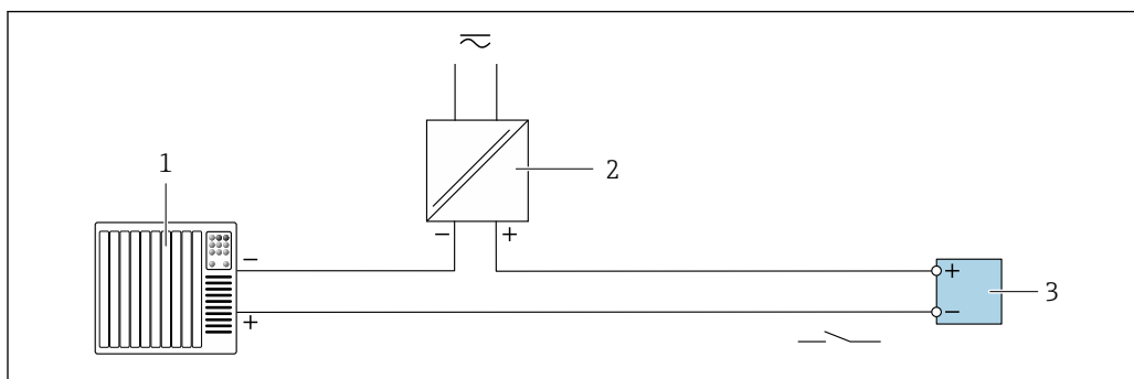
20 Przykład podłączenia wyjścia przekaźnikowego (pasywnego)
