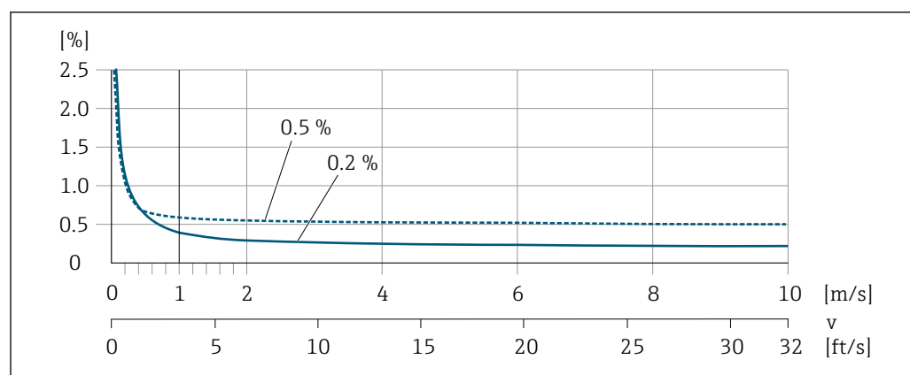
24 Maksymalny błąd pomiaru w % w.w.
