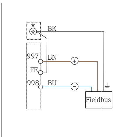
26 Aansluitschema
