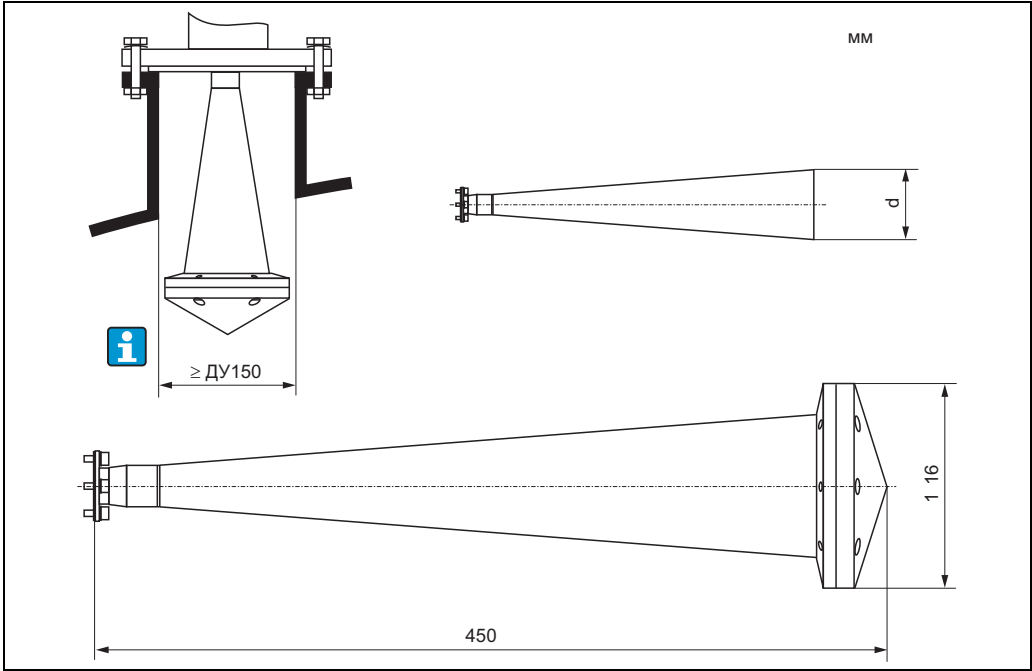
Крышка рупора для рупорной антенны 100 мм – для антенны диаметром d = 95 мм – для FMR240: вариант антенны Н, 5 – для FMR250: вариант антенны Е
