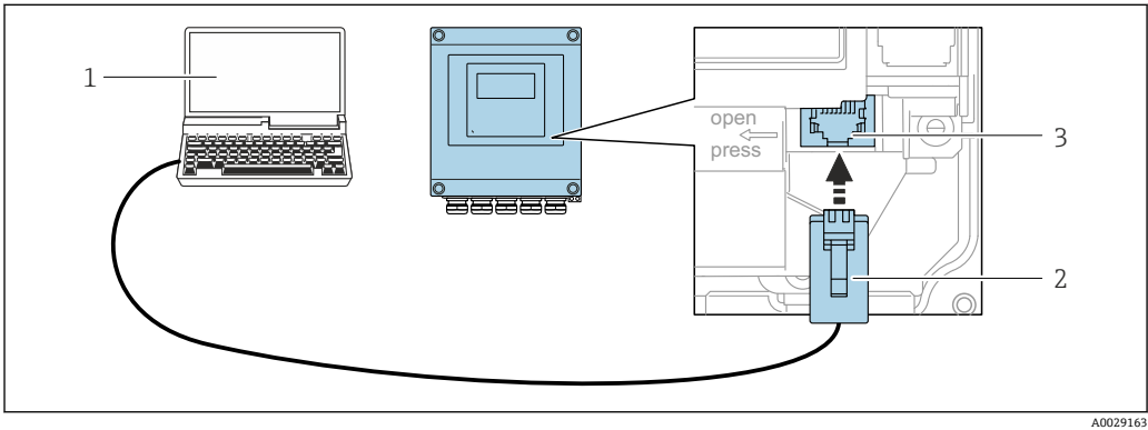
图 31 通过服务接口 (CDI-RJ45) 操作
