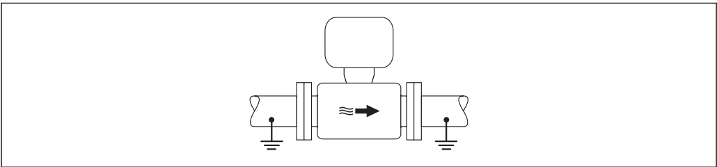
图 17 通过测量管实现电势平衡
