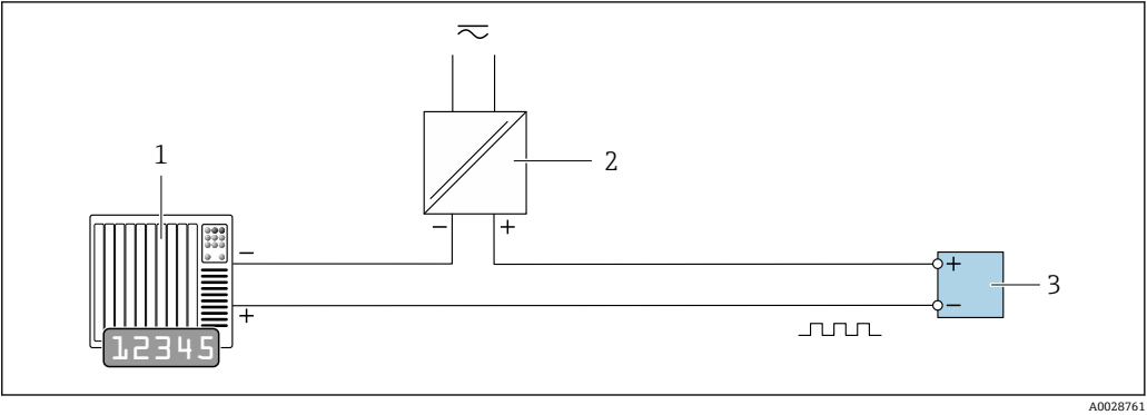
23 脉冲/频率输出(无源信号)的连接实例
