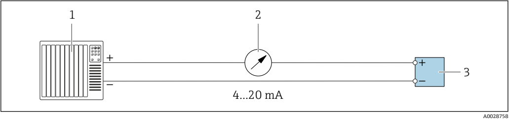
21 4...20 mA 有源电流输出的连接实例
