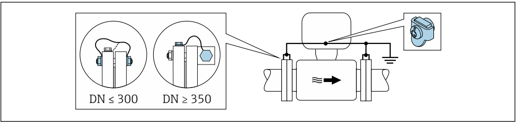
图 18 通过接地端子和管道法兰实现电势平衡
