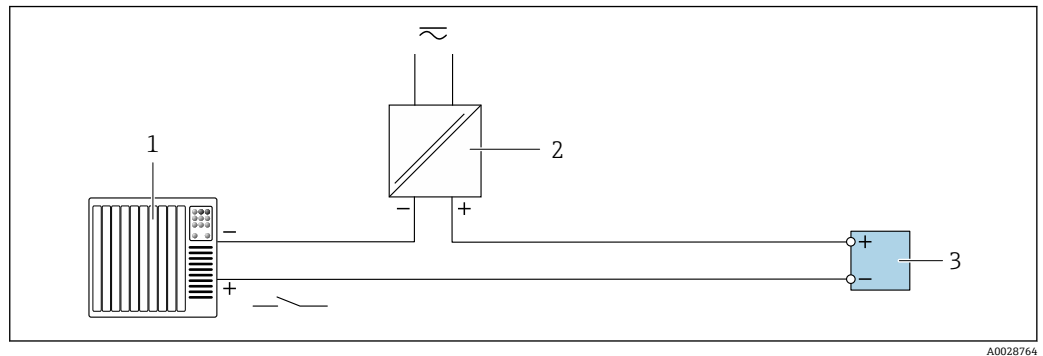
图 27 状态输入的连接实例
