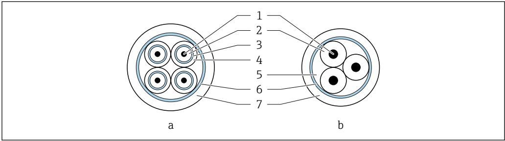
图 14 电缆横截面积
