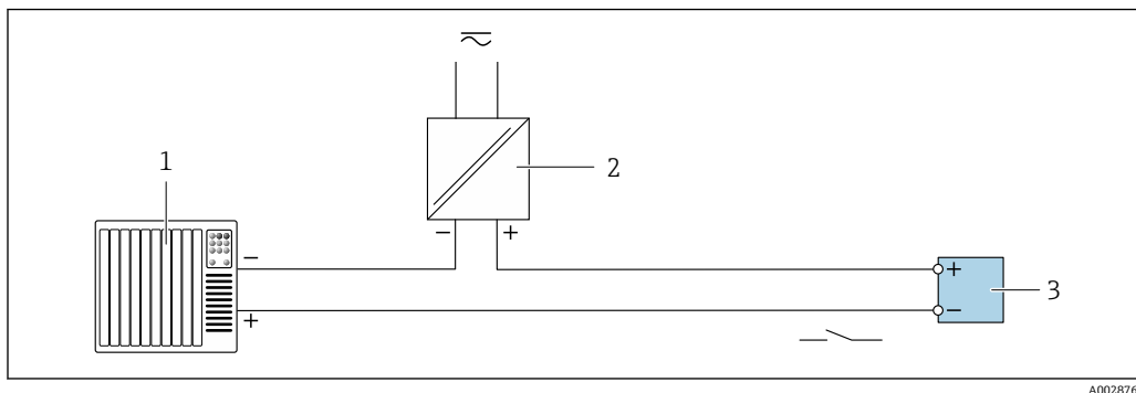
图 24 开关量输出(无源信号)的连接实例
