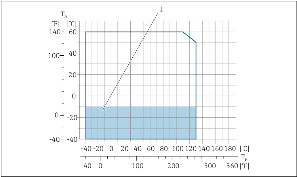
43 PTFE TA 环境温度范围 TF 流体温度 1 灰色区域: -10 ... -40 °C (+14 ... -40 °F)环境温度范围仅适用于不锈钢法兰
