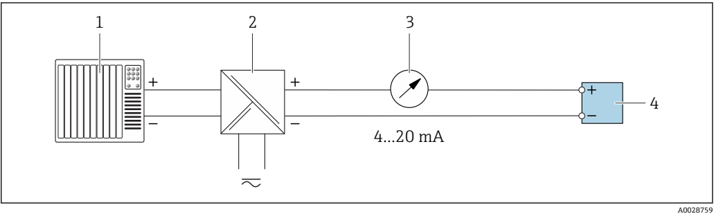
22 4...20 mA 无源电流输出的连接实例
