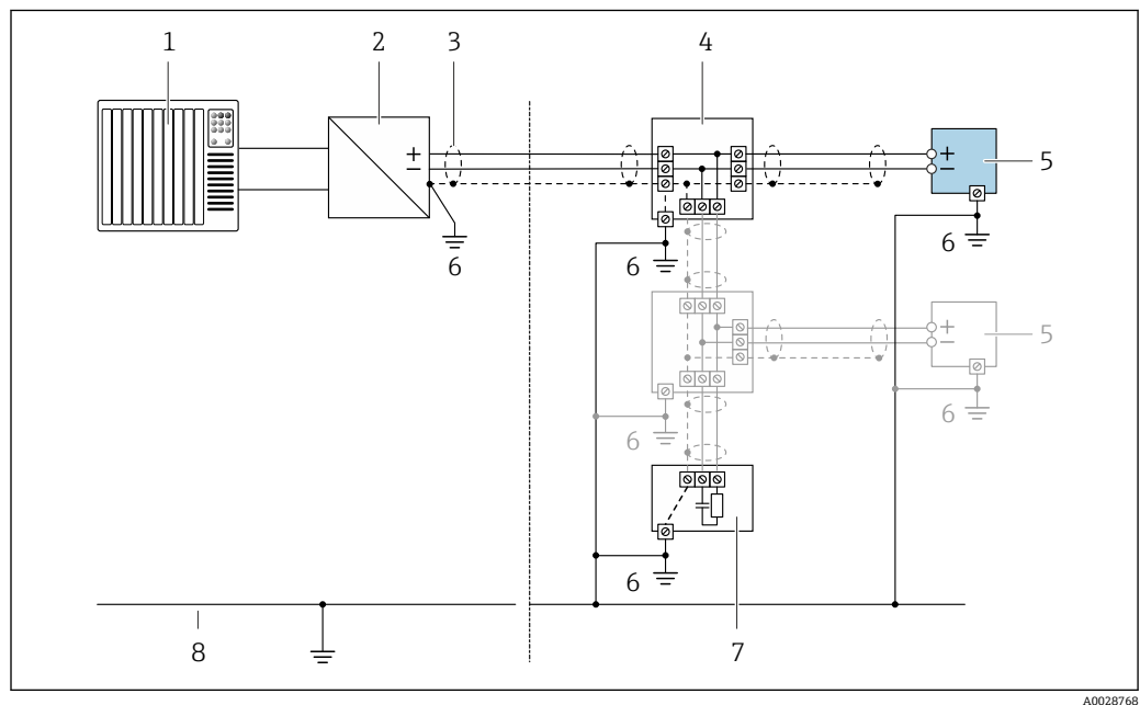
20 PROFIBUS PA 的连接实例
