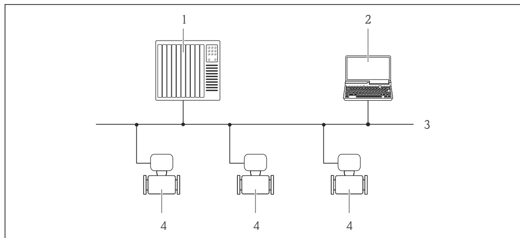
図 43 PROFIBUS DP ネットワークを介したリモート操作のオプション
