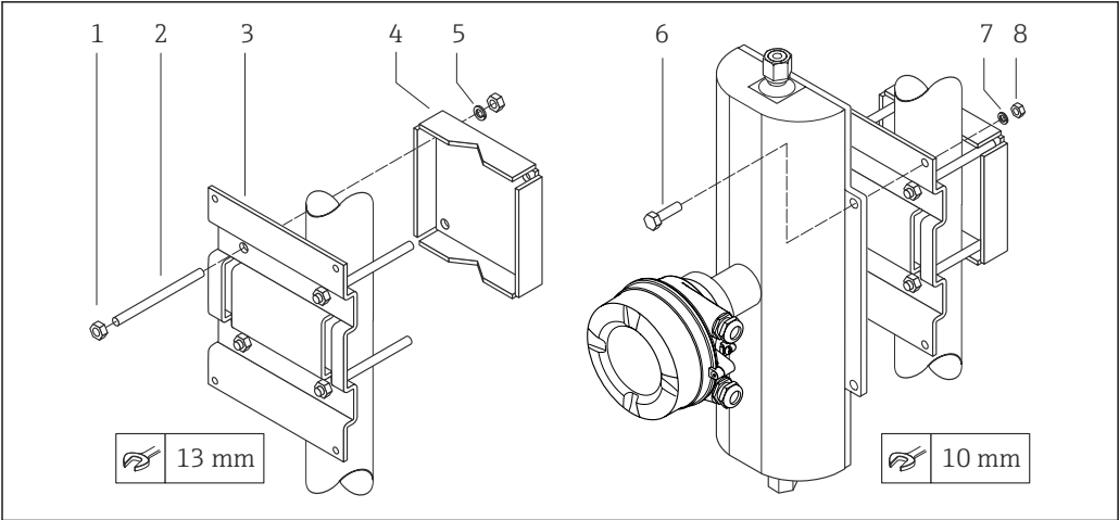
20 柱取付キット
