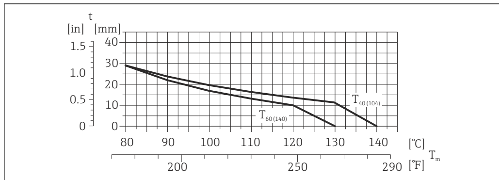
図 29 測定物の温度および周囲温度に応じた断熱材の推奨最大厚さ
