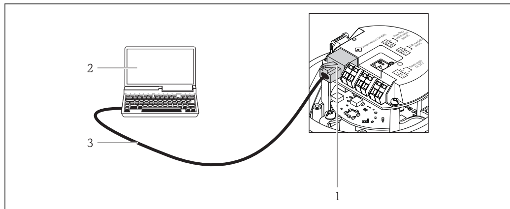
■ 46 「出力」のオーダーコードの接続、オプション B : 4~20 mA HART、パルス/周波数/スイッチ出力
