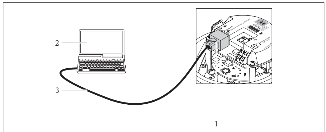
図 48 「出力」のオーダーコードの接続、オプション N : EtherNet/IP
