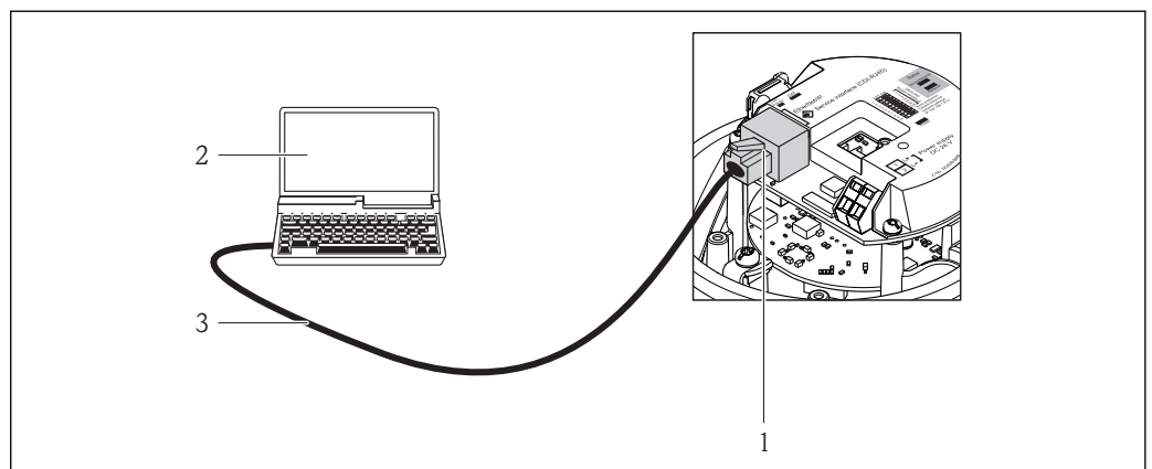
図 49 「出力」のオーダーコード、オプション R : PROFINET の接続
