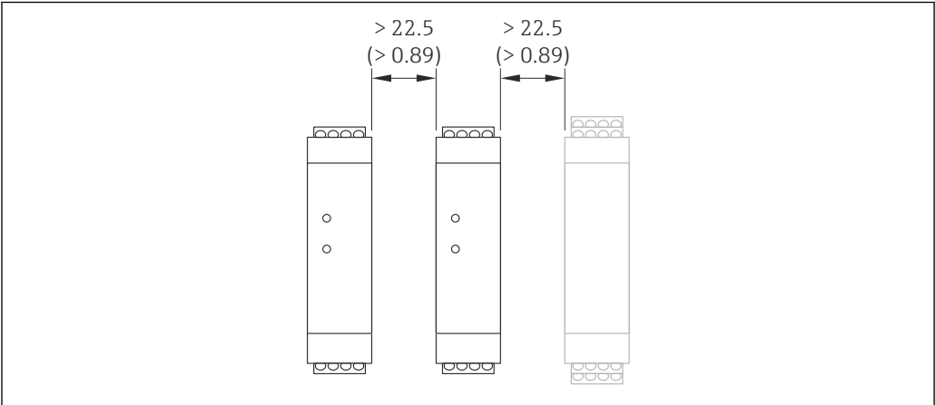
21 Promass 100 安全バリアまたはその他のモジュールとの最小距離。単位 mm (in)
