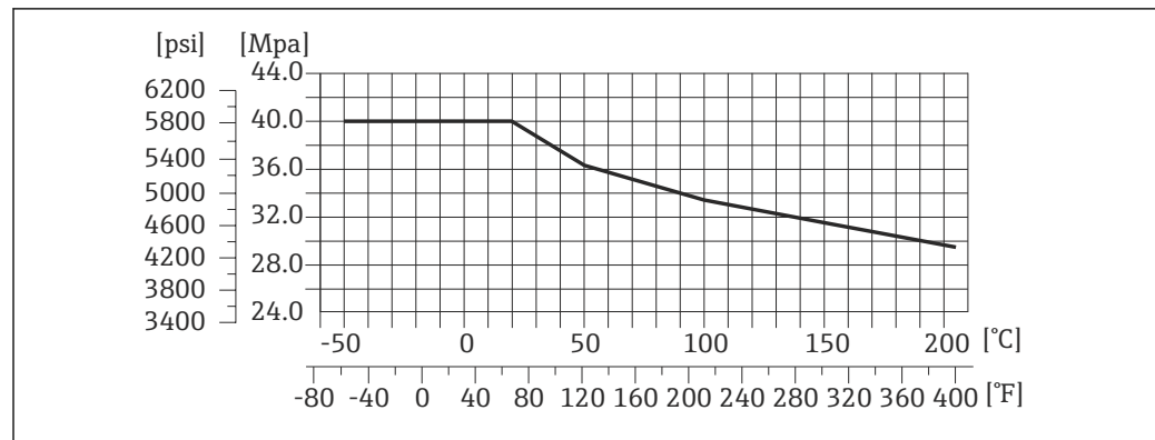
図 28 フランジ接続 4-VCO-4 カップリング : 1.4539 (SUS 890L 相当) ; ¼ NPT ネジ込み式アダプタ : 1.4539 (SUS 890L 相当)、¼" または ⅜" Swagelok カップリング : 1.4539 (SUS 890L 相当)
