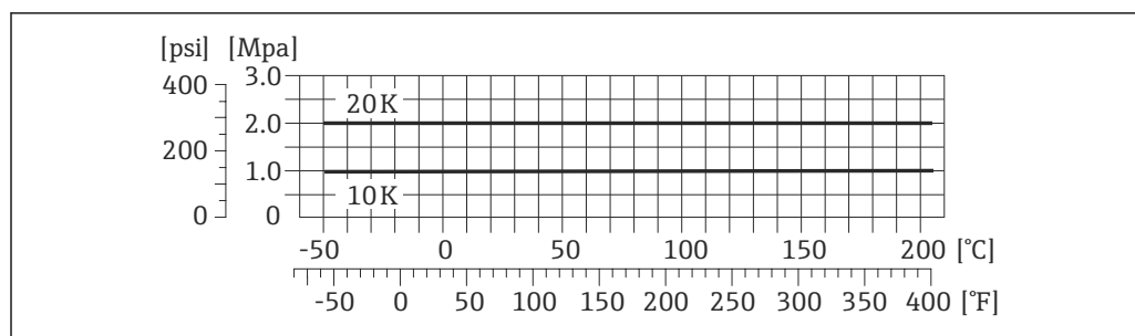
図 25 フランジ材質：1.4539 (SUS 890L 相当)、アロイ C22；ラップジョイントフランジ (非接液)：1.4404 (SUS F316L 相当)
