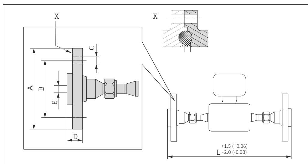
図 33 単位 mm (in)
