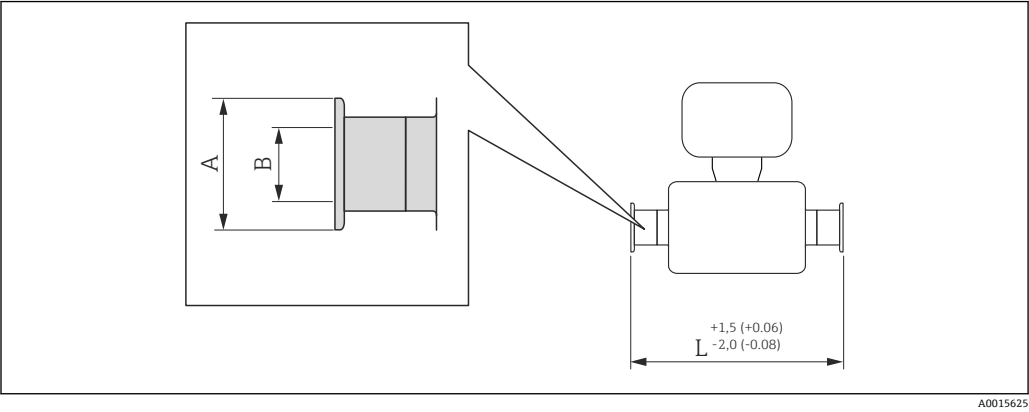
37 単位 mm (in)
