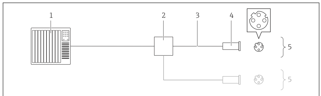
■ 15 EtherNet/IP の接続例
