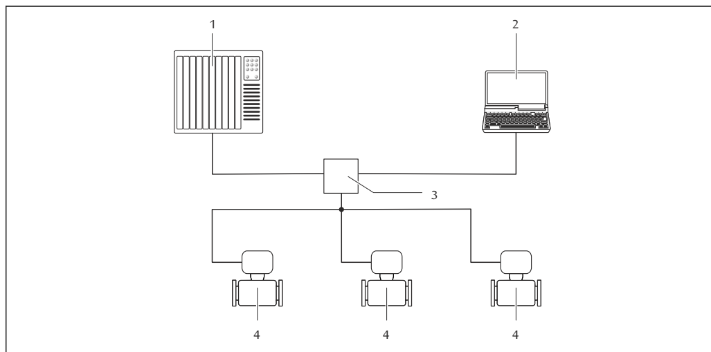
図 45 PROFINET ネットワーク経由のリモート操作オプション
