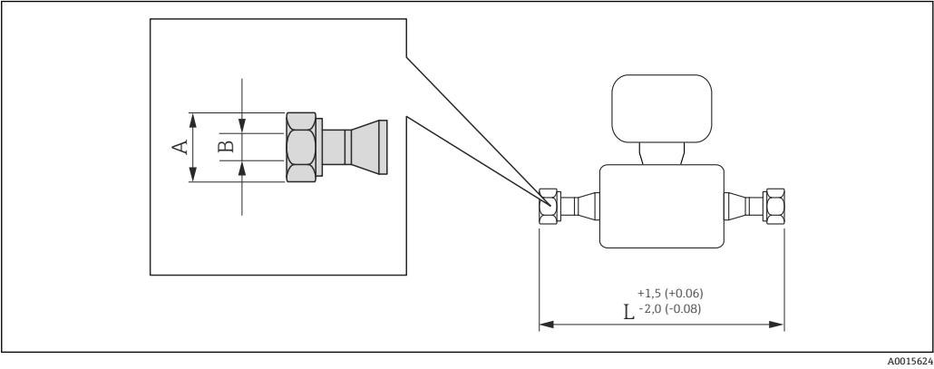
36 単位 mm (in)
