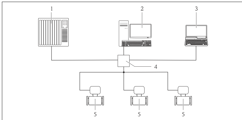
図 44 Ethernet ベースのフィールドバス経由のリモート操作オプション
