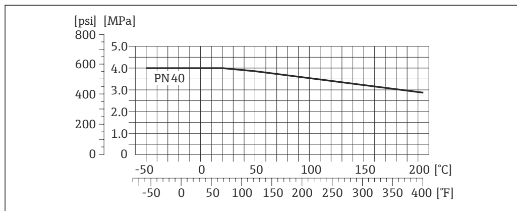
図 23 フランジ材質：1.4539 (SUS 890L 相当)、アロイ C22；ラップジョイントフランジ (非接液)：1.4404 (SUS F316 または F316L 相当)
