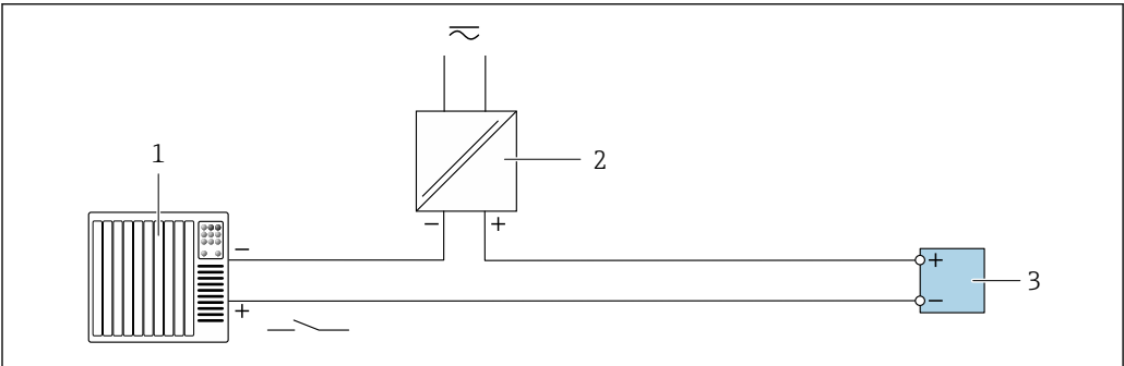
图 13 状态输入的连接实例
