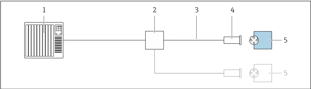
图 12 工业以太网(EtherNet/IP)的连接实例
