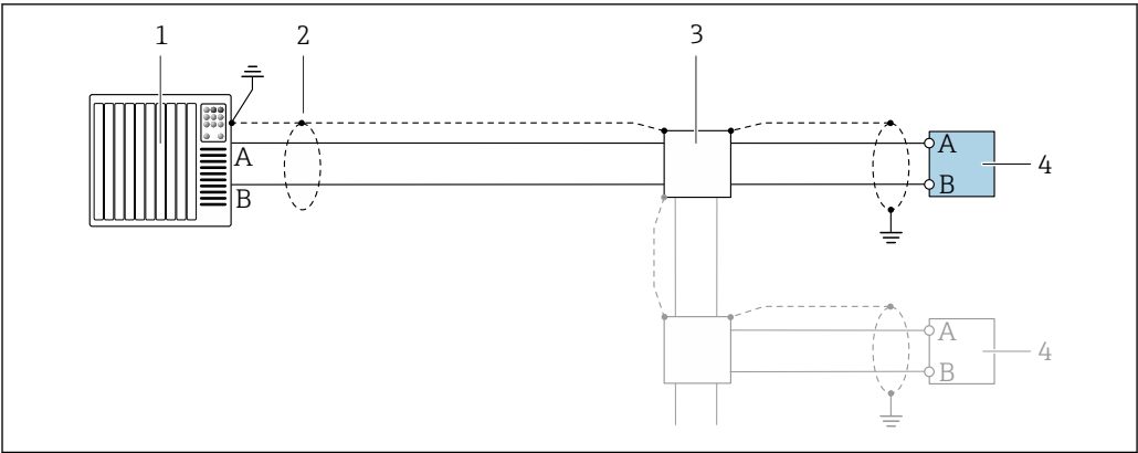
图 11 Modbus RS485 的连接示例，在非危险区和 2 区 / Div. 2 防爆场合中
