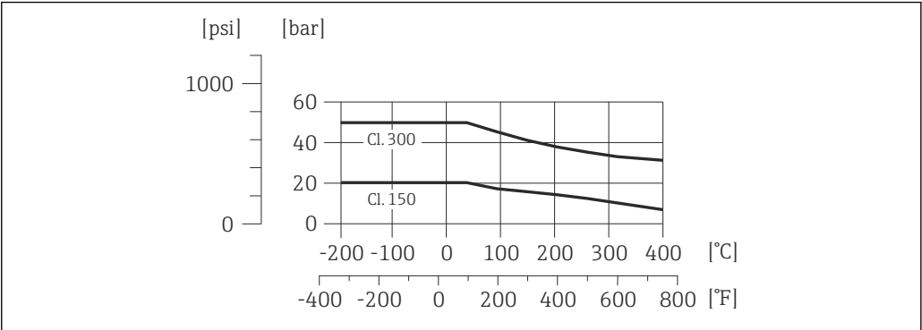
18 Werkstoff Prozessanschluss: Rostfreier Stahl, mehrfachzertifiziert, 1.4404 (F316, F316L)
