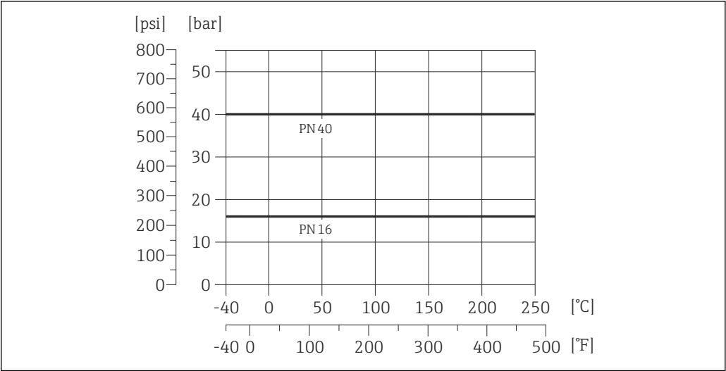
17 Werkstoff Prozessanschluss: Guss CX2MW ähnlich zu Alloy C22/2.4602
