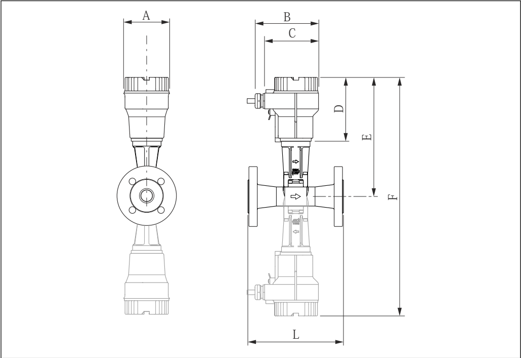
26 Gestrichelt: Dualsensausführung
