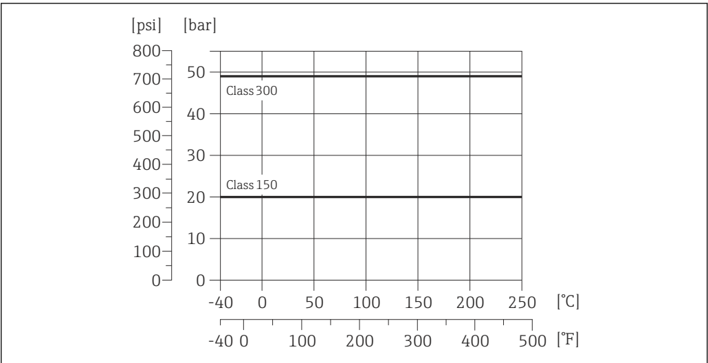
19 Werkstoff Prozessanschluss: Guss CX2MW ähnlich zu Alloy C22/2.4602
