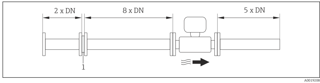
1 Strömungsgleichrichter
