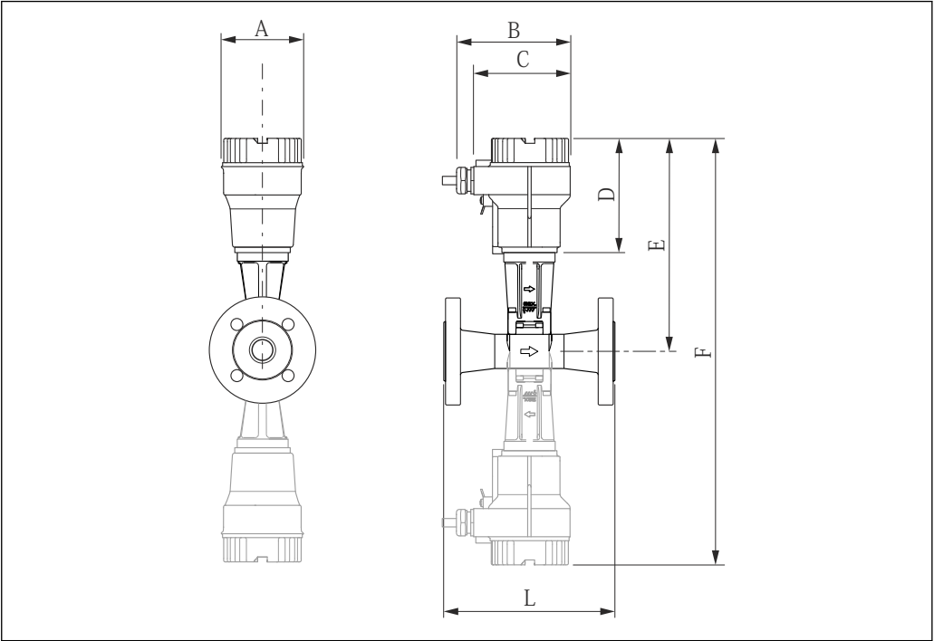
23 Gestrichelt: Dualsensausführung
