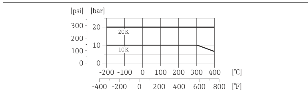
20 Werkstoff Prozessanschluss: Rostfreier Stahl, mehrfachzertifiziert, 1.4404 (F316, F316L)
