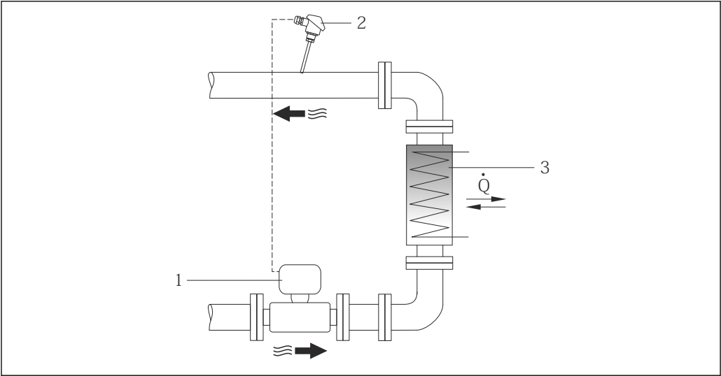
15 Aufbau zur Wärmedifferenzmessung von Sattedampf und Wasser
