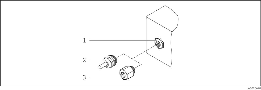
28 Mögliche Kabeleinführungen/-verschraubungen
