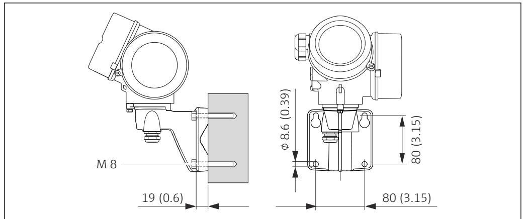
13 Maßeinheit mm (in)
