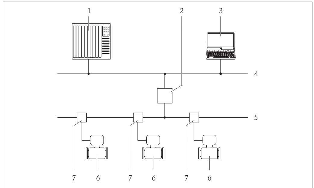
31 Möglichkeiten der Fernbedienung via PROFIBUS PA Netzwerk
