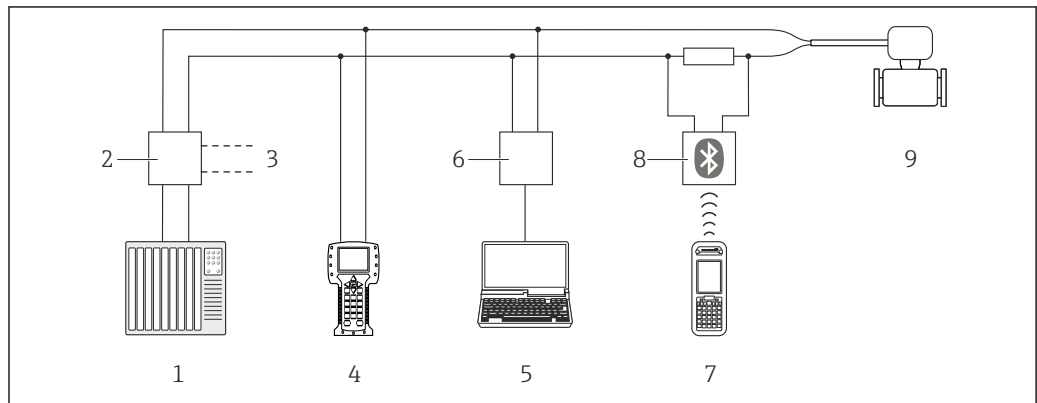
30 Möglichkeiten der Fernbedienung via HART-Protokoll
