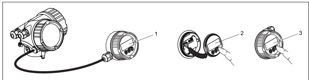
29 Bedienmöglichkeiten über FHX50
