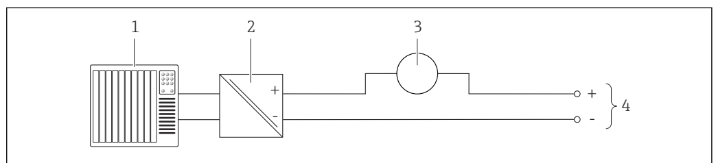
10 Anschlussbeispiel für 4-20 mA Stromeingang
