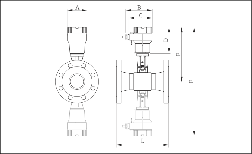
21 Gestrichelt: Dualsensausführung
