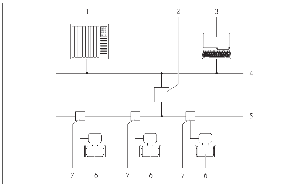
32 Möglichkeiten der Fernbedienung via PROFIBUS PA Netzwerk
