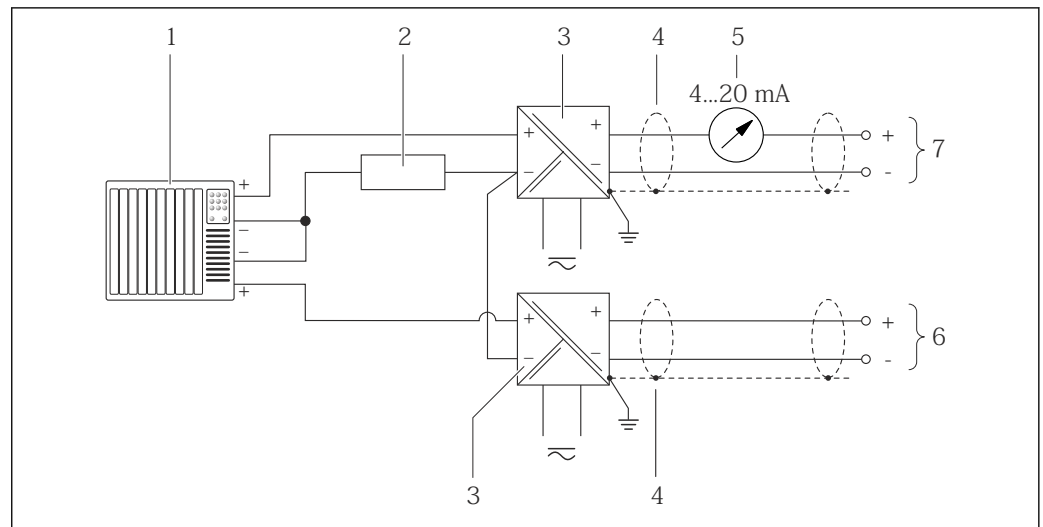
11 Anschlussbeispiel für HART-Eingang mit gemeinsamem "Minus"
