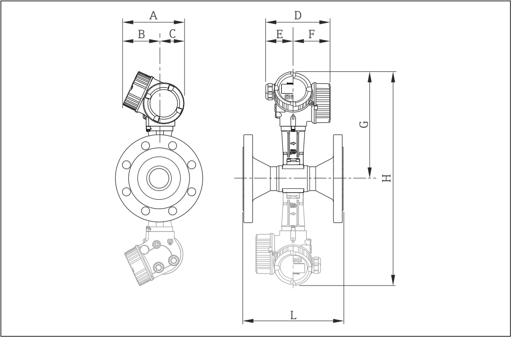
25 Gestrichelt: Dualsensausführung
