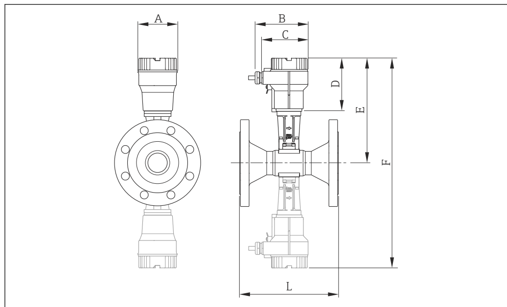
22 Gestrichelt: Dualsensausführung
