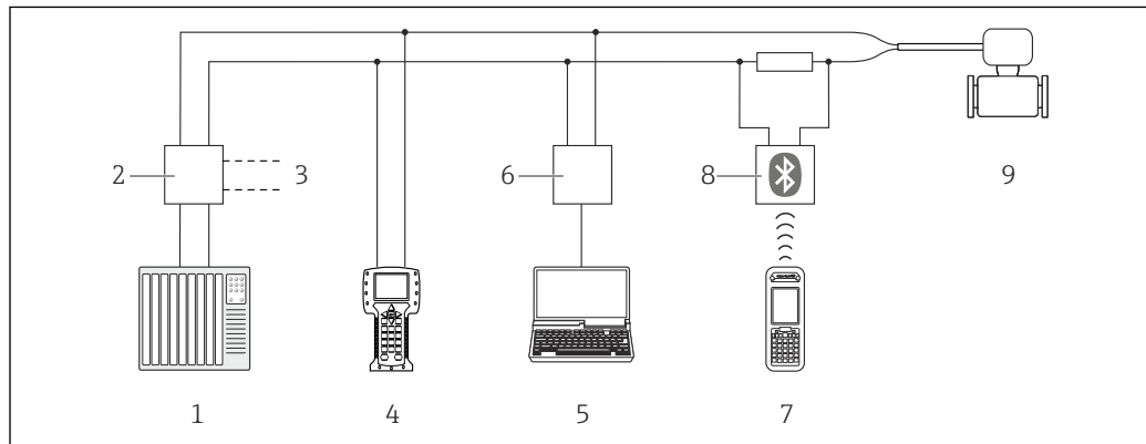
31 Möglichkeiten der Fernbedienung via HART-Protokoll
