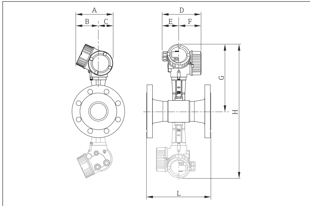
24 Gestrichelt: Dualsensausführung
