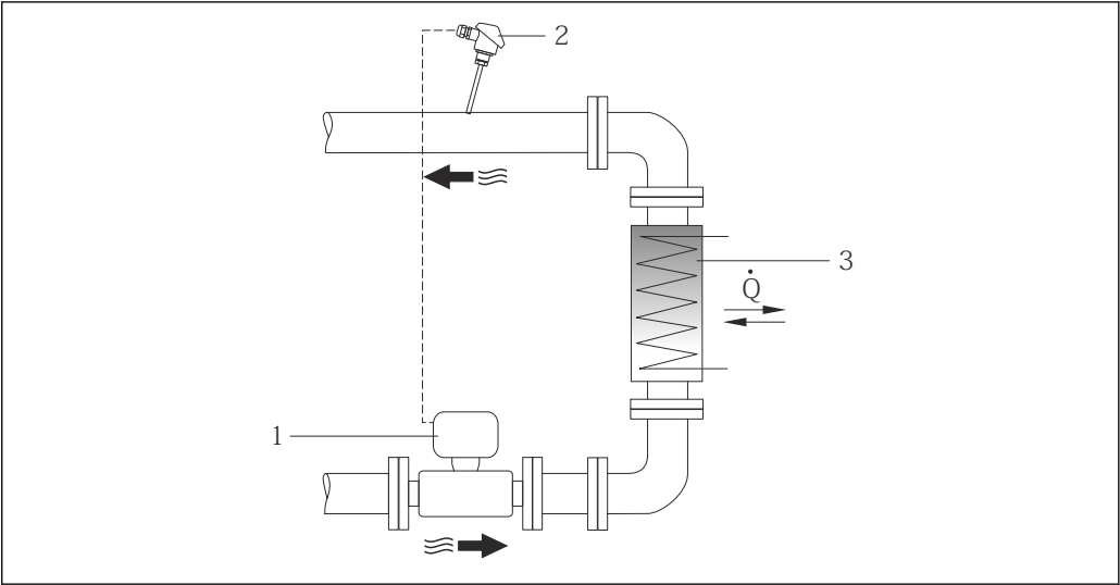
15 Aufbau zur Wärmedifferenzmessung von Sattdampf und Wasser
