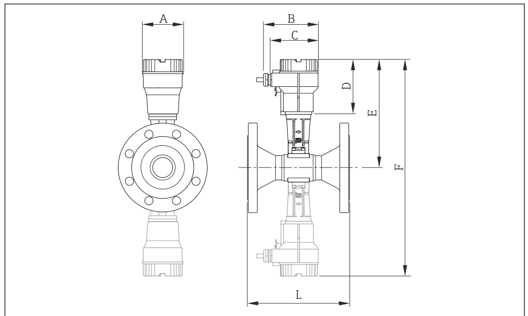
27 Gestrichelt: Dualsensausführung
