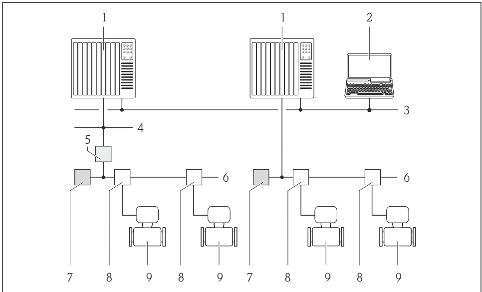
12 Möglichkeiten der Fernbedienung via FOUNDATION Fieldbus Netzwerk
