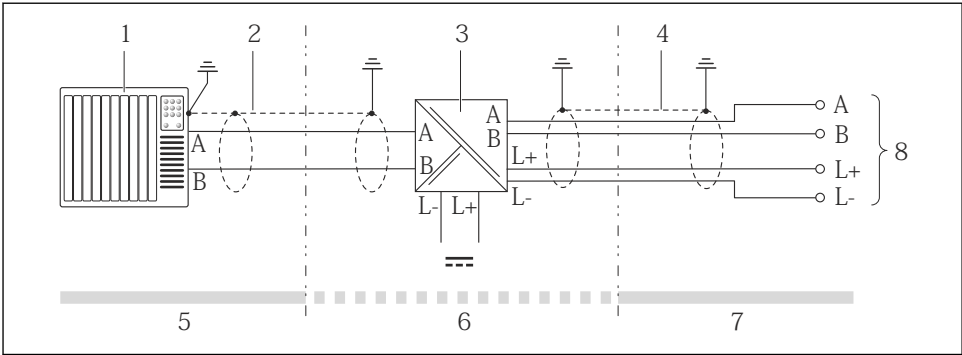
13 Raccordement électrique entre le transmetteur et la barrière de sécurité Promass 100
