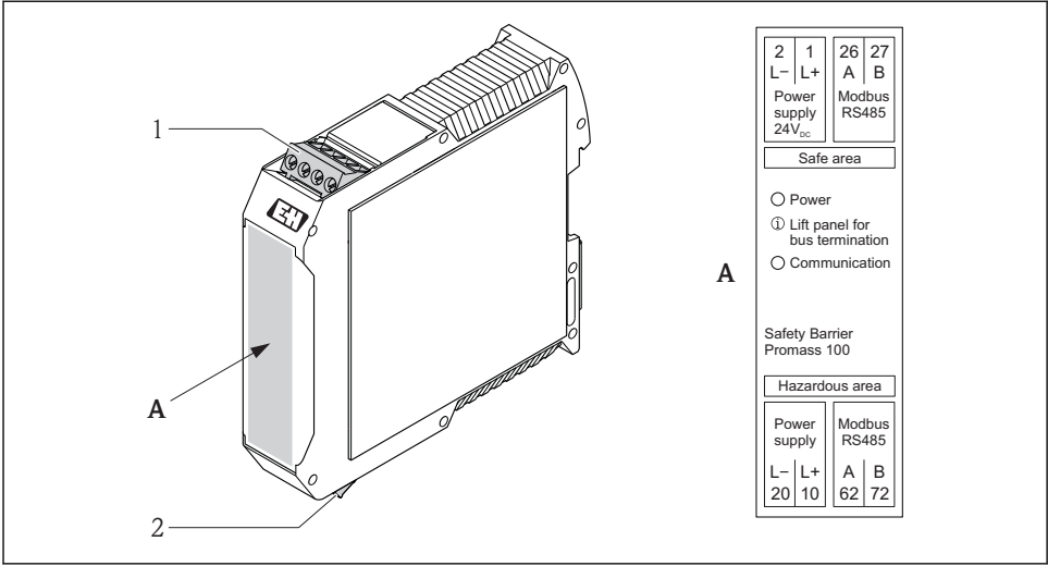
10 Barrière de sécurité Promass 100 avec raccordements
