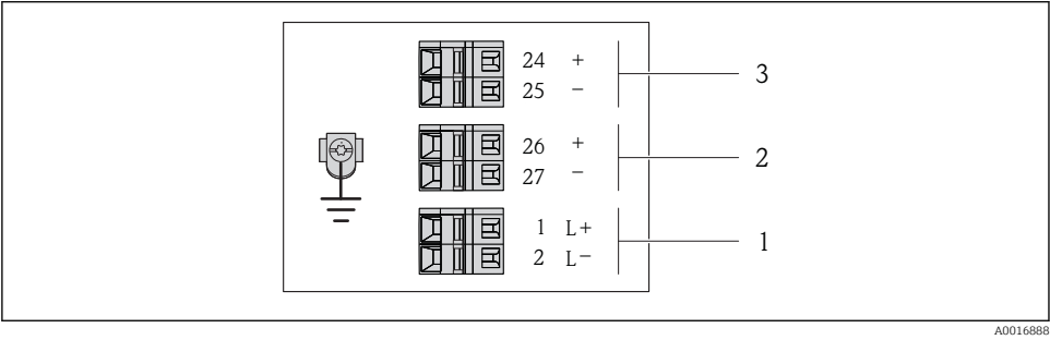
5 Occupation des bornes 4-20 mA HART avec sortie impulsion/fréquence/tor
