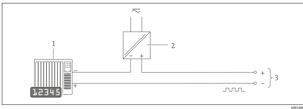
图 5 脉冲/频率输出(无源信号)的连接实例
