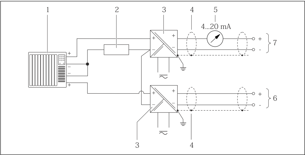
图 10 HART 输入(共用负信号端)的连接示意图
