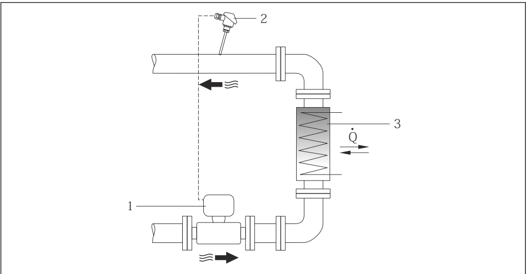
15 饱和蒸汽和水的温差测量的系统布局示意图
