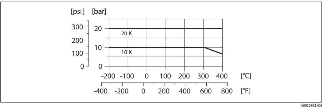
18 过程连接材料：不锈钢，铸钢，多项认证，1.4408 (CF3M)
