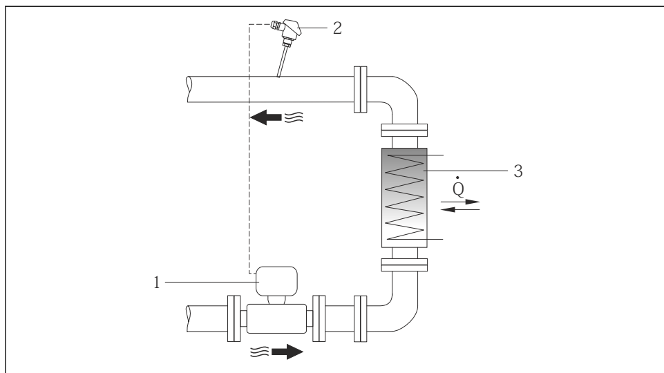
3 Disposición para medidas de diferencias delta de temperatura en vapor saturado o en agua
