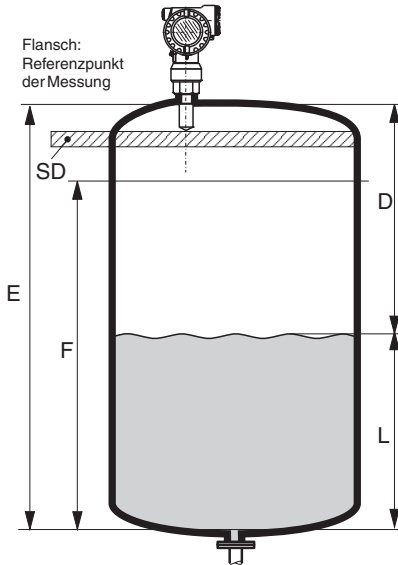
Füllstandmessung in Flüssigkeiten
