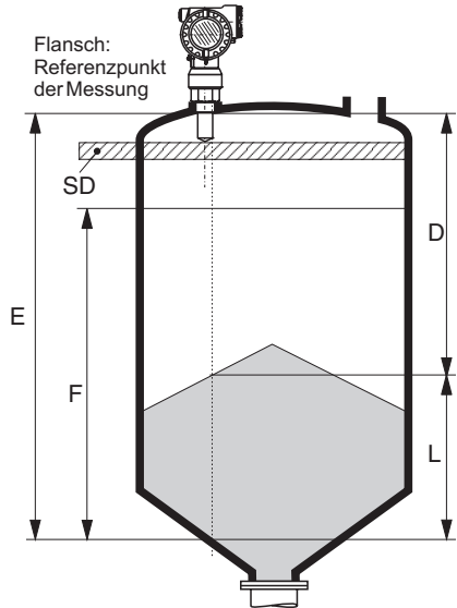
Füllstandmessung in Schüttgütern
