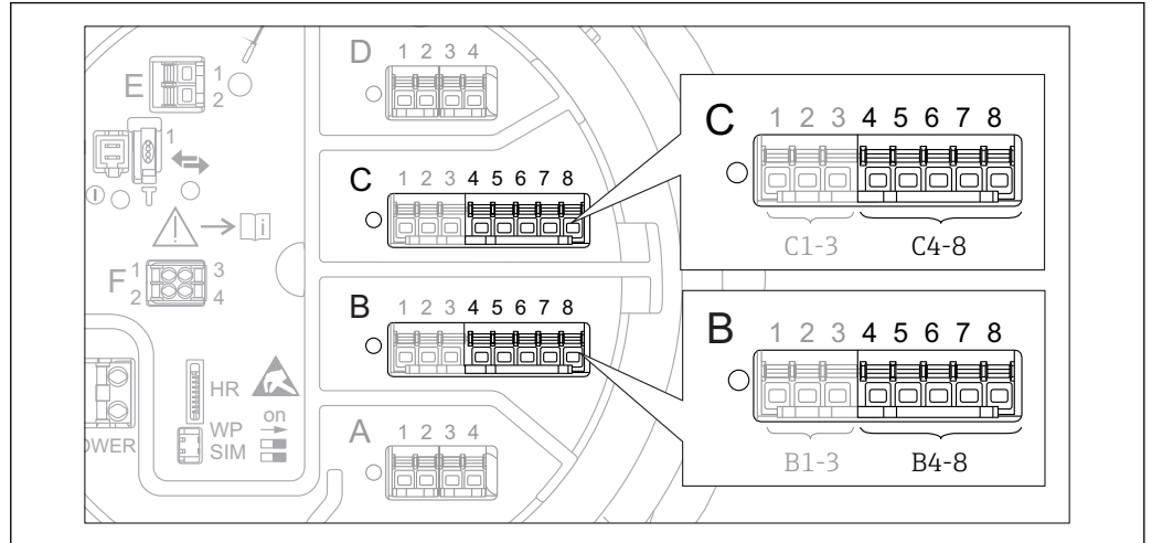
図 4 「Analog IP」 サブメニュー用端子 (それぞれ「B4-8」または「C4-8」)
