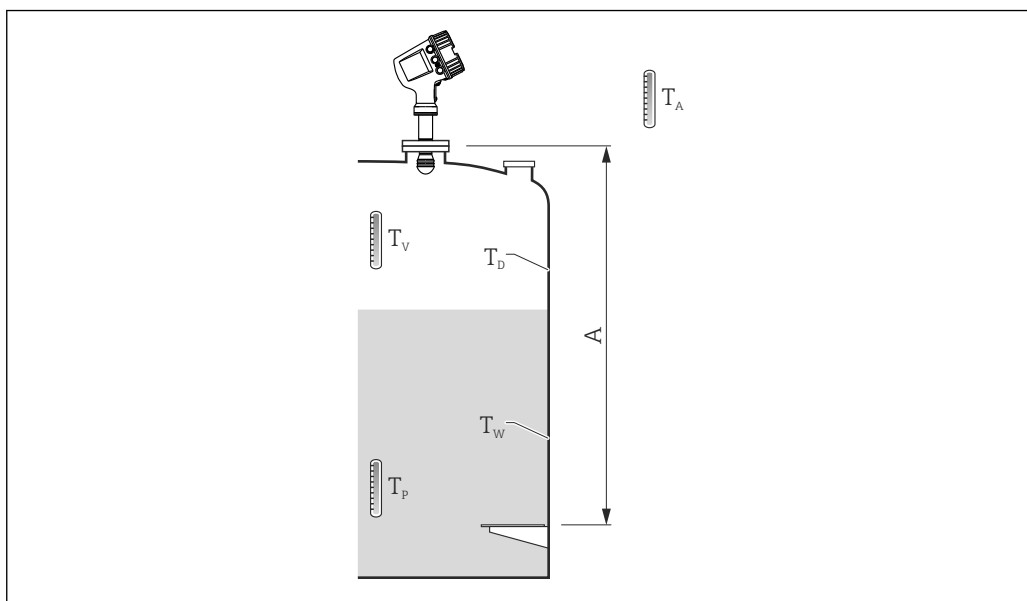
図 12 CTSh 演算用パラメータ
