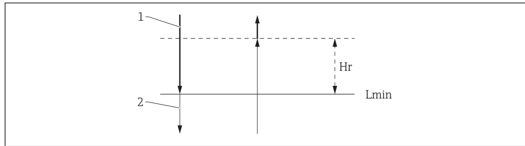
図 14 HTMS ヒステリシス
