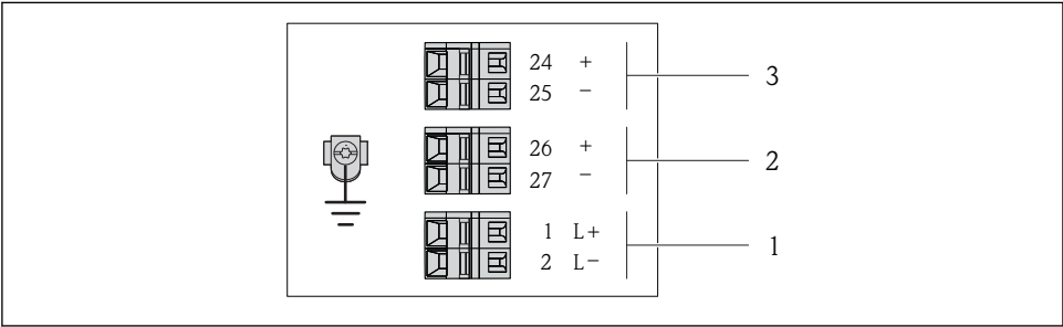
4 Occupation des bornes 4-20 mA HART avec sortie impulsion/fréquence/tor
