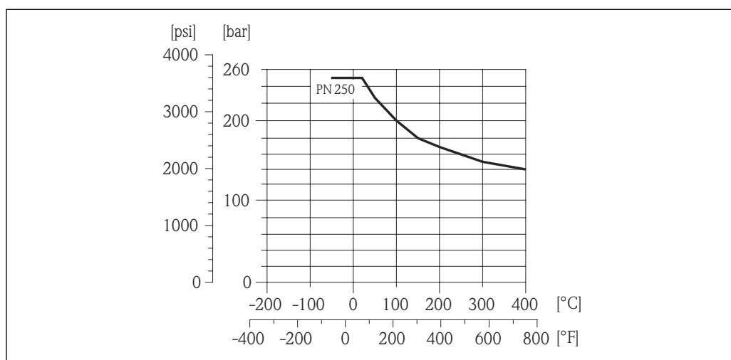
18 Materiał przyłącza: stal k.o. 1.4571, podobna do F316 Ti
