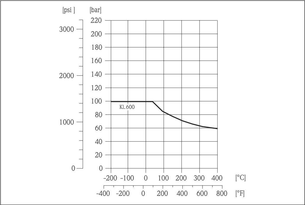
19 Materiał przyłącza: staliwo k.o., międzynarodowe dopuszczenia, 1.4408 (CF3M)
