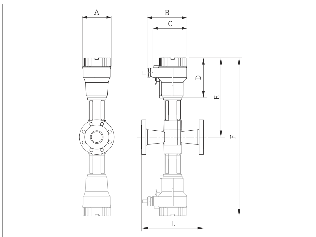
■ 24 Szarą linią przerywaną oznaczono wersję z dwoma niezależnymi czujnikami i przetwornikami
