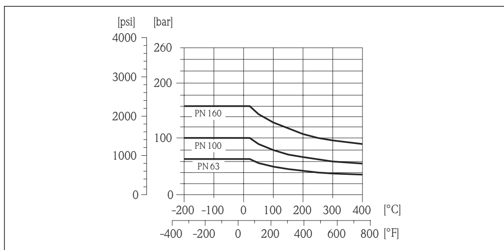
17 Materiał przyłącza: staliwo k.o., międzynarodowe dopuszczenia, 1.4408 (CF3M)
