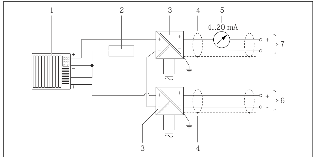
☒ 13 Exemple de raccordement pour entrée HART avec "moins" commun
