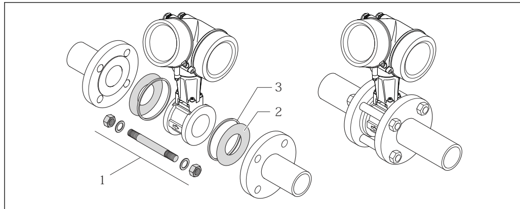
8 Set de montage version entre brides
