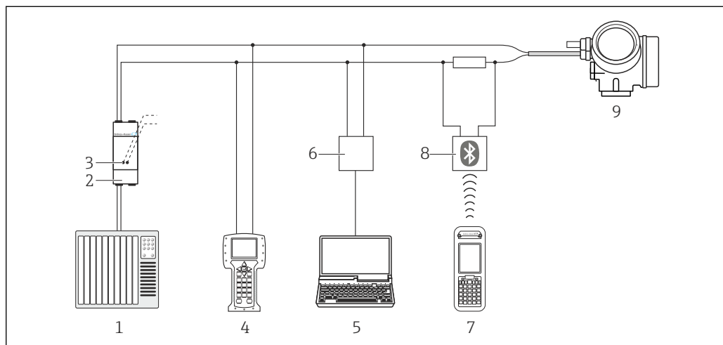
図 34 HART 経由のリモート操作用オプション
