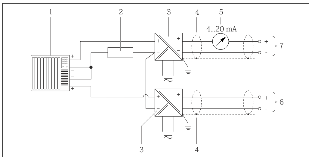
図 12 HART 入力（マイナスコモン）の接続例
