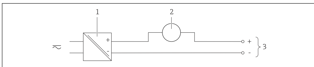
図 11 4~20 mA 電流入力の接続例
