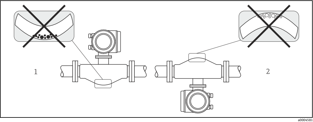
水平管道上的安装示意图
