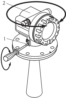
F12/F23外壳
