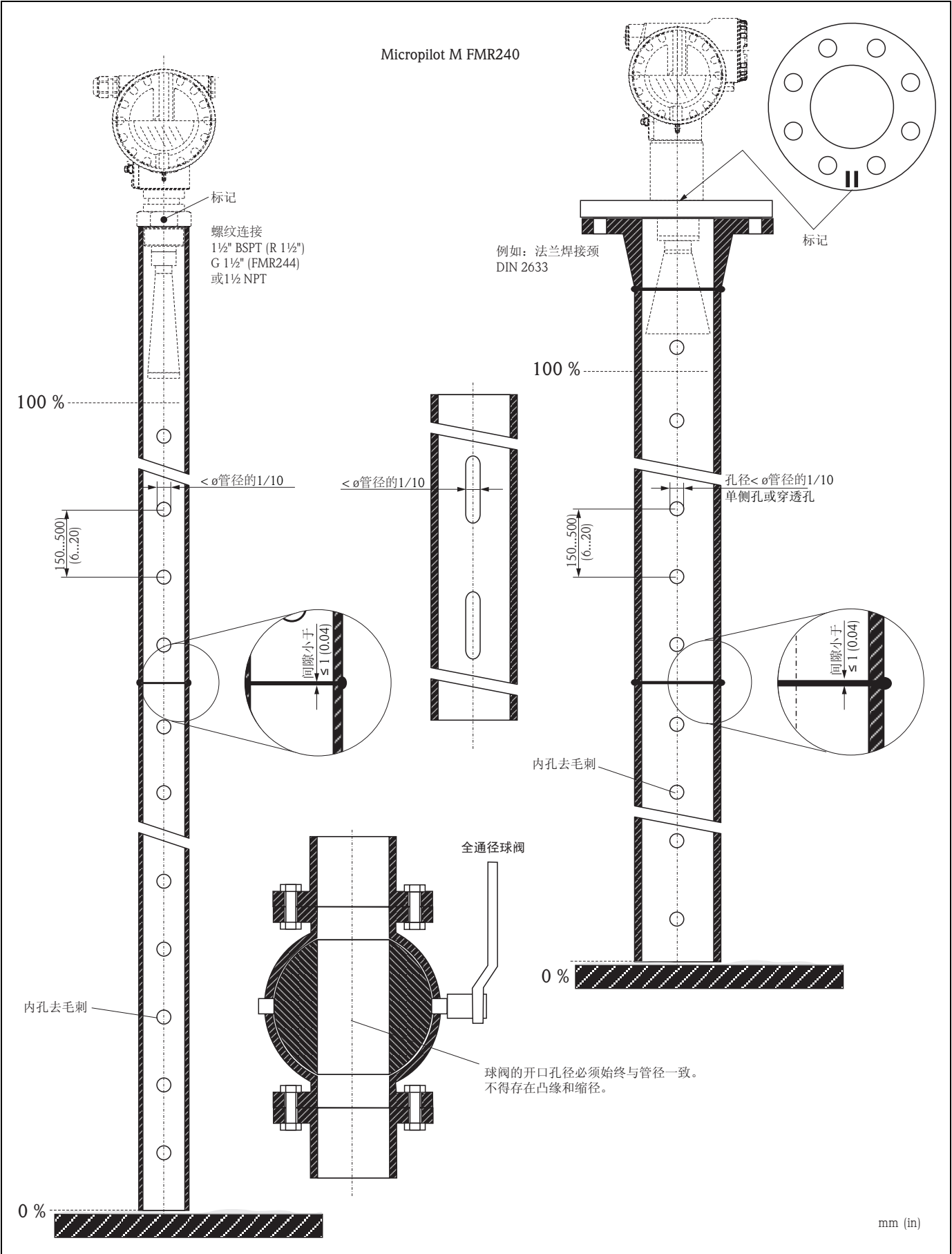
导波管的结构示意图
