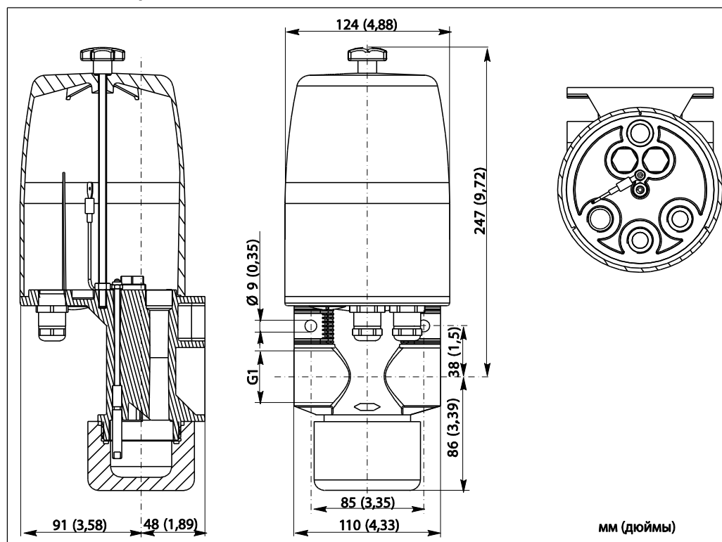
Рис. 3. Размеры
