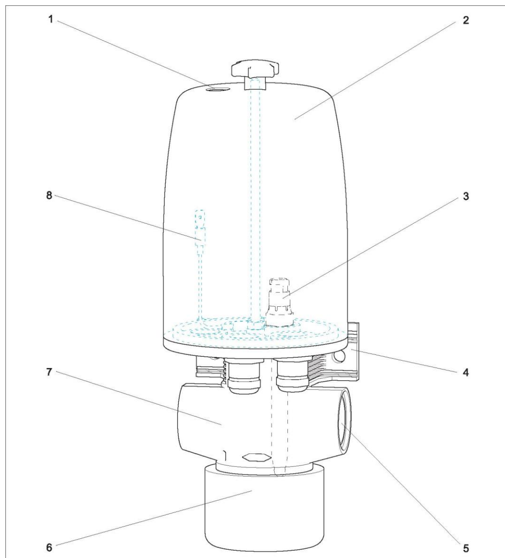
Рис. 1. Арматура CPA250 с датчиком
