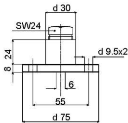
Рис. 2. Компрессионный фитинг TA 60 с фланцем Кабельные уплотнители PTFE или AISI 316
