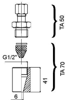
Рис. 3. Приварной гигиенический фитинг TA 70 для использования с TA 50
