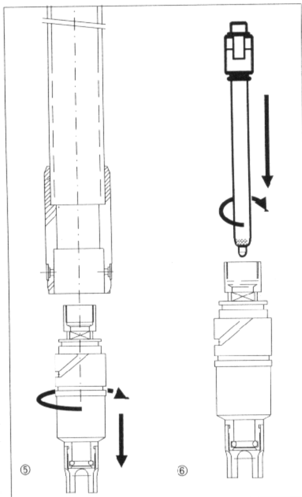
Obr. 6 : Montáž elektrody pH / redox
