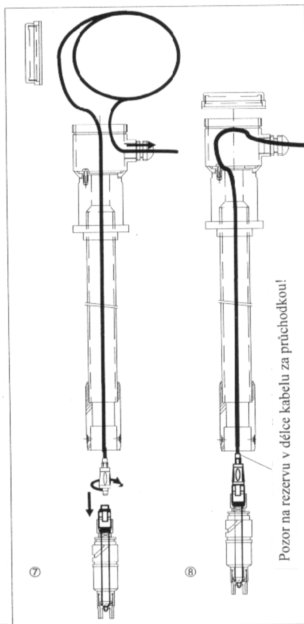
Obr. 7 : Montáž měřicího kabelu s konektorem
