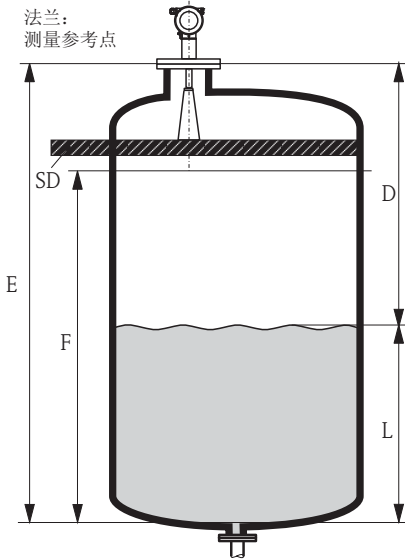
液位测量
