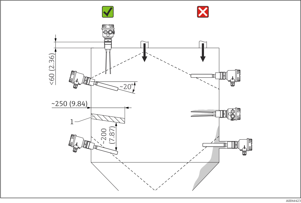
Unità di misura mm (in) 1 Tettuccio di protezione (fornito dal cliente)
