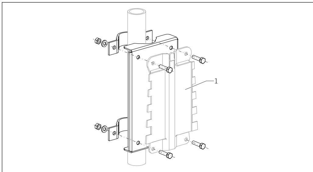
図 13 ポリカーボネート製フィールドハウジング用の取付プレート
