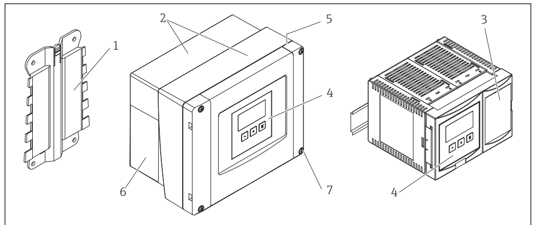
図 8 ポリカーボネート製フィールドハウジングと DIN レールハウジングの構成品
