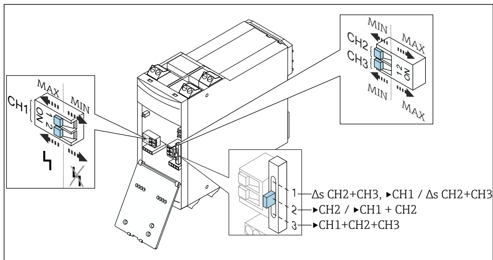
図 13 機能設定用のスイッチ
