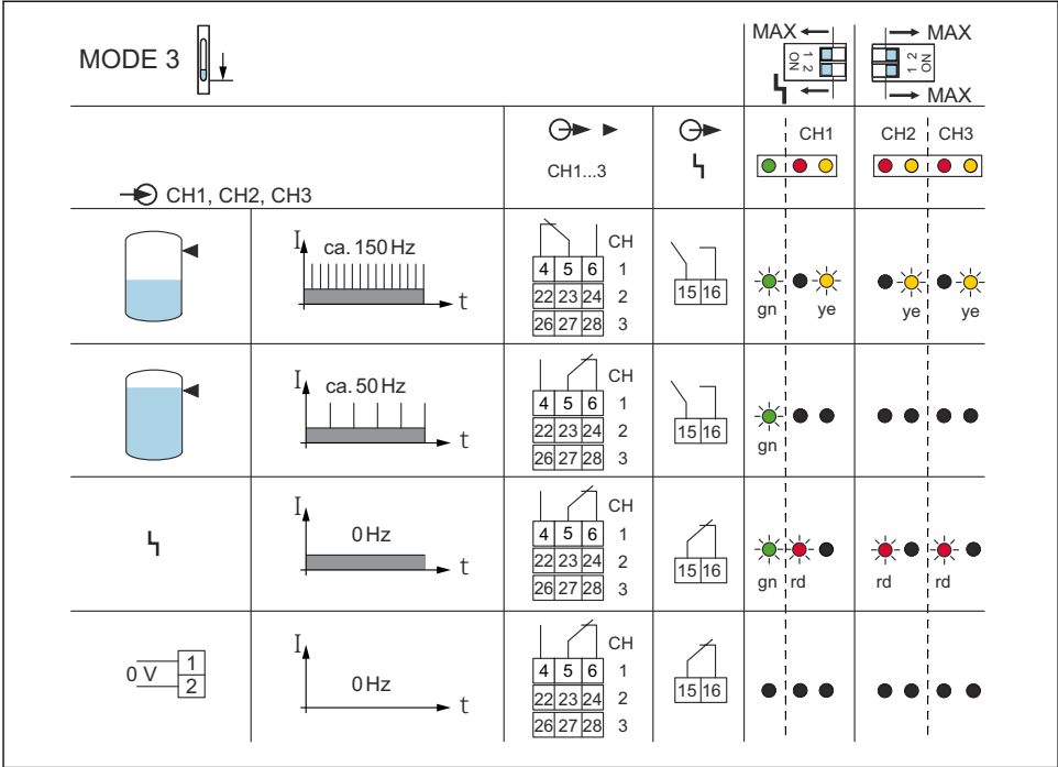
図 18 スイッチング動作および信号伝達
