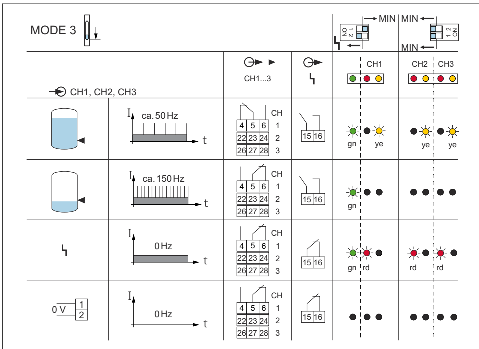
図 19 スイッチング動作および信号伝達
