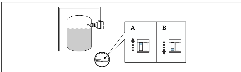
図 15 エレクトロニックインサート (FEL57) のスイッチ位置
