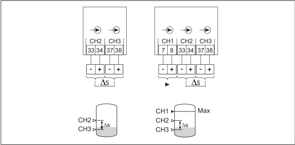
図 8 2 点制御 \Delta s 用のセンサの接続
