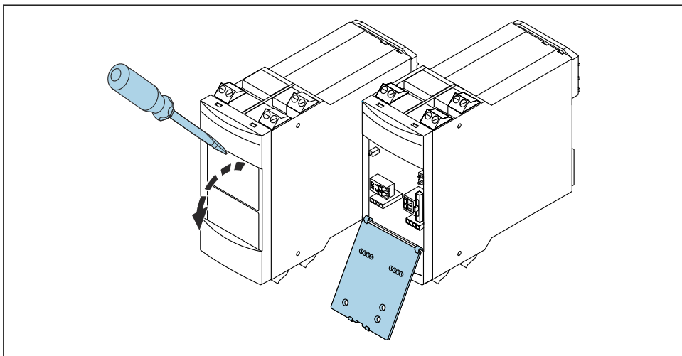
10 フロントパネルの開放
