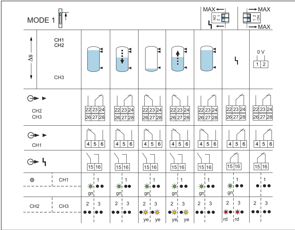
図 20 スwitching動作および信号伝達
