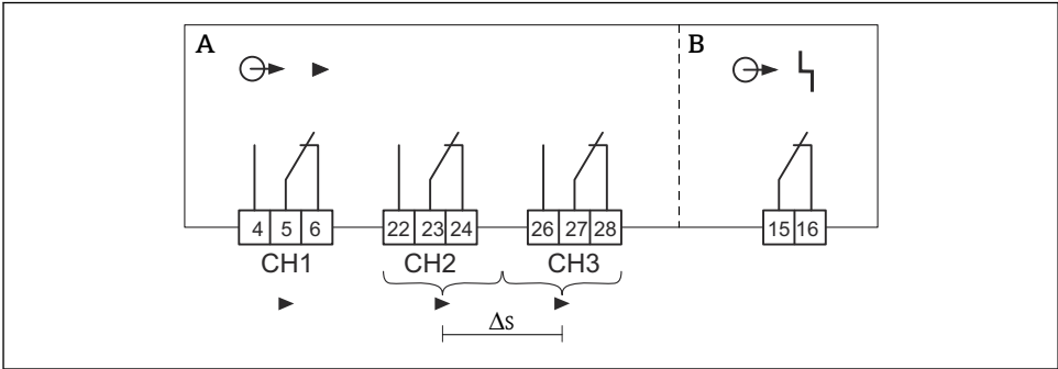
図 9 出力の接続
