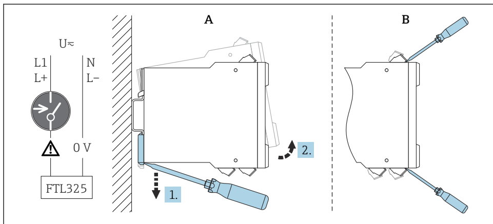
図 5 取外し
