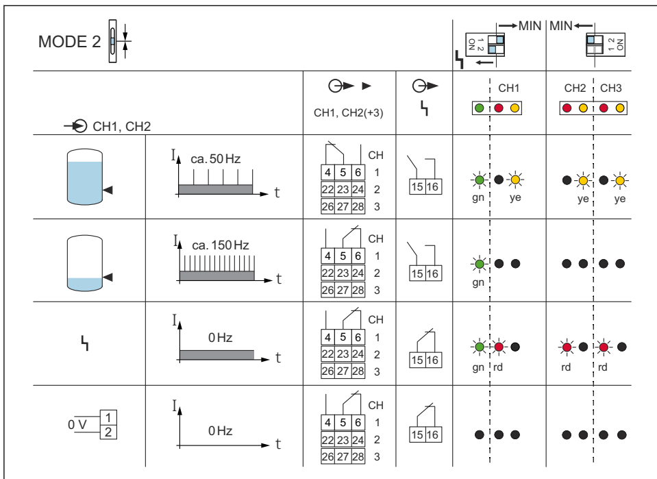
図 17 スイッチング動作および信号伝達
