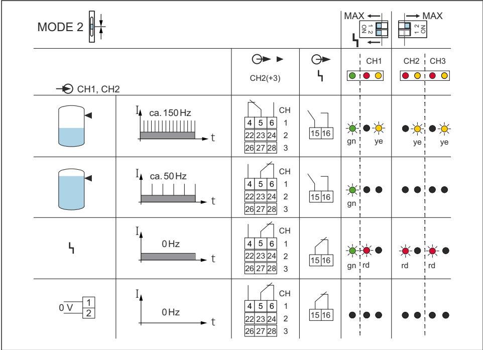
図 16 スイッチング動作および信号伝達
