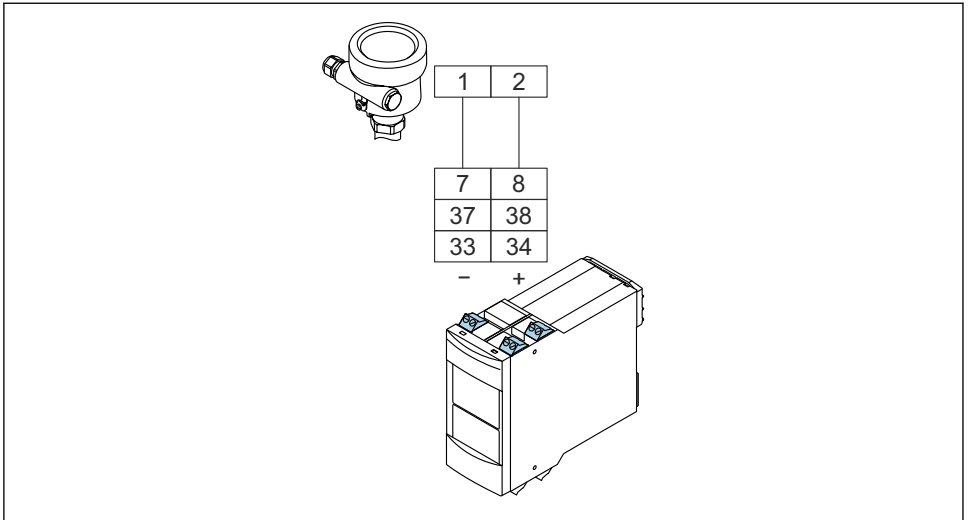
7 センサと Nivotester の接続
