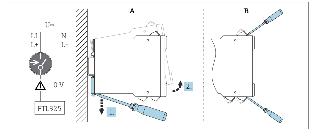
図 6 取外し
