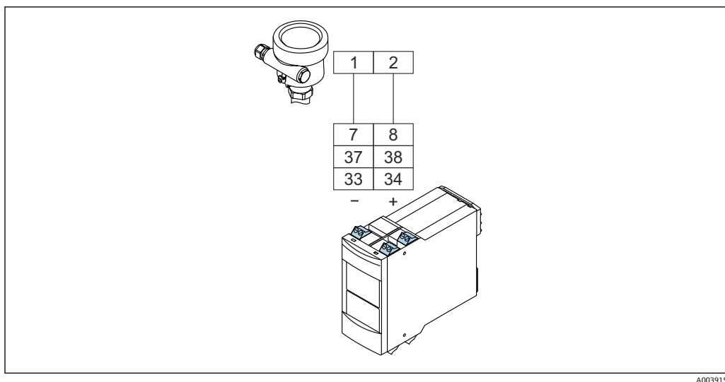
図 8 センサと Nivotester の接続
