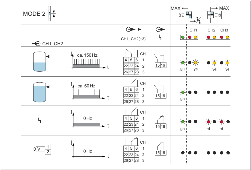
図 20 スwitching動作および信号伝達
