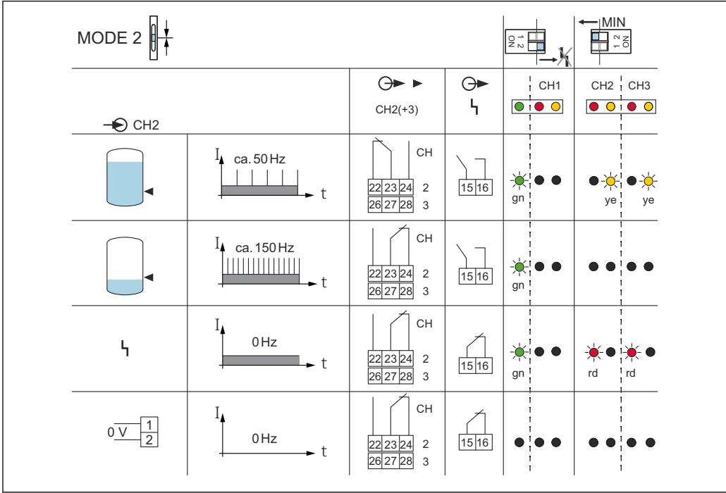
図 18 スイッチング動作および信号伝達
