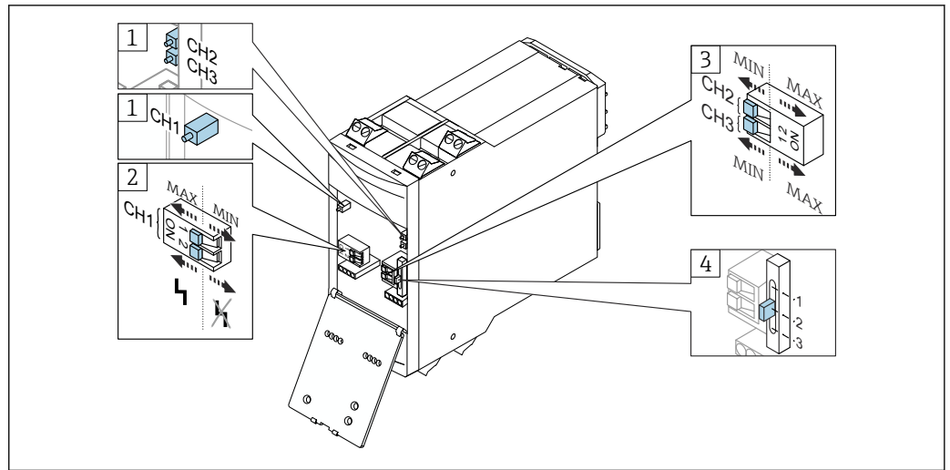
図 13 操作部
