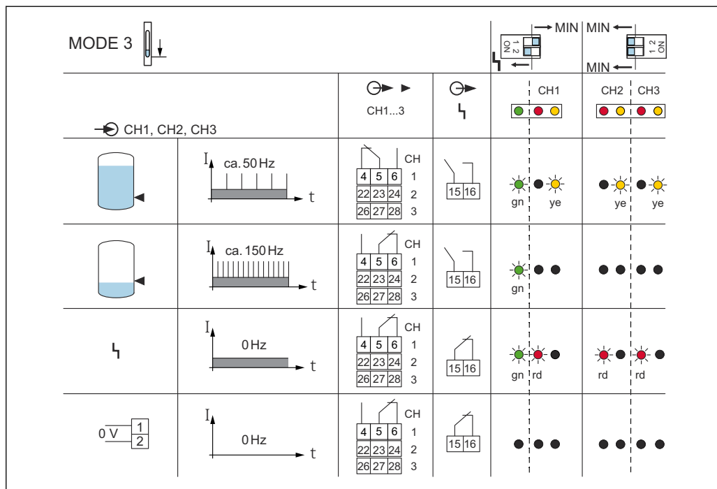
図 25 スイッチング動作および信号伝達
