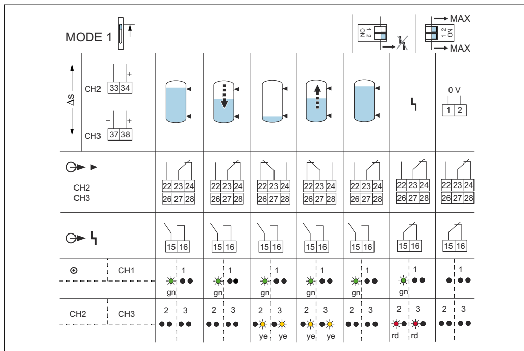
図 27 スイッチング動作および信号伝達
