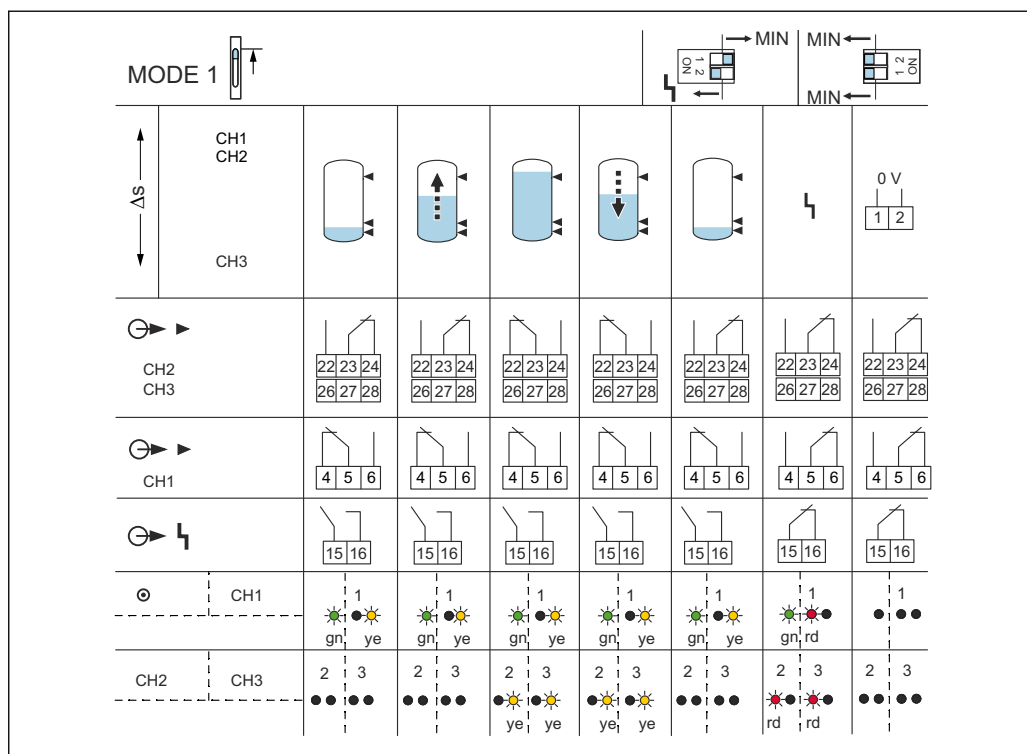
図 31 スイッチング動作および信号伝達
