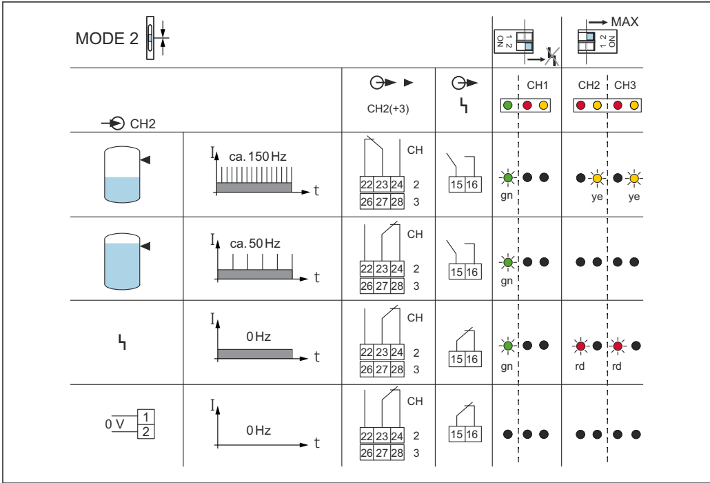
図 17 スイッチング動作および信号伝達
