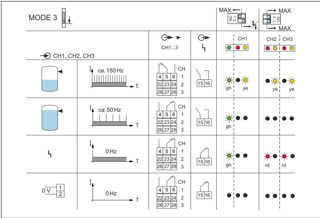
図 24 スイッチング動作および信号伝達
