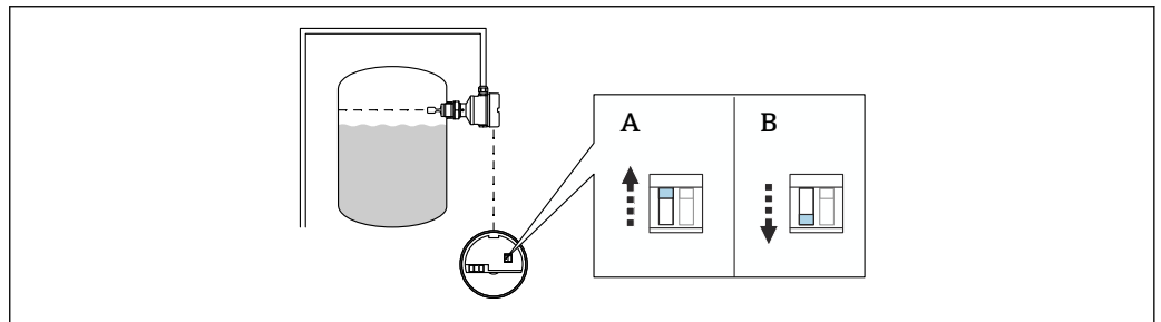
図 16 エレクトロニックインサート (FEL57) のスイッチ位置
