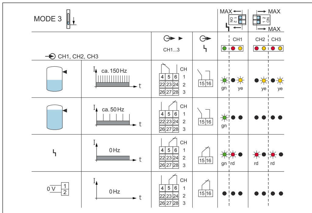
図 23 スイッチング動作および信号伝達
