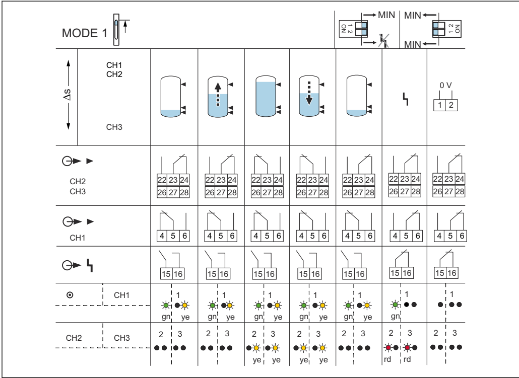
図 32 スイッチング動作および信号伝達
