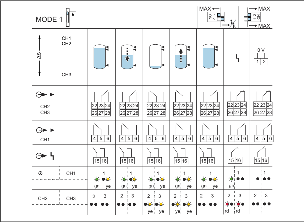
図 30 スイッチング動作および信号伝達
