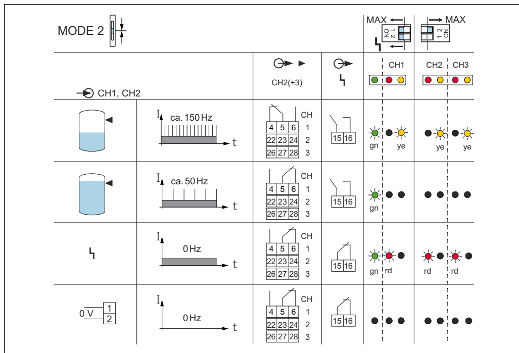
図 19 スイッチング動作および信号伝達
