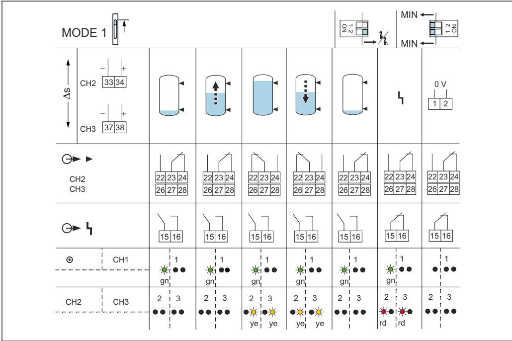
図 28 スイッチング動作および信号伝達
