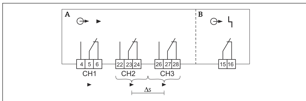
図 10 出力の接続
