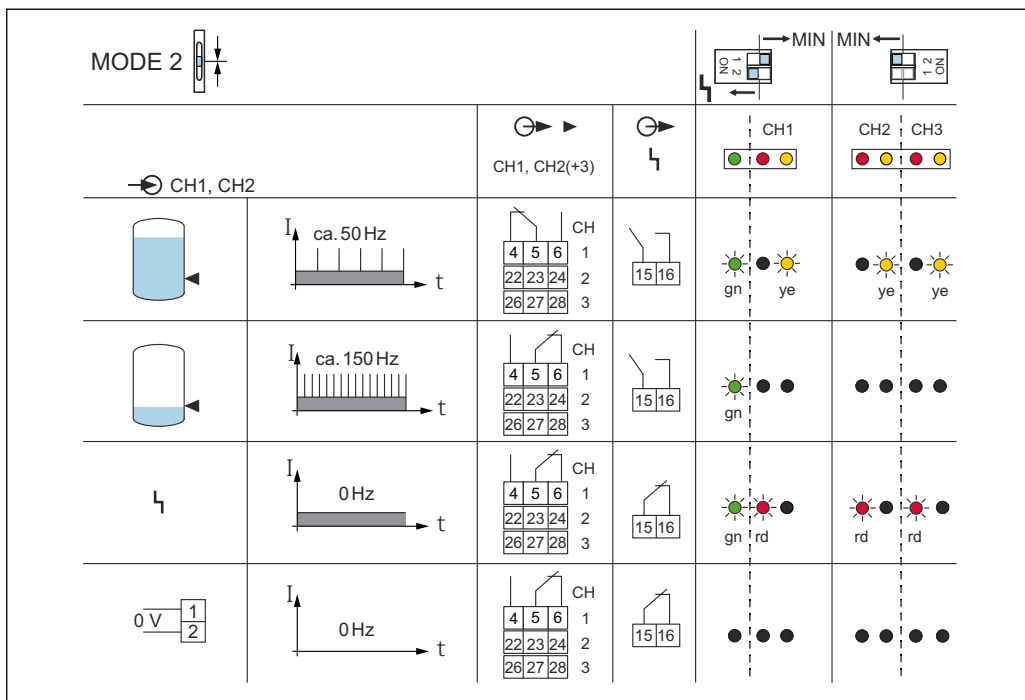
図 21 スイッチング動作および信号伝達
