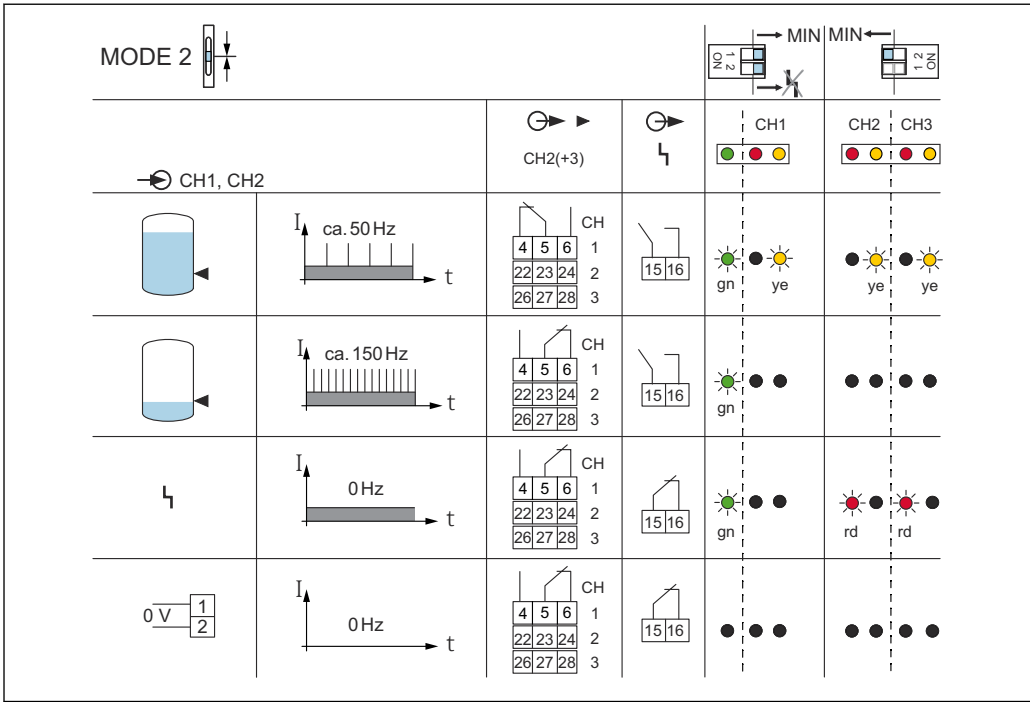
図 22 スイッチング動作および信号伝達
