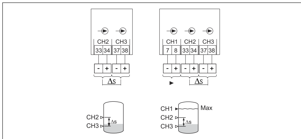
図 9 2 点制御 \Delta s 用のセンサの接続
