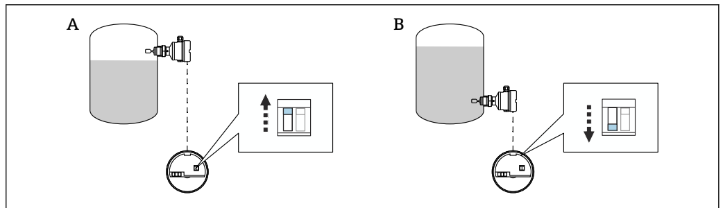
図 15 エレクトロニックインサート (FEL67) のスイッチ位置
