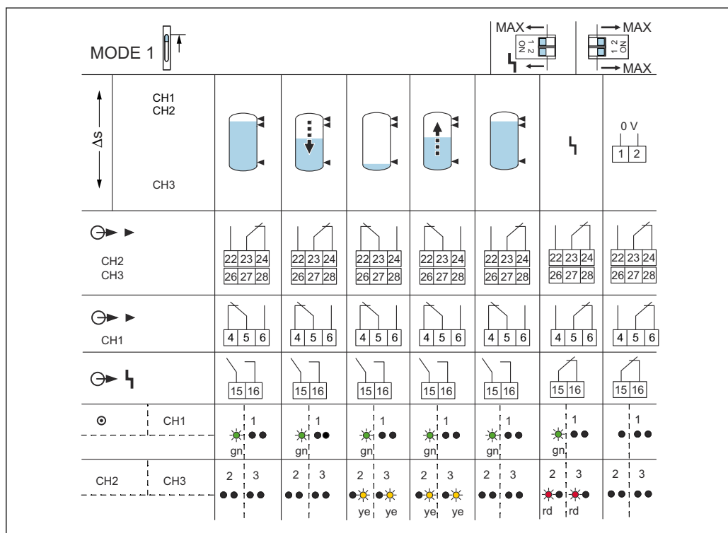
図 29 スイッチング動作および信号伝達
