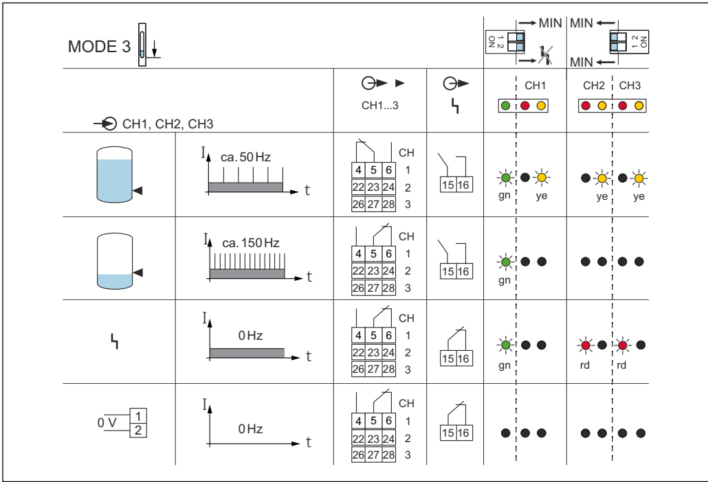
図 26 スイッチング動作および信号伝達
