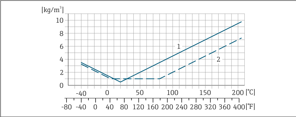
1 Étalonnage sur site de la masse volumique, exemple pour +20 °C (+68 °F) 2 Étalonnage spécial de la masse volumique
