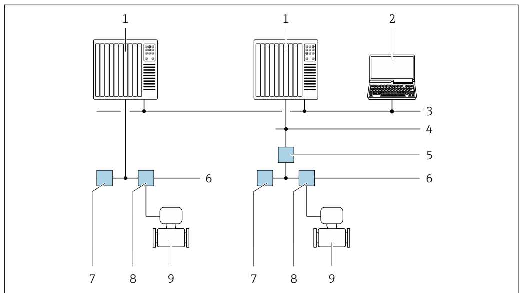
30 Possibilités de configuration à distance via réseau FOUNDATION Fieldbus
