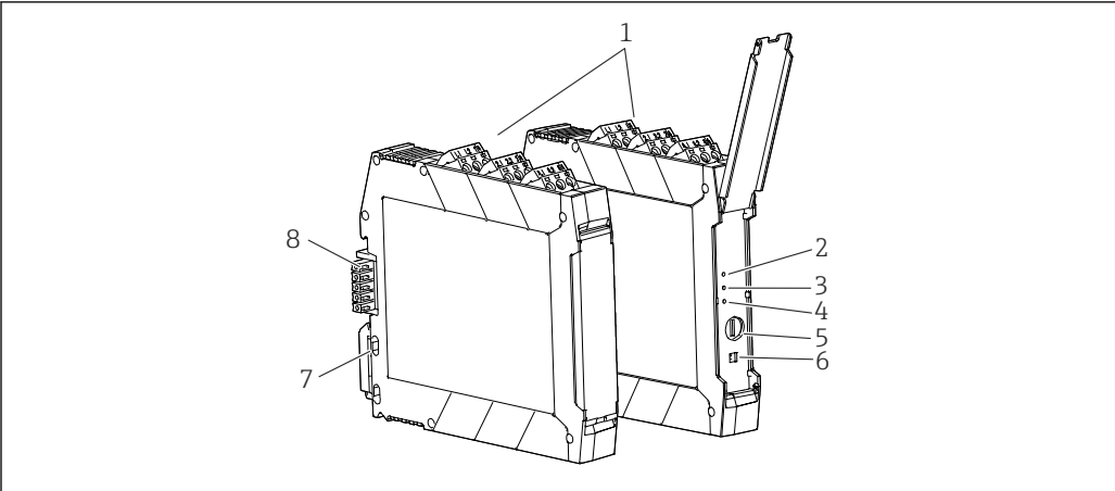
11 Display e elementos de operação
