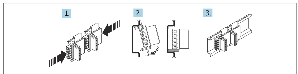
2 Instalação do conector de barramento de trilho DIN 17.5 mm (0.69 in)
