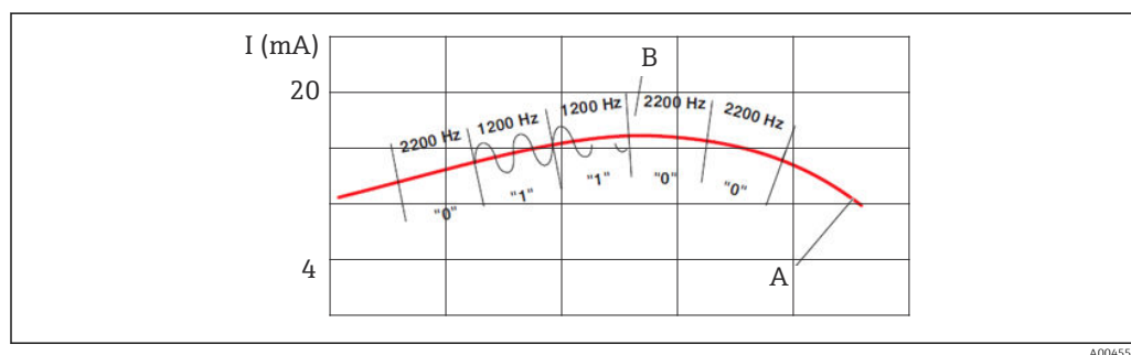
16 Sinal HART modulado
