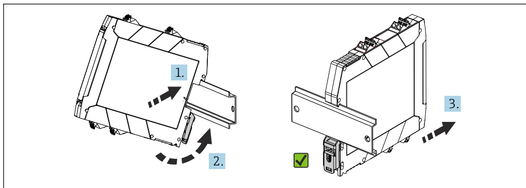
3 Instalação no trilho DIN
