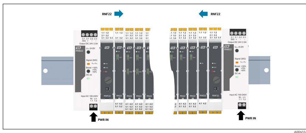
Fig. 15 Exemplo de alimentação através de dois módulos de alimentação RNF22
