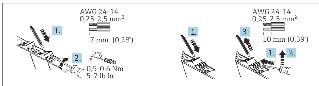
5 Conexão elétrica usando terminais de parafuso (esquerda) e terminais push-in (direita)
