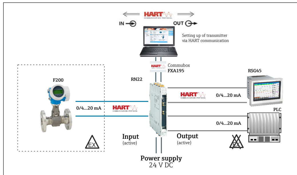
19 Medição de vazão em uma área classificada com um duplicador de sinal RN22
