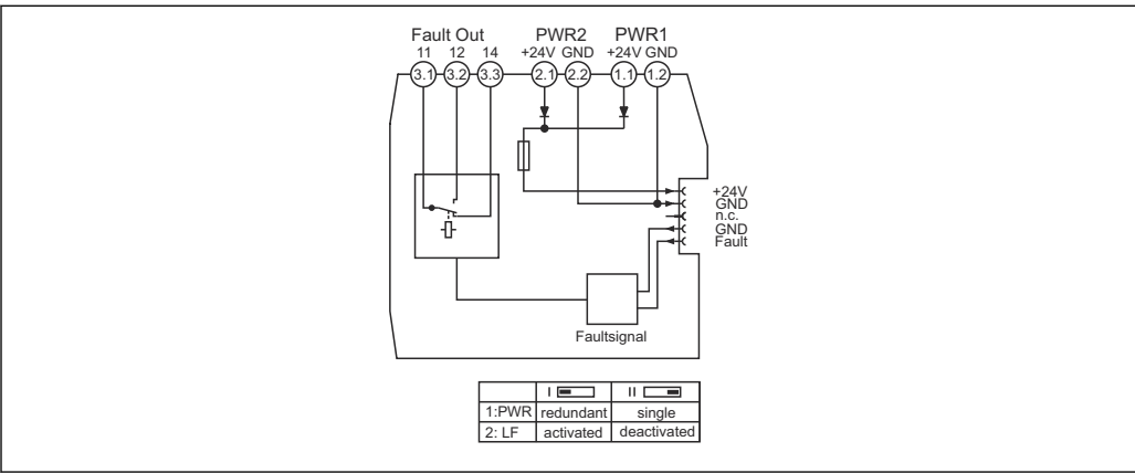
8 Esquema de ligação elétrica RNF22: módulo de alimentação e mensagem de erro
