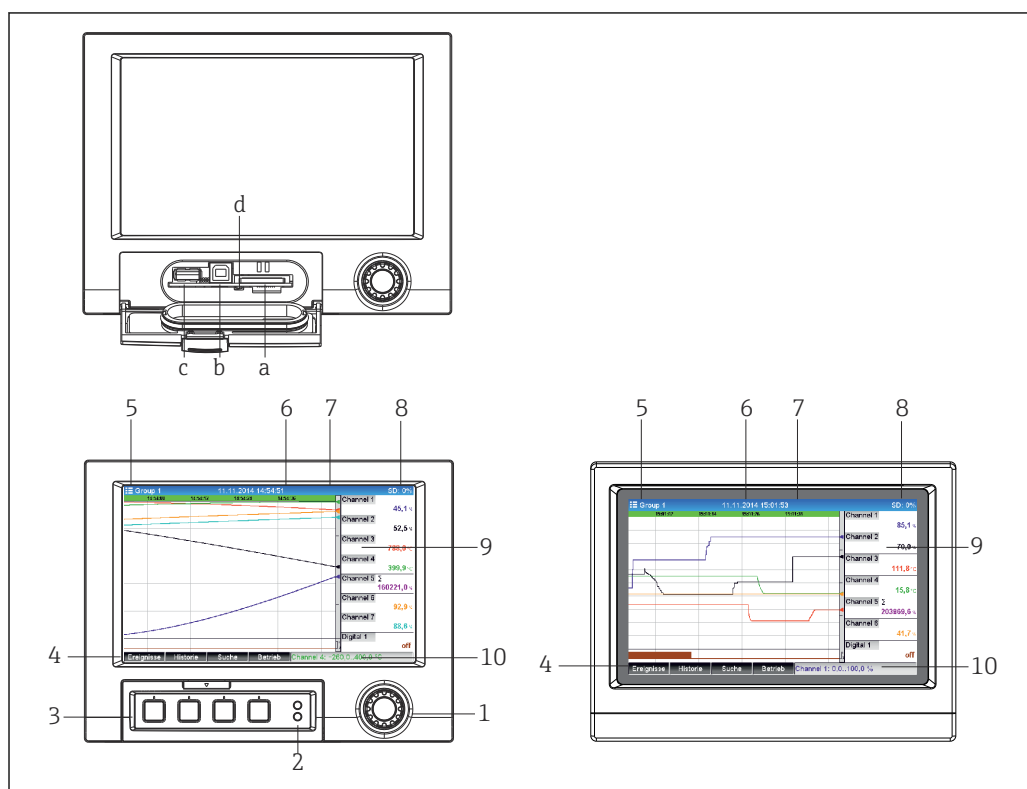
図 6 機器前面（左側：ナビゲータおよび前面インターフェイス付きバージョン、右側：ステンレス製の前面部およびタッチスクリーン付きバージョン）
