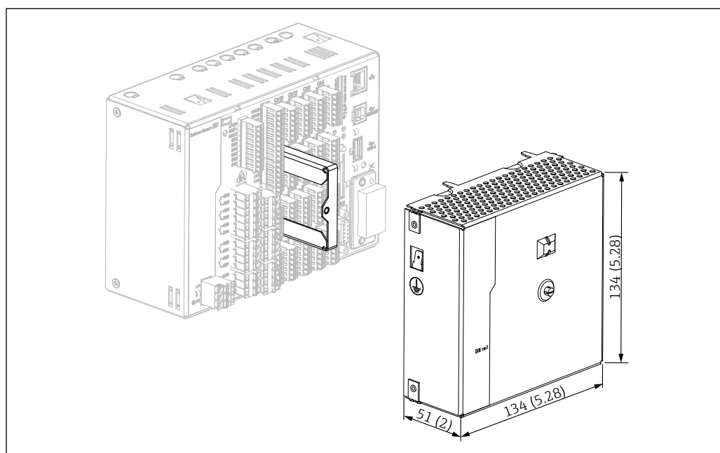
図 5 DIN レール型の端子カバーの寸法（単位：mm (in)）
