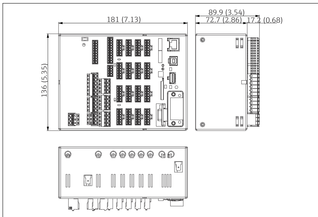
図 4 DIN レール型の寸法（単位：mm (in)）
