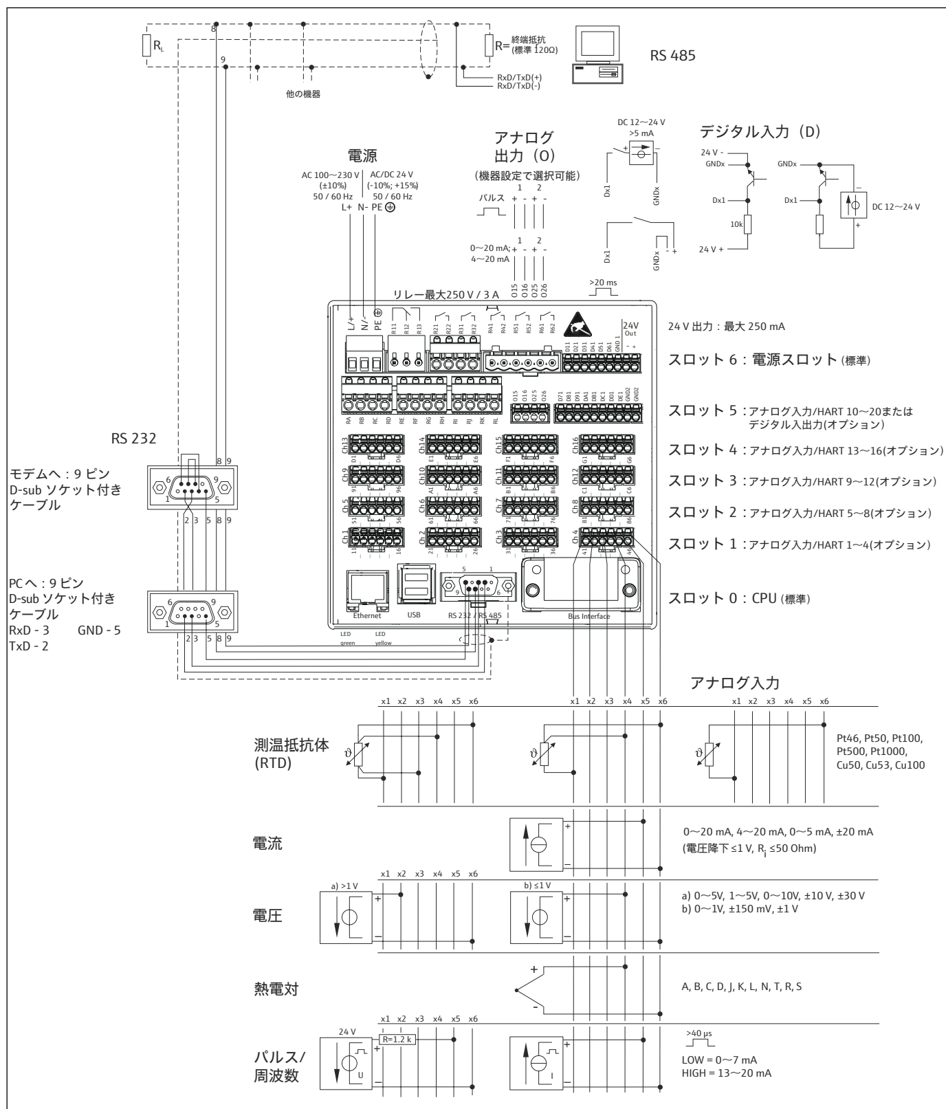
図 2 HART® 入力 (オプション) の接続例は、取扱説明書を参照してください。
