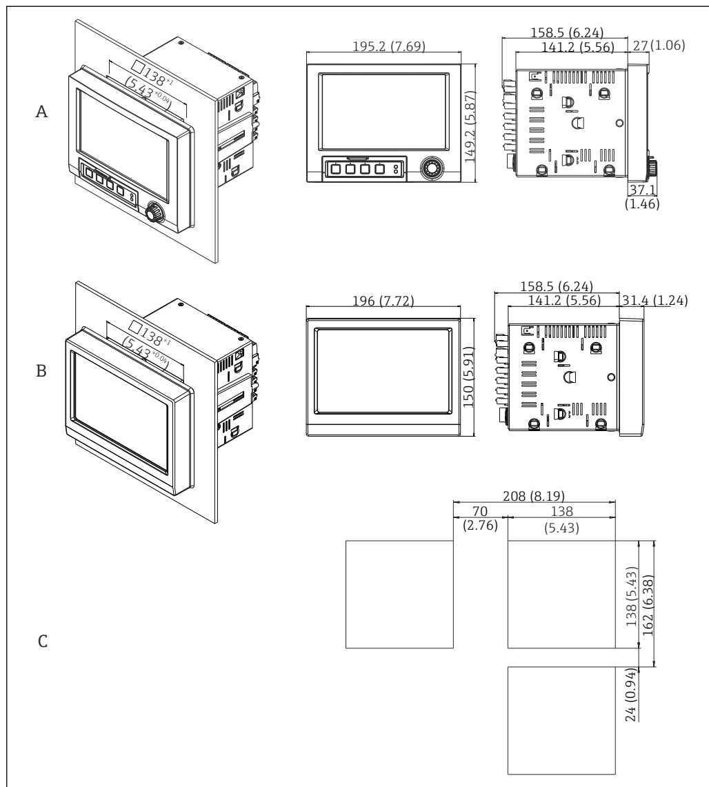
図 3 パネルの取付けおよび寸法 (単位: mm (in))
