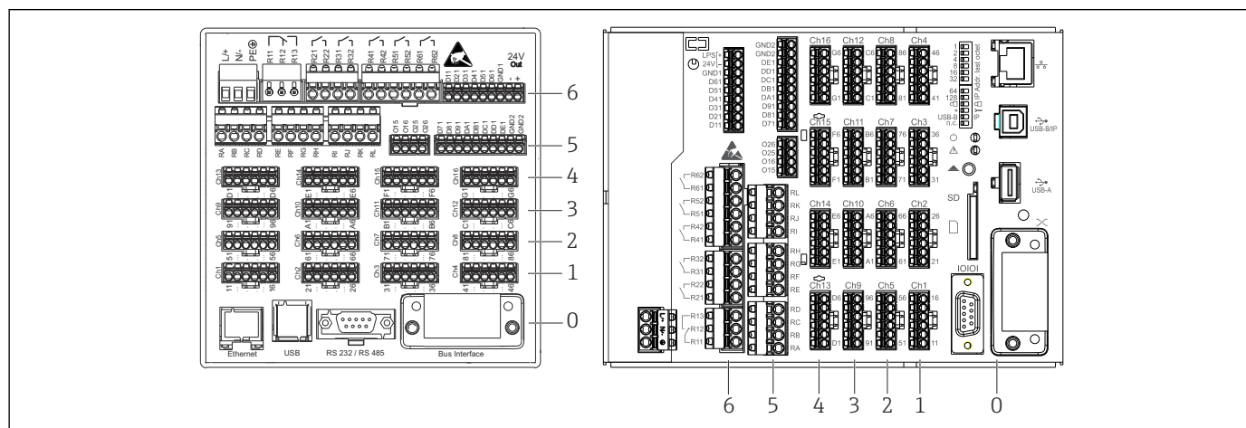
図 1 接続部：機器背面、パネル取付型（左）、DIN レール取付型（右）
